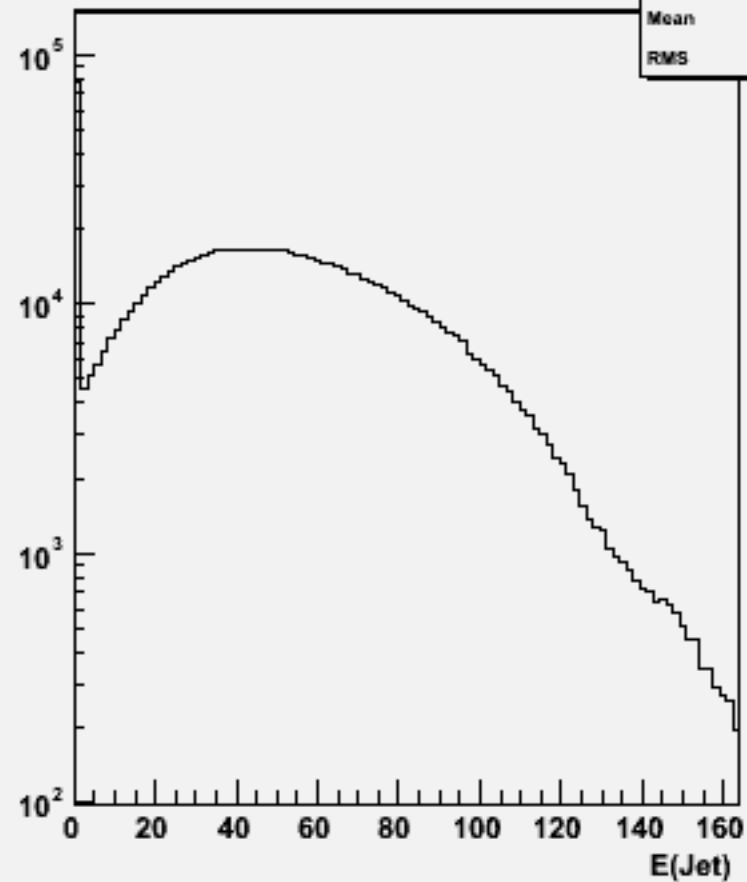
Jet energies(All jets)w100723 e1e1n2e2e3n3_o
