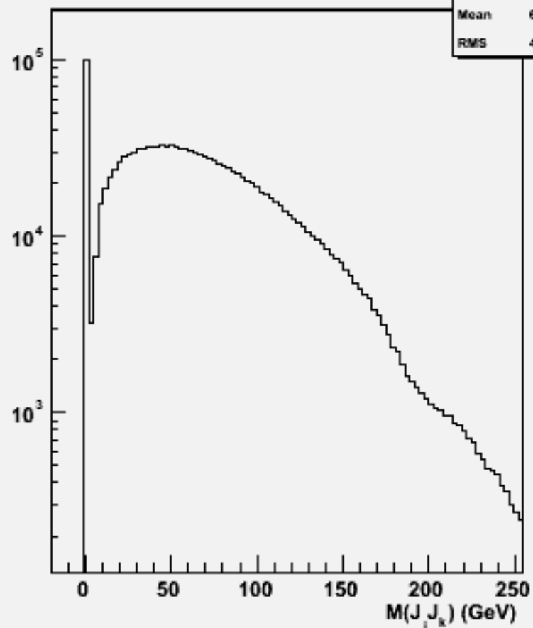
2jets mass(All comb)w100723 e1e1n2e2e3n3_o
