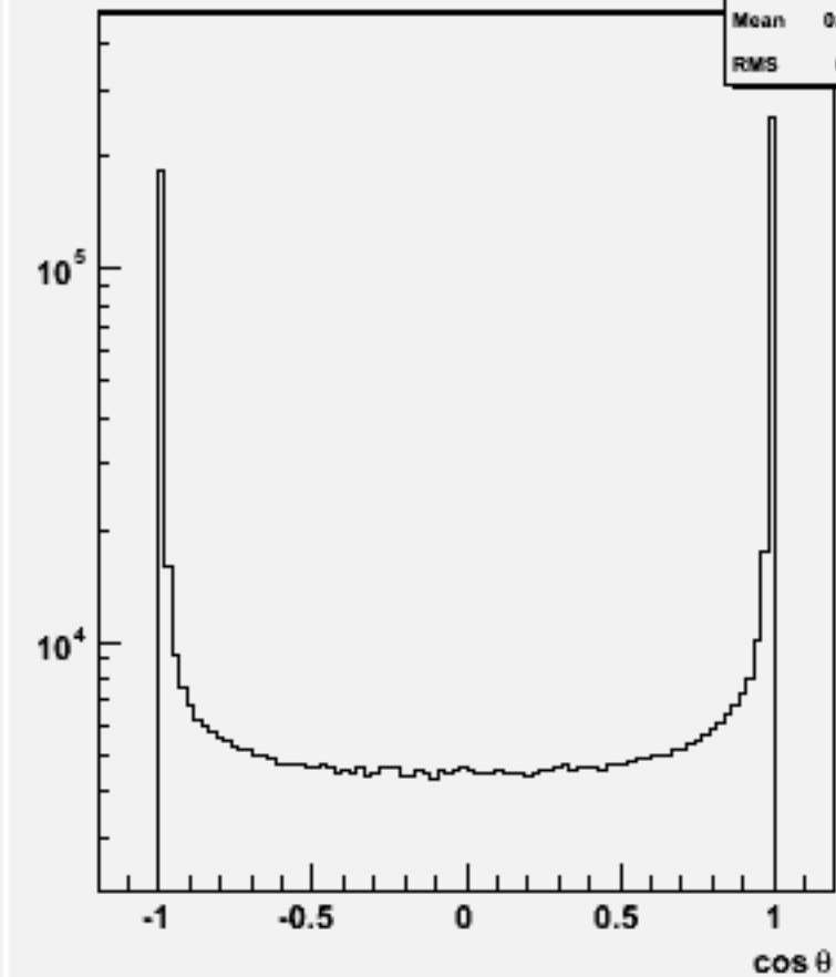
Jet cos \theta (All jets)w100723 e1e1n2e2e3n3_o
