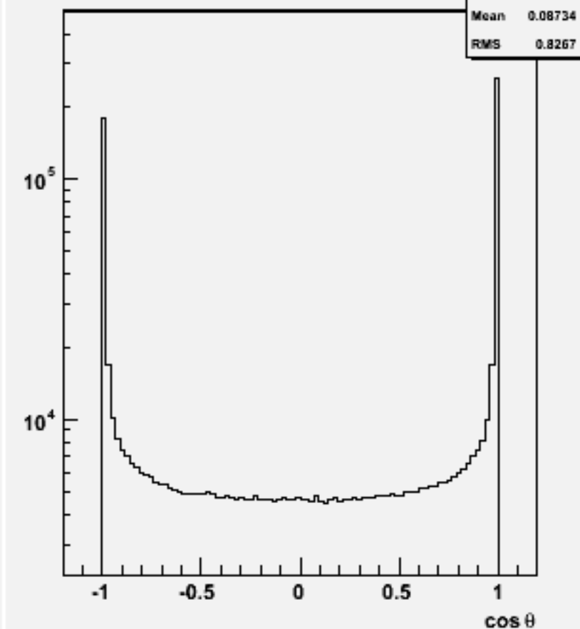
Jet cos theta (All jets)w100722 e1e1n2e2e2n2_o
