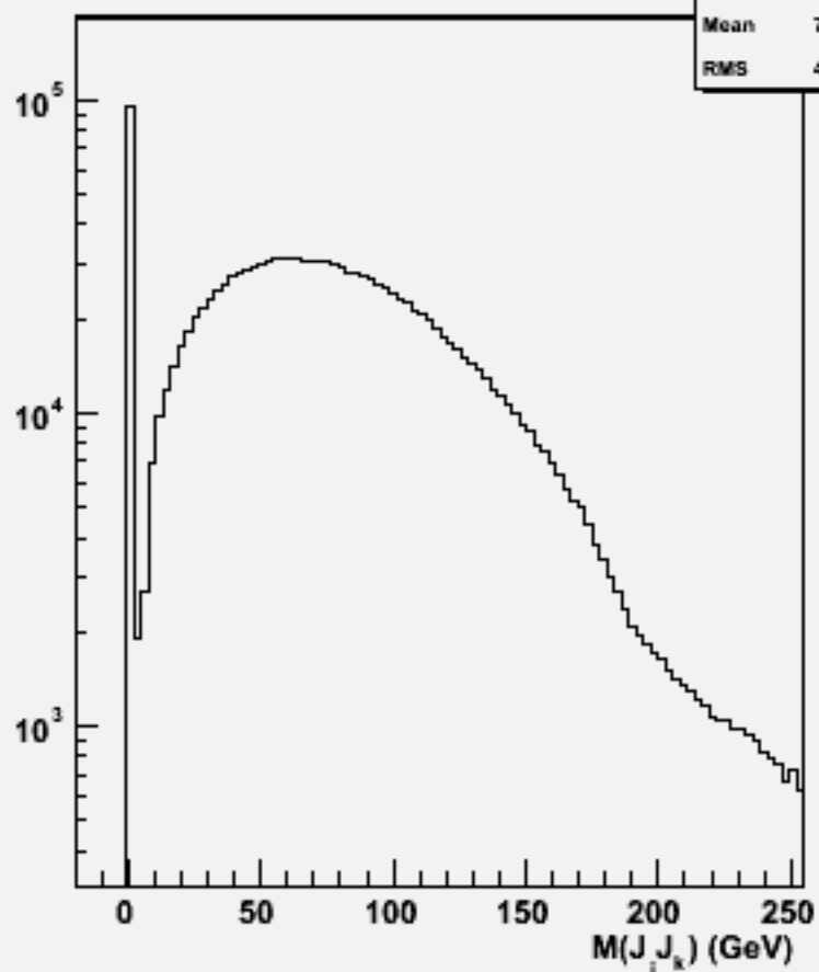
2jets mass(All comb)w100722 e1e1n2e2e2n2_o
