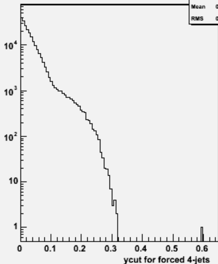
Ycut for 4-jets :w100722 e1e1n2e2e2n2_o
