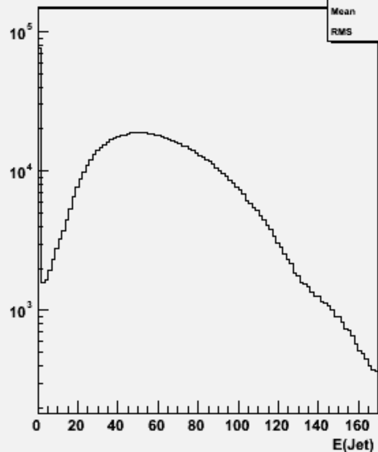
Jet energies(All jets)w100722 e1e1n2e2e2n2_o
