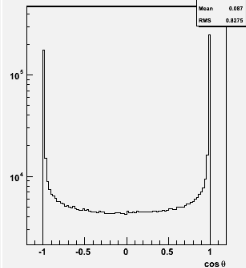
Jet cos theta (All jets)w100721 e1e1n2e2e2n2_o
