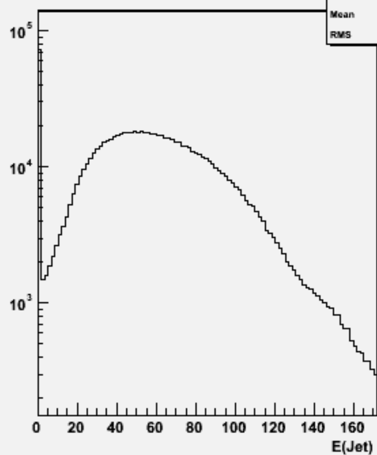
Jet energies(All jets)w100721 e1e1n2e2e2n2_o
