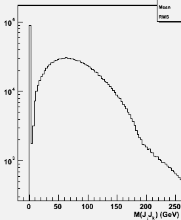
2jets mass(All comb)w100721 e1e1n2e2e2n2_o
