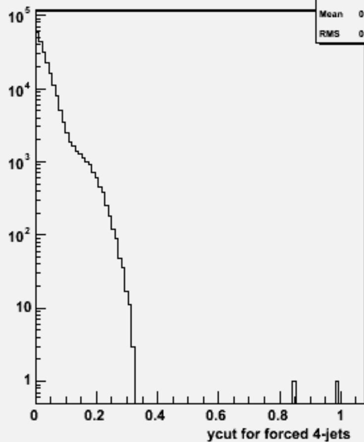
Ycut for 4-jets :w100721 e1e1n2e2e2n2_o
