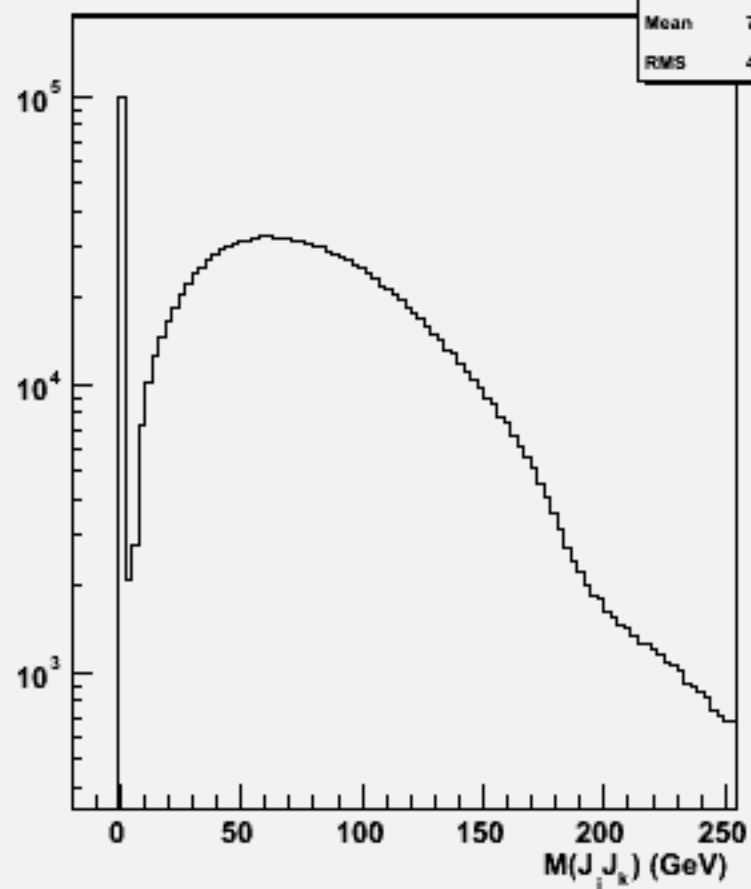
2jets mass(All comb)w100720 e1e1n2e2e2n2_o
