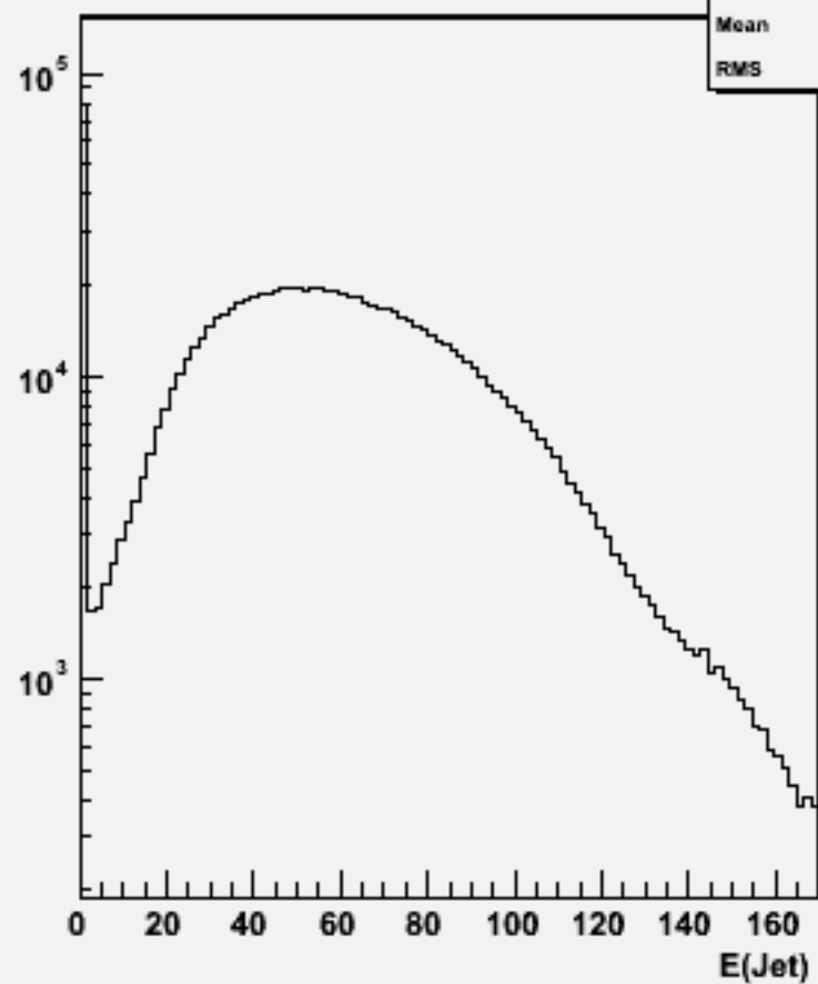
Jet energies(All jets)w100720 e1e1n2e2e2n2_o
