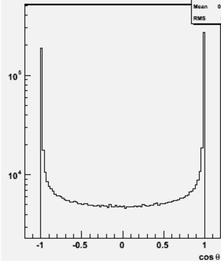
Jet cos \theta (All jets)w100720 e1e1n2e2e2n2_o
