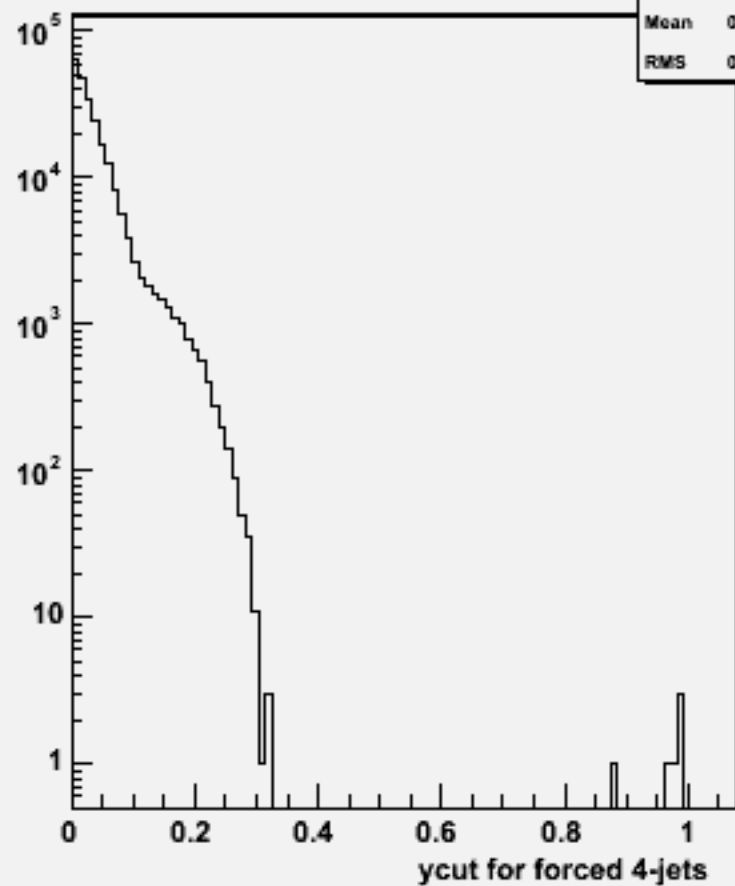
Ycut for 4-jets :w100720 e1e1n2e2e2n2_o
