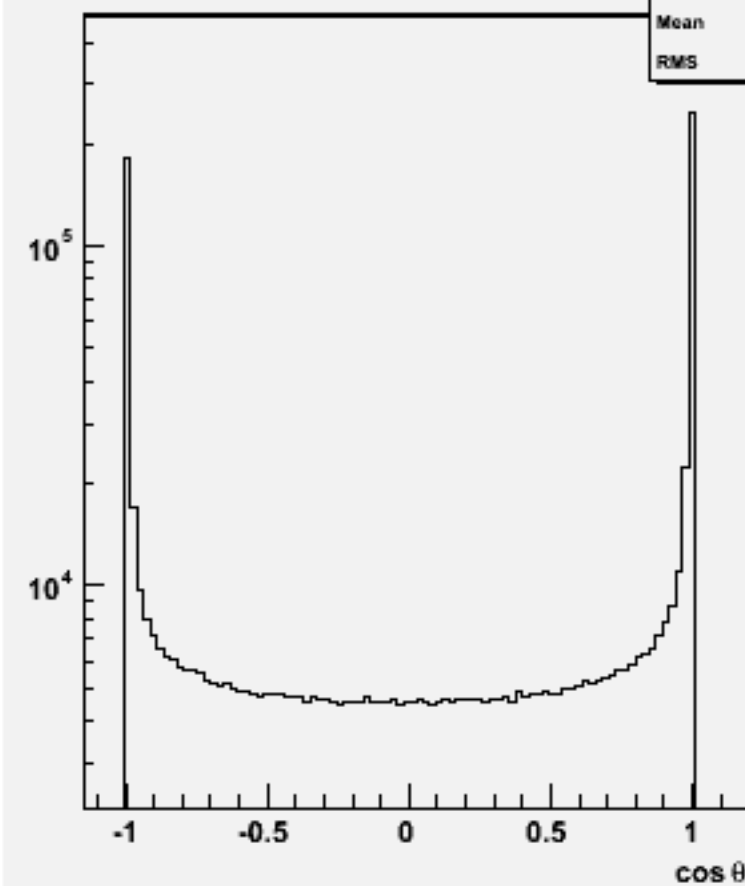
Jet cos \theta (All jets)w100719 e1e1n2e2e2n2_o
