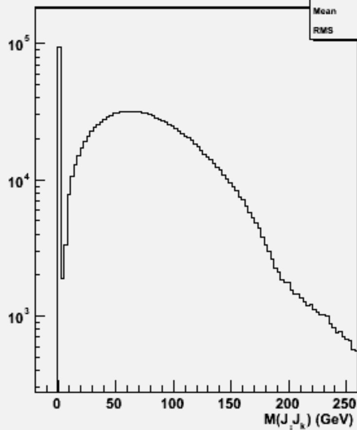
2jets mass(All comb)w100719 e1e1n2e2e2n2_o
