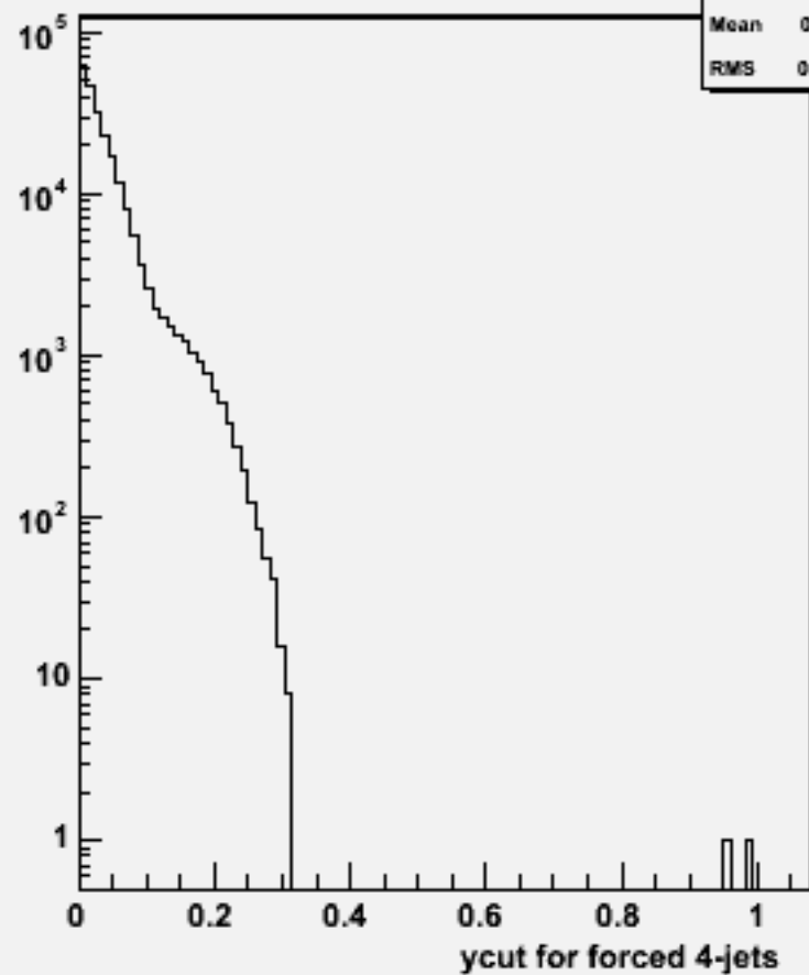
Ycut for 4-jets :w100719 e1e1n2e2e2n2_o
