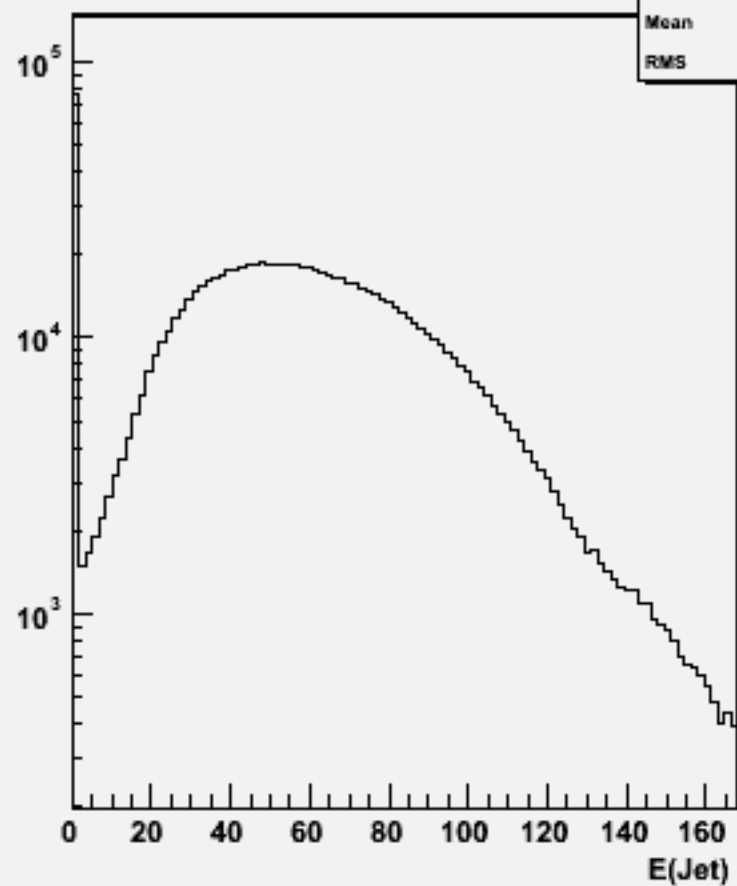
Jet energies(All jets)w100719 e1e1n2e2e2n2_o
