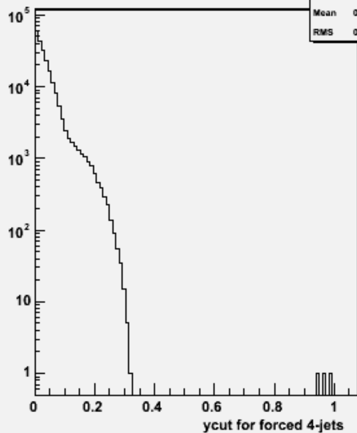
Ycut for 4-jets :w100718 e1e1n2e2e1n1_o
