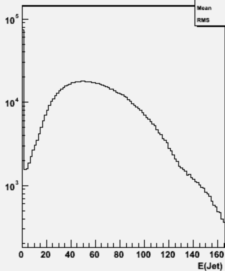
Jet energies(All jets)w100718 e1e1n2e2e1n1_o
