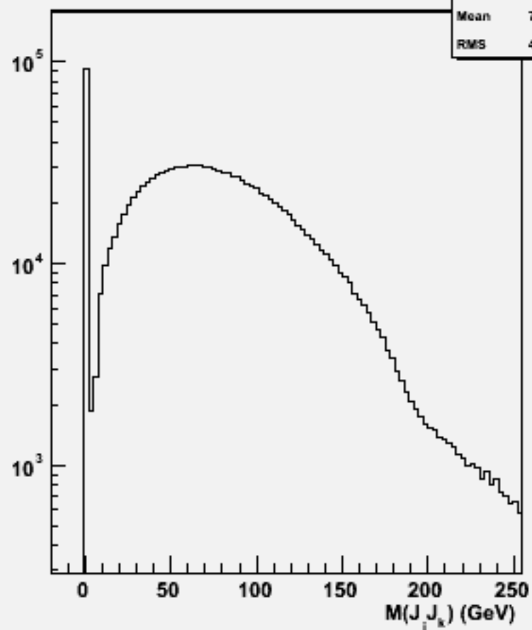
2jets mass(All comb)w100718 e1e1n2e2e1n1_o
