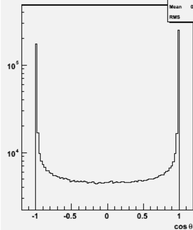
Jet cos \theta (All jets)w100718 e1e1n2e2e1n1_o
