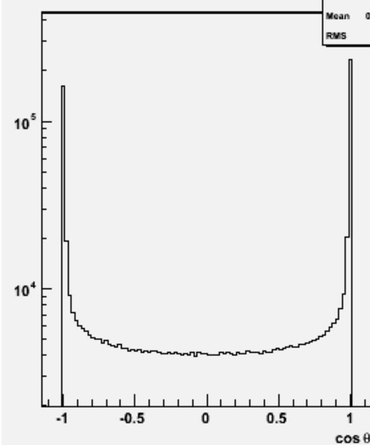
Jet cos \theta (All jets)w100717 e1e1n2e2e1n1_o
