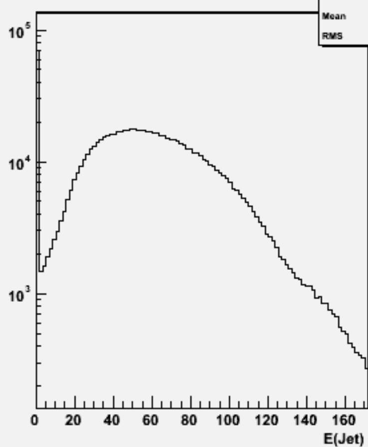
Jet energies(All jets)w100717 e1e1n2e2e1n1_o
