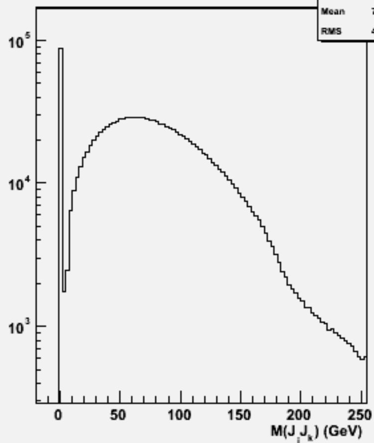
2jets mass(All comb)w100717 e1e1n2e2e1n1_o
