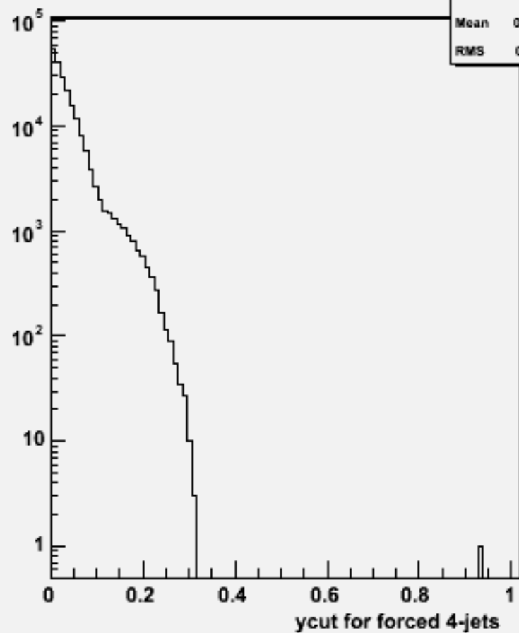
Ycut for 4-jets :w100717 e1e1n2e2e1n1_o
