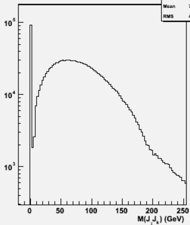
2jets mass(All comb)w100715 e1e1n2e2e1n1_o
