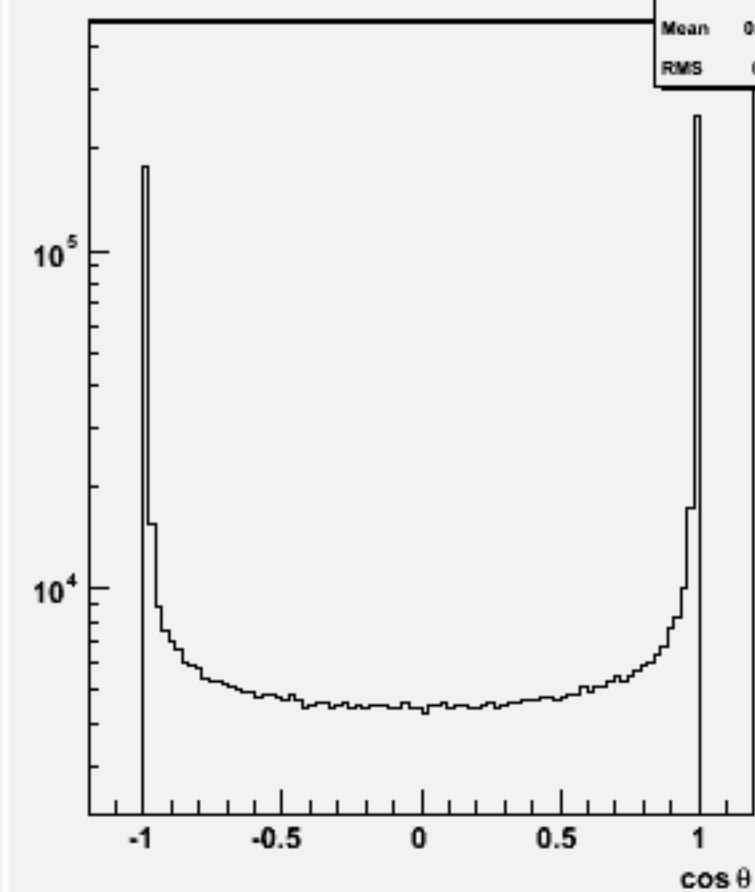
Jet cos \theta (All jets)w100715 e1e1n2e2e1n1_o
