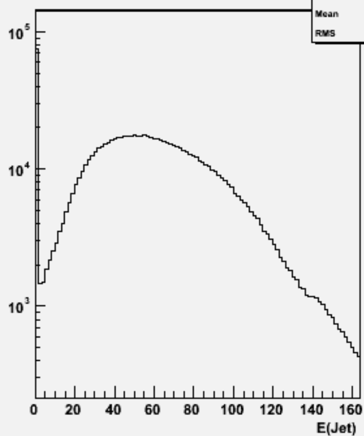
Jet energies(All jets)w100715 e1e1n2e2e1n1_o
