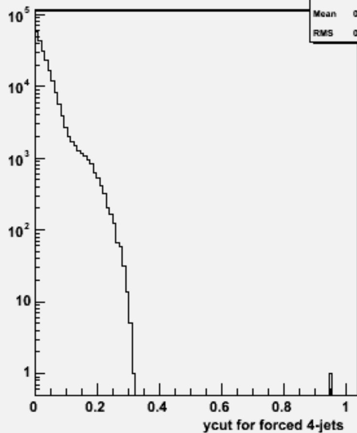
Ycut for 4-jets :w100715 e1e1n2e2e1n1_o
