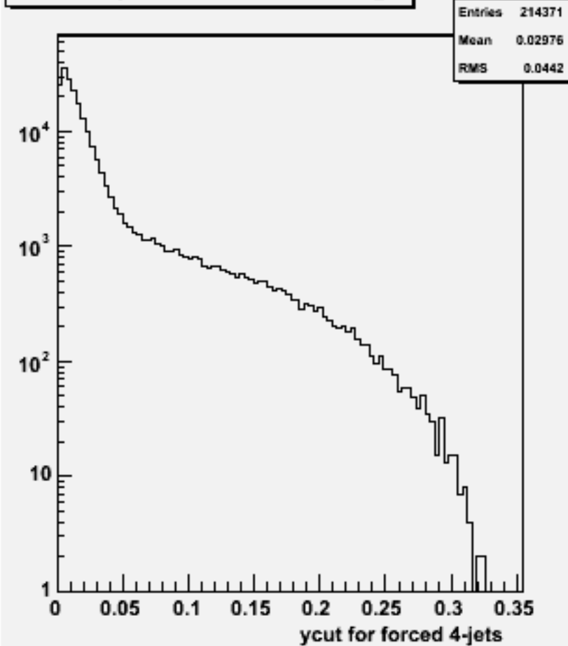
Ycut for 4-jets :w100714 e1e1n1e1sc_o
