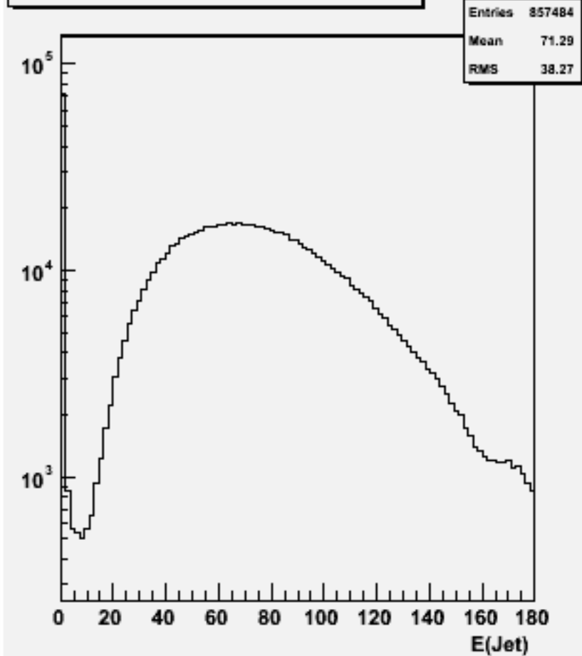
Jet energies(All jets)w100714 e1e1n1e1sc_o
