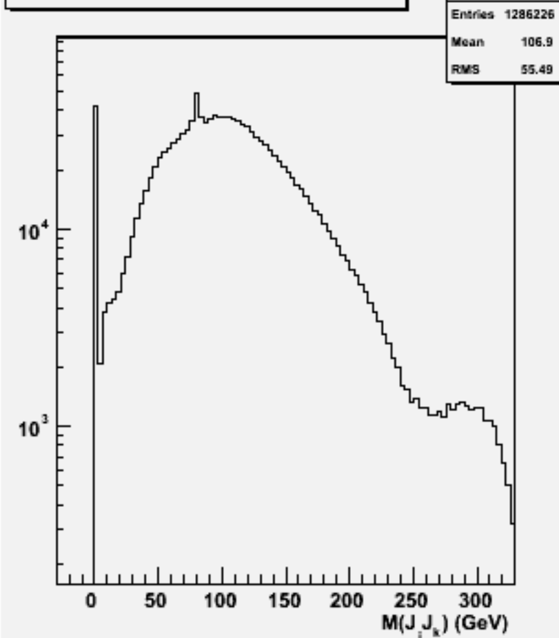
2jets mass(All comb)w100714 e1e1n1e1sc_o
