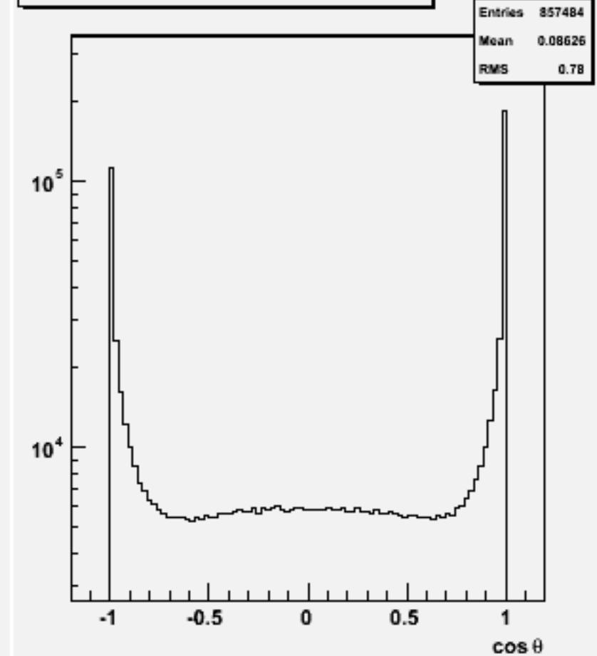
Jet cos \theta (All jets)w100714 e1e1n1e1sc_o
