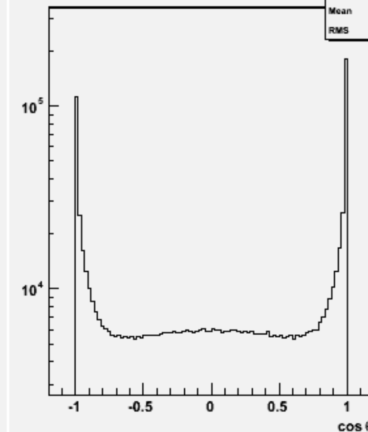
Jet cos \theta (All jets)w100712 e1e1n1e1sc_o
