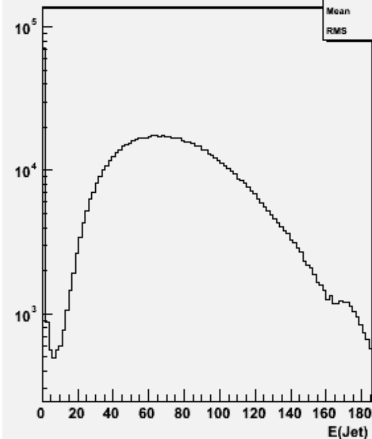
Jet energies(All jets)w100712 e1e1n1e1sc_o
