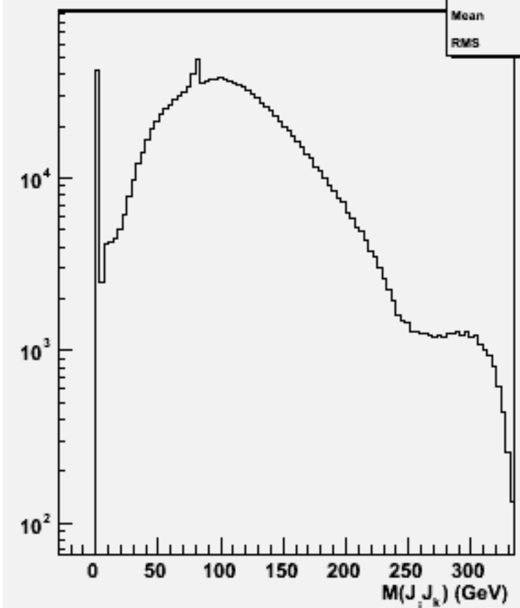
2jets mass(All comb)w100712 e1e1n1e1sc_o
