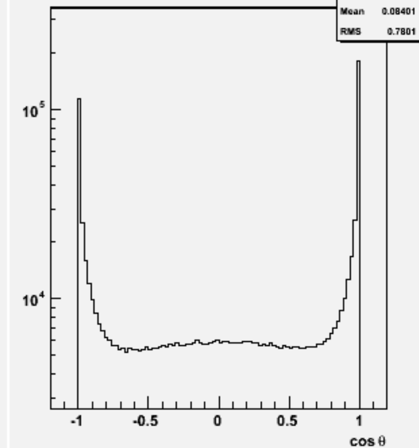
Jet cos \theta (All jets)w100711 e1e1n1e1sc_o
