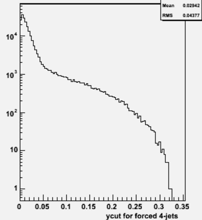
Ycut for 4-jets :w100711 e1e1n1e1sc_o
