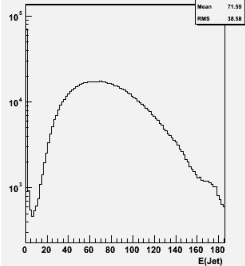
Jet energies(All jets)w100711 e1e1n1e1sc_o
