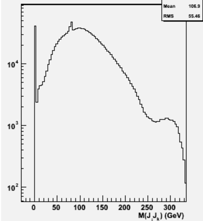
2jets mass(All comb)w100711 e1e1n1e1sc_o
