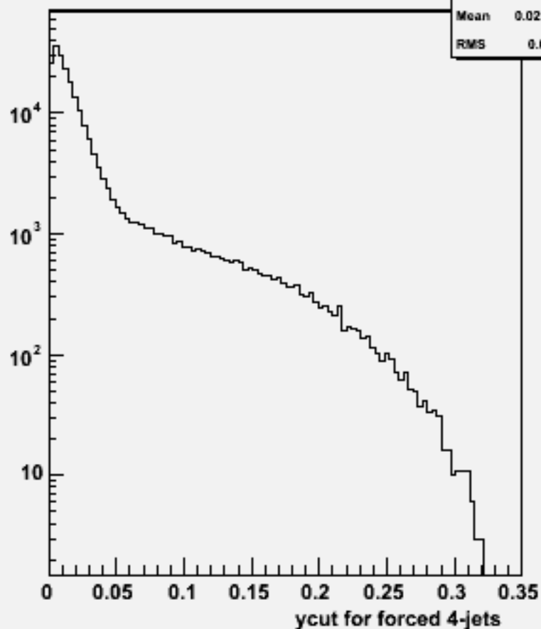
Ycut for 4-jets :w100710 e1e1n1e1du_o
