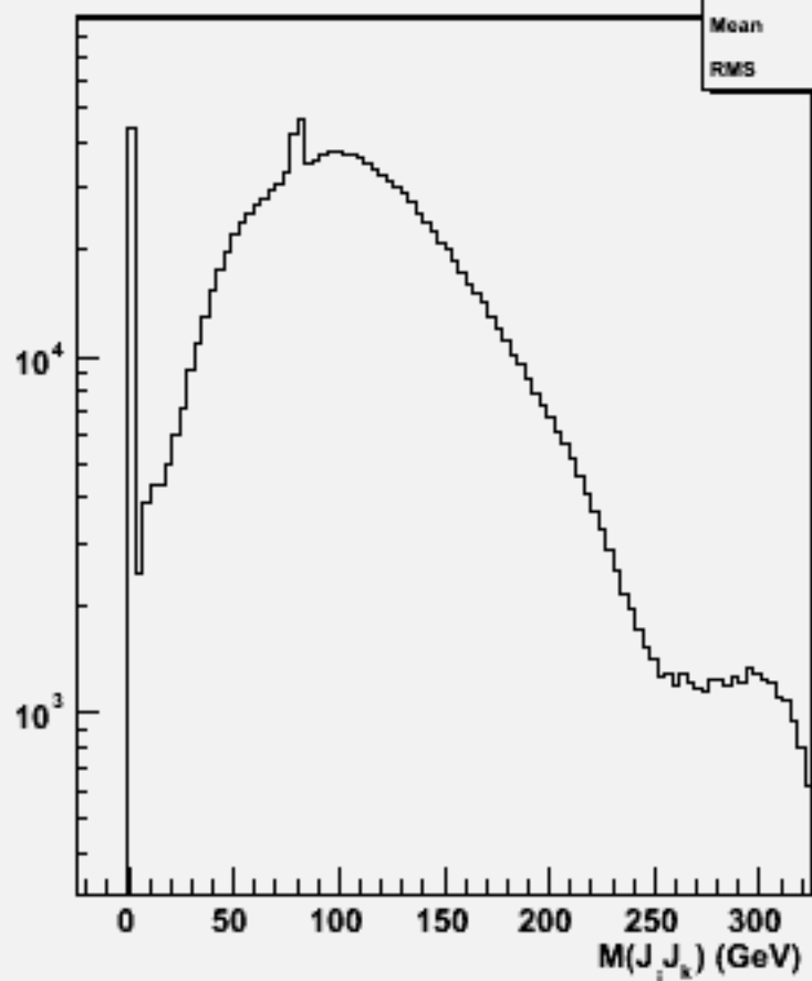
2jets mass(All comb)w100710 e1e1n1e1du_o
