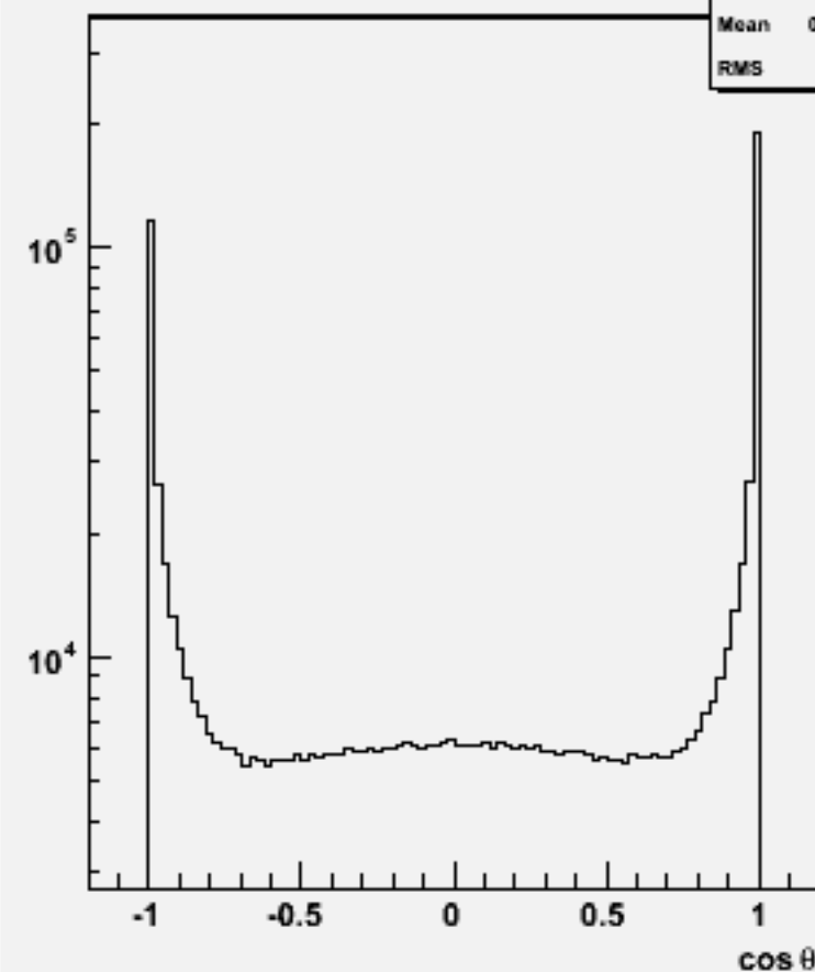
Jet cos \theta (All jets)w100710 e1e1n1e1du_o
