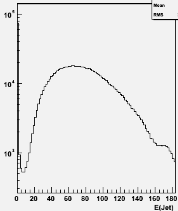
Jet energies(All jets)w100710 e1e1n1e1du_o
