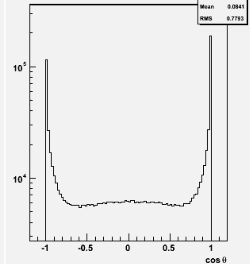
Jet cos \theta (All jets)w100708 e1e1n1e1du_o
