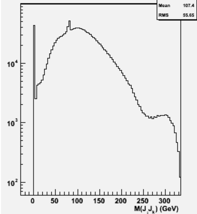
2jets mass(All comb)w100708 e1e1n1e1du_o
