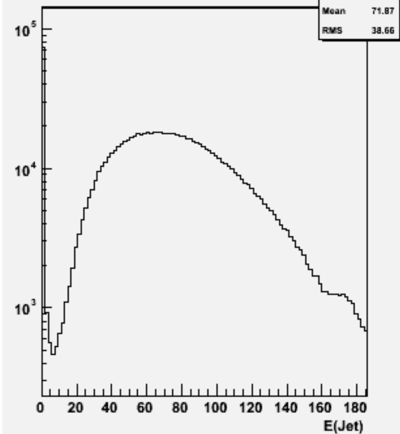
Jet energies(All jets)w100708 e1e1n1e1du_o
