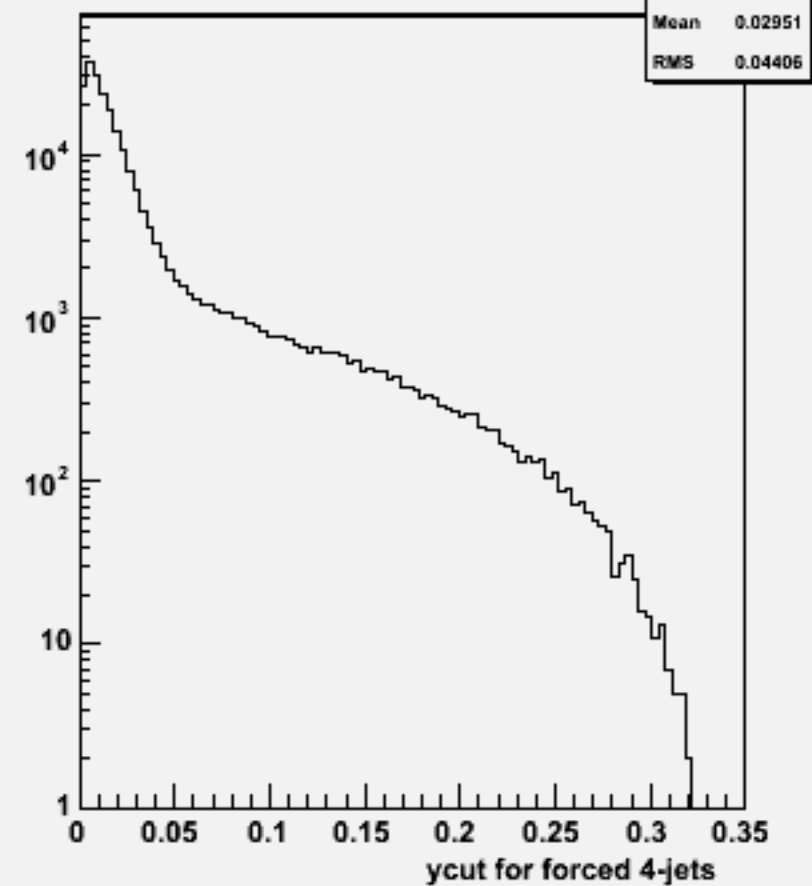
Ycut for 4-jets :w100708 e1e1n1e1du_o
