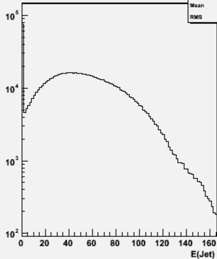
Jet energies(All jets)w100706 e1e1n1e1e3n3_o
