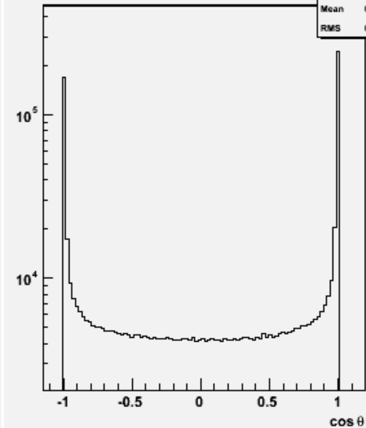
Jet cos \theta (All jets)w100706 e1e1n1e1e3n3_o
