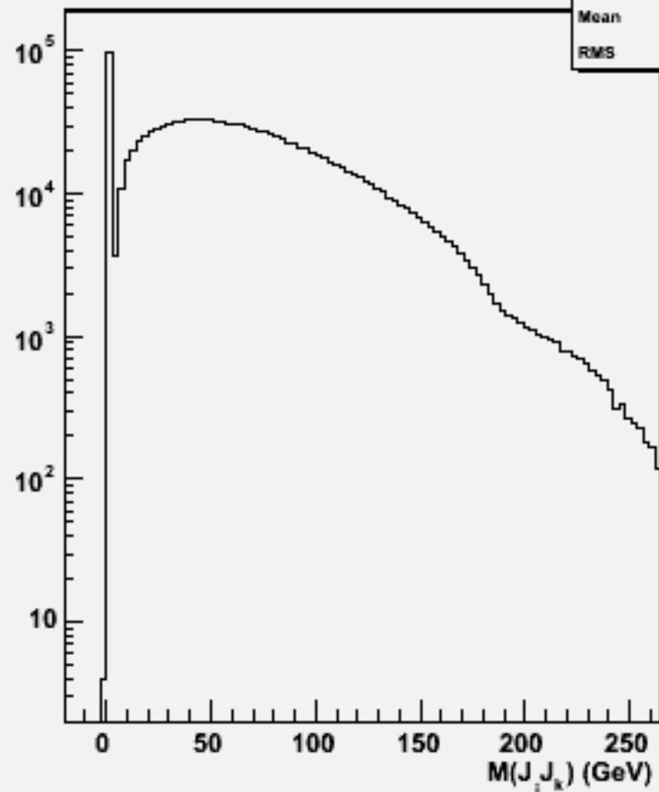
2jets mass(All comb)w100706 e1e1n1e1e3n3_o
