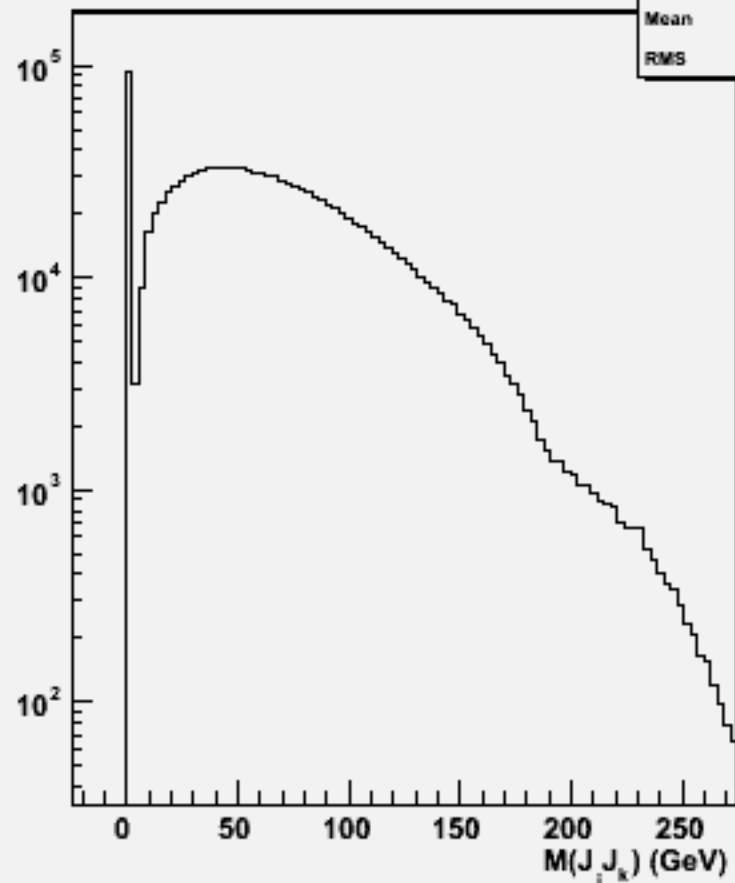
2jets mass(All comb)w100705 e1e1n1e1e3n3_o
