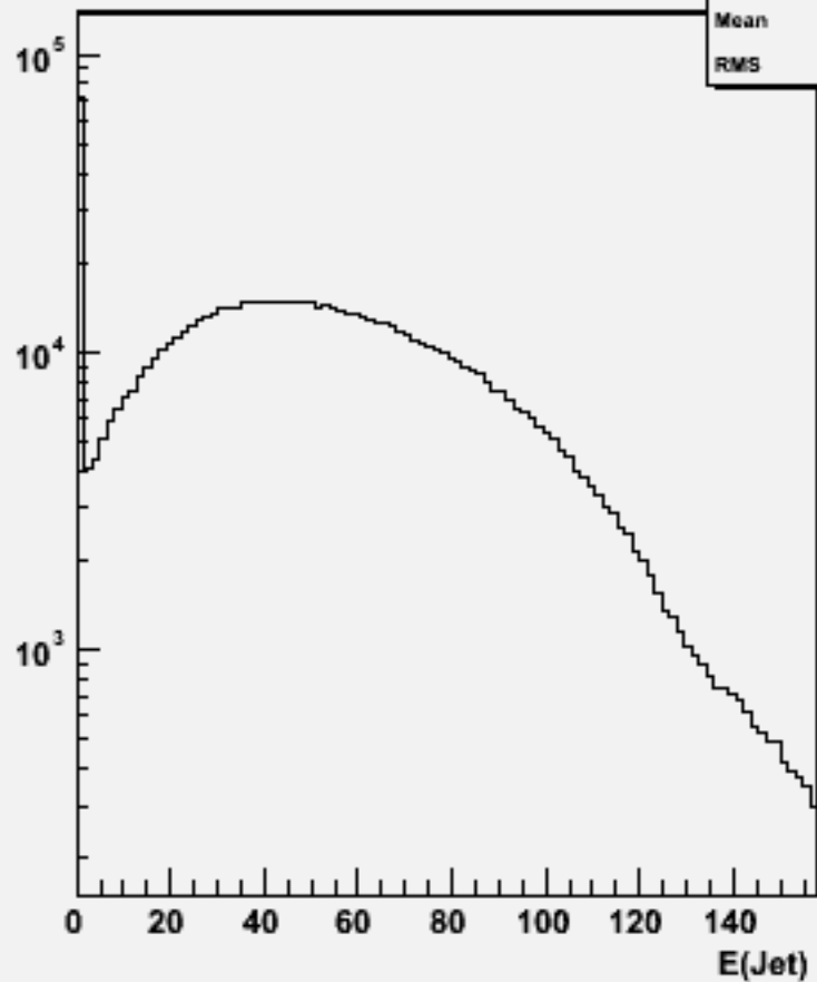
Jet energies(All jets)w100705 e1e1n1e1e3n3_o
