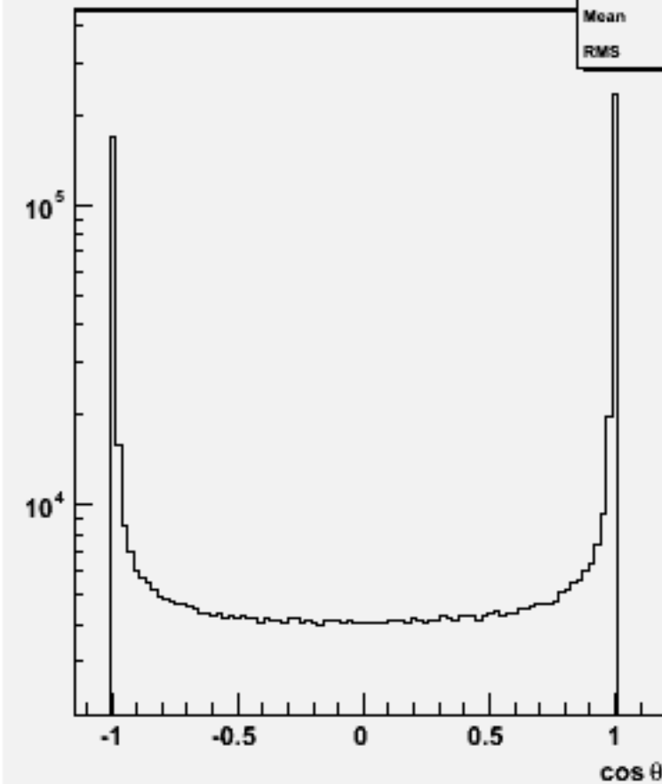
Jet cos \theta (All jets)w100705 e1e1n1e1e3n3_o
