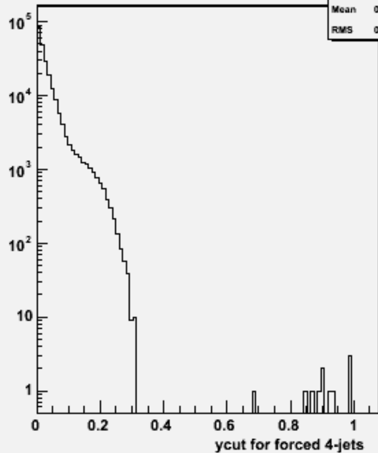
Ycut for 4-jets :w100704 e1e1n1e1e3n3_o
