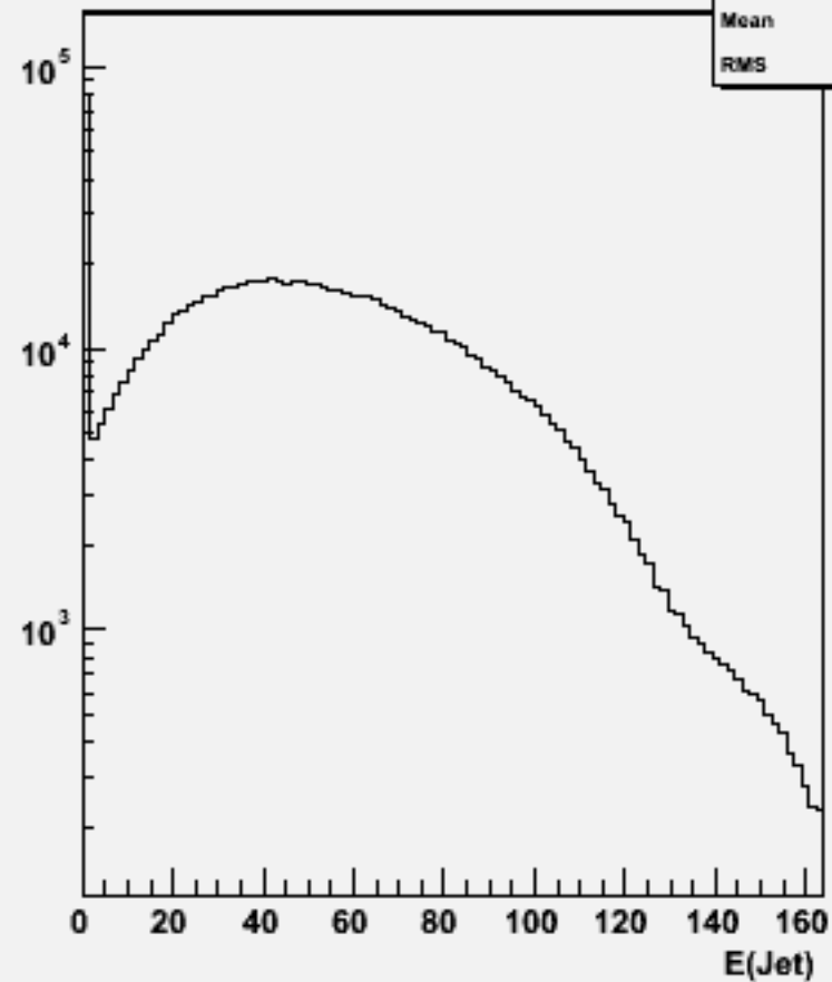
Jet energies(All jets)w100704 e1e1n1e1e3n3_o
