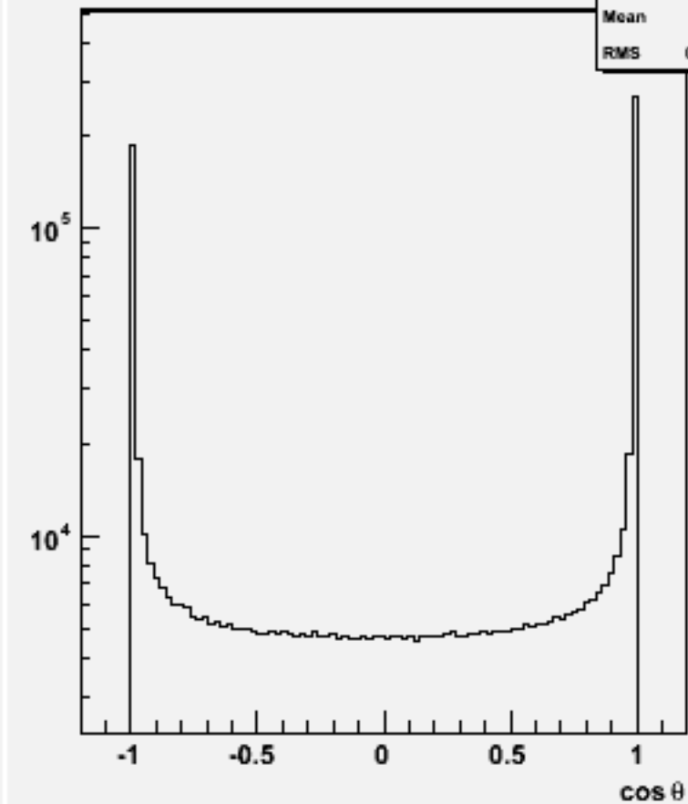
Jet cos \theta (All jets)w100704 e1e1n1e1e3n3_o
