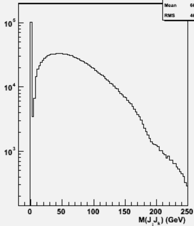
2jets mass(All comb)w100704 e1e1n1e1e3n3_o
