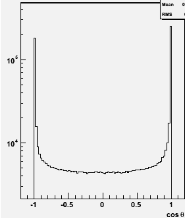
Jet cos \theta (All jets)w100703 e1e1n1e1e3n3_o
