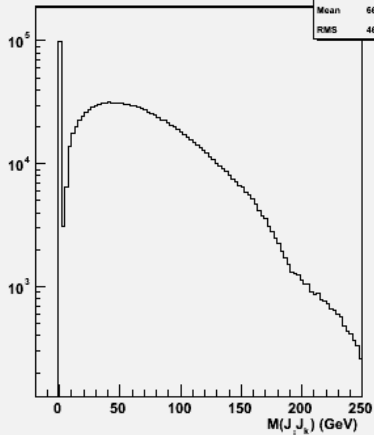
2jets mass(All comb)w100703 e1e1n1e1e3n3_o
