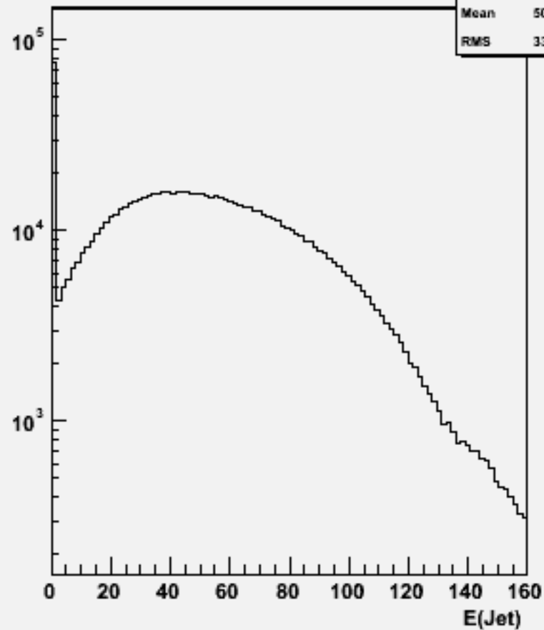
Jet energies(All jets)w100703 e1e1n1e1e3n3_o
