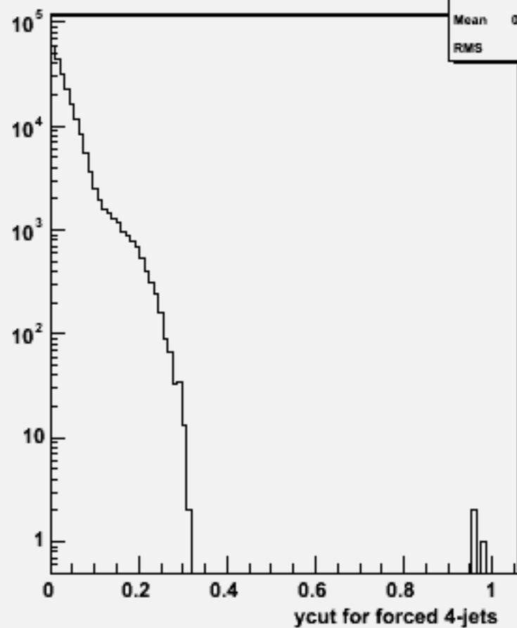
Ycut for 4-jets :w100702 e1e1n1e1e2n2_o
