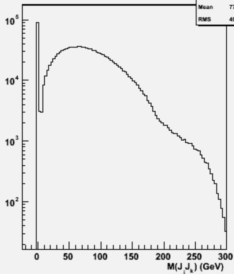
2jets mass(All comb)w100702 e1e1n1e1e2n2_o
