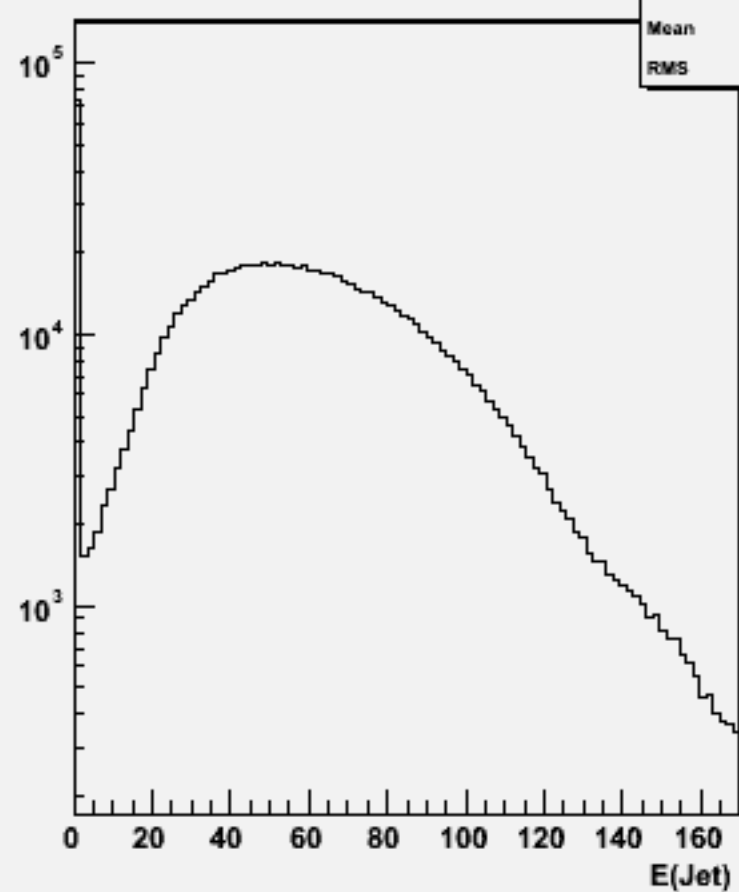
Jet energies(All jets)w100702 e1e1n1e1e2n2_o
