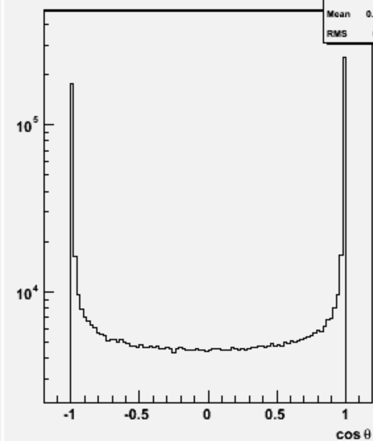
Jet cos \theta (All jets)w100702 e1e1n1e1e2n2_o
