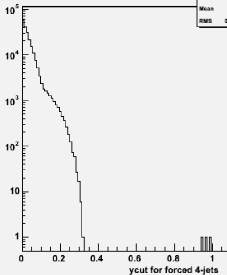
Ycut for 4-jets :w100701 e1e1n1e1e2n2_o
