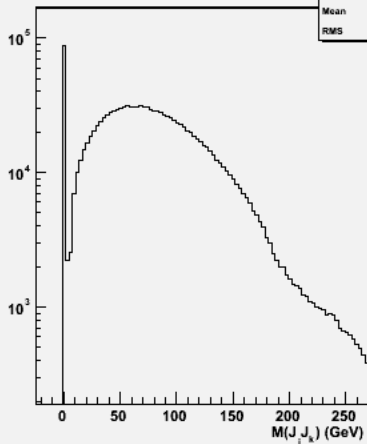
2jets mass(All comb)w100701 e1e1n1e1e2n2_o
