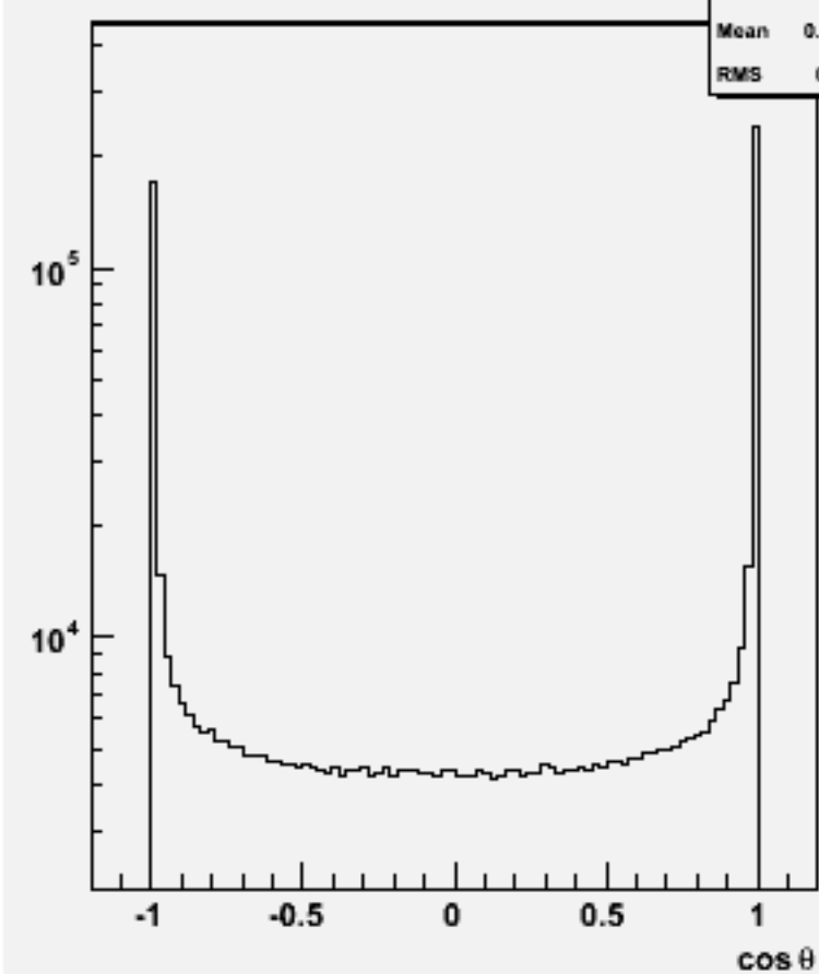
Jet cos \theta (All jets)w100701 e1e1n1e1e2n2_o
