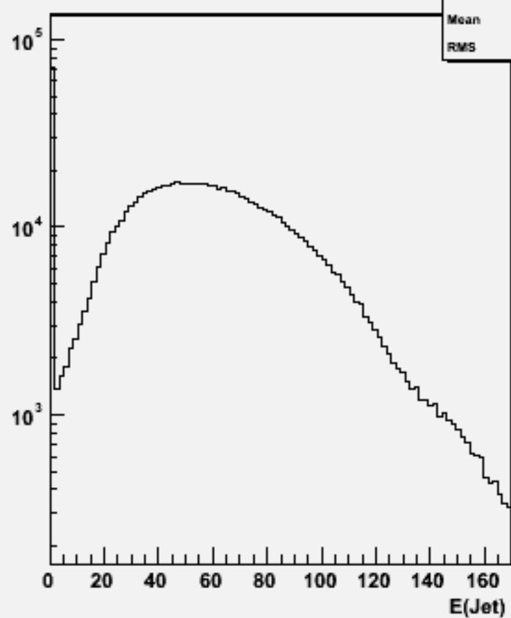
Jet energies(All jets)w100701 e1e1n1e1e2n2_o
