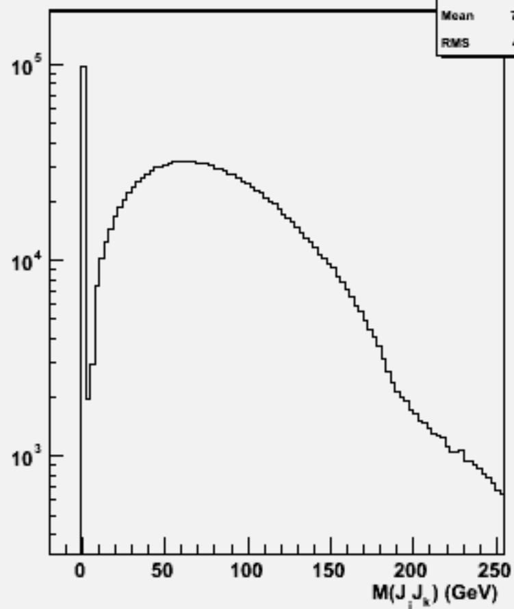
2jets mass(All comb)w100700 e1e1n1e1e2n2_o
