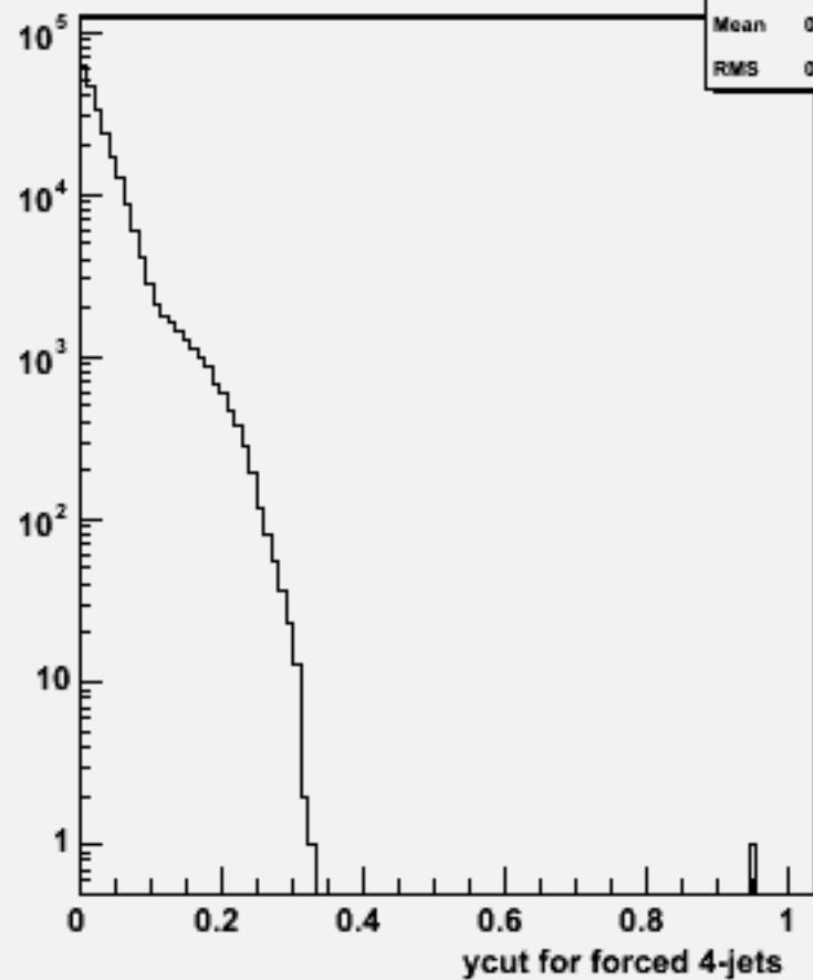
Ycut for 4-jets :w100700 e1e1n1e1e2n2_o
