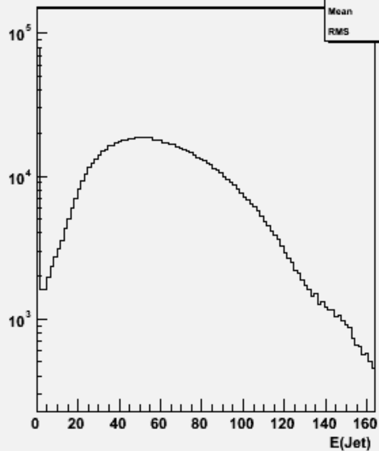
Jet energies(All jets)w100700 e1e1n1e1e2n2_o
