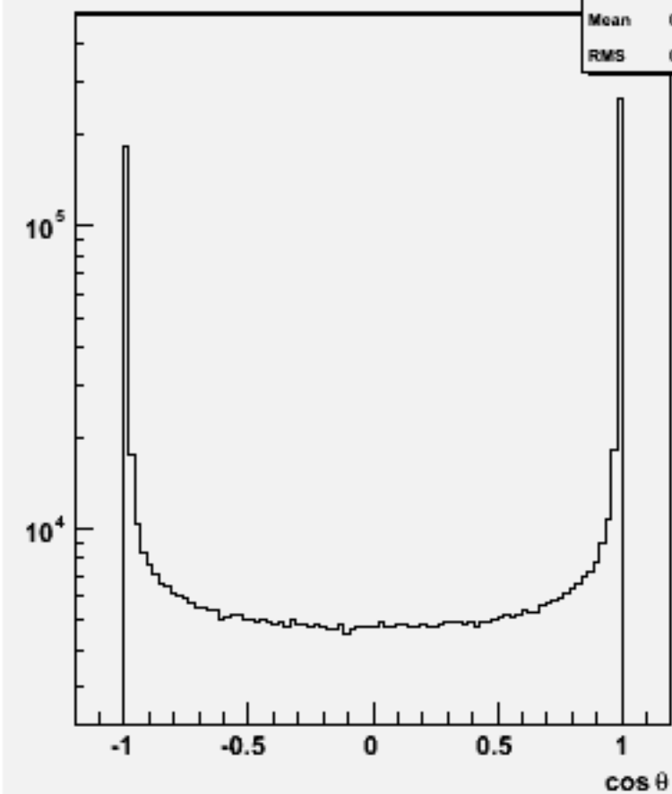
Jet cos \theta (All jets)w100700 e1e1n1e1e2n2_o
