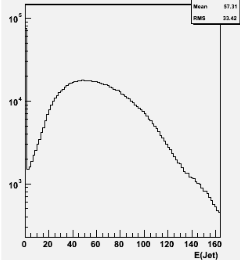
Jet energies(All jets)w100699 e1e1n1e1e2n2_o
