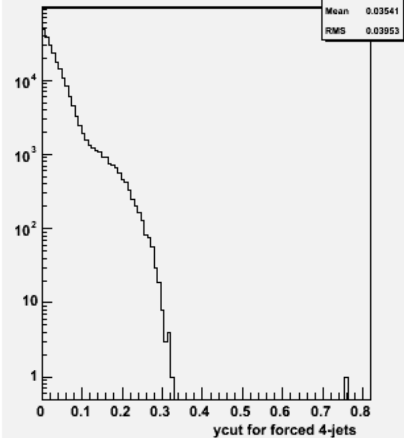
Ycut for 4-jets :w100699 e1e1n1e1e2n2_o
