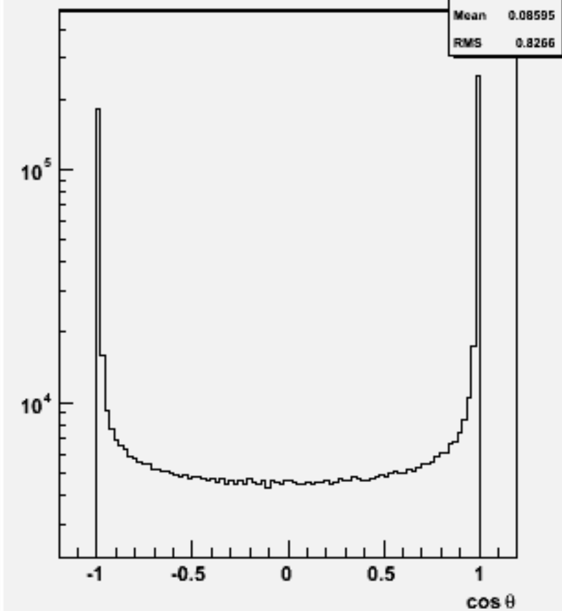
Jet cos \theta (All jets)w100699 e1e1n1e1e2n2_o
