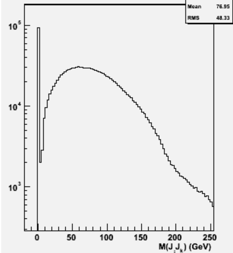
2jets mass(All comb)w100699 e1e1n1e1e2n2_o
