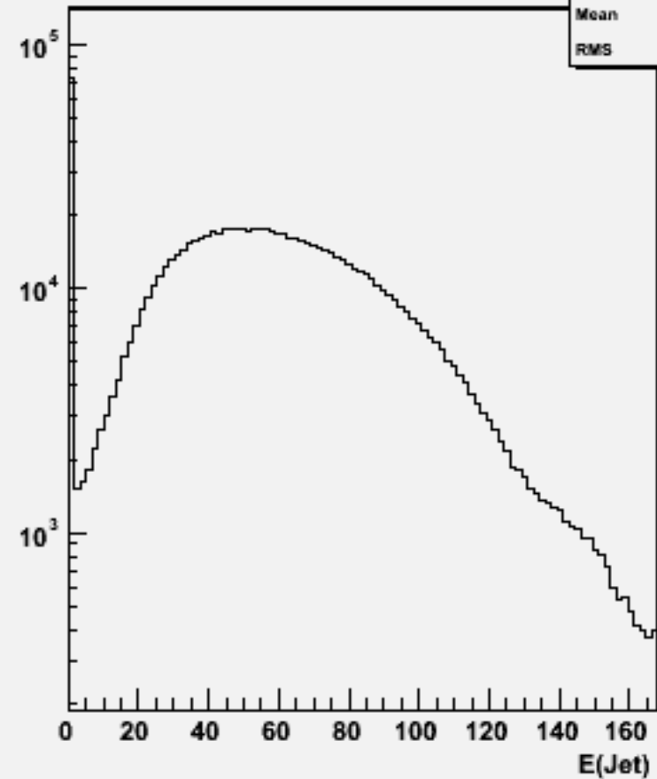
Jet energies(All jets)w100698 e1e1n1e1e1n1_o
