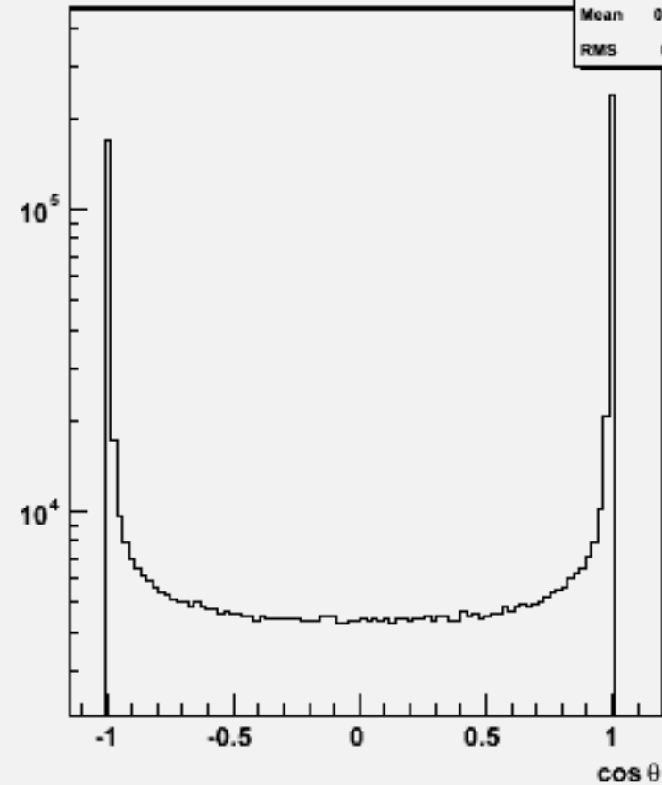
Jet cos \theta (All jets)w100698 e1e1n1e1e1n1_o
