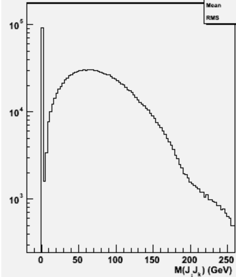
2jets mass(All comb)w100698 e1e1n1e1e1n1_o
