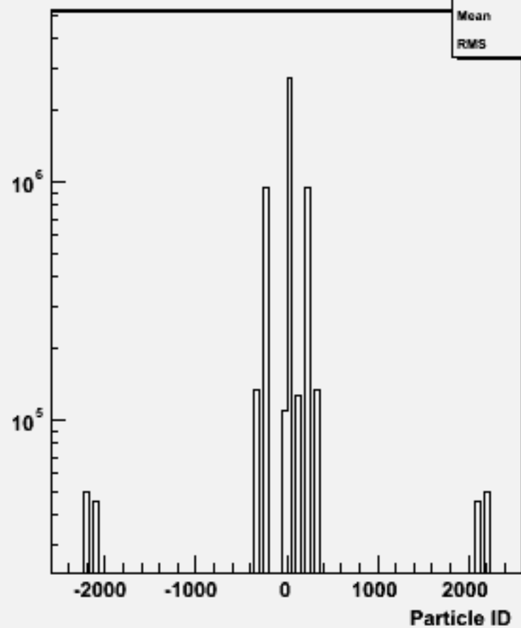
Particle ID : w100692 bbbb_o
