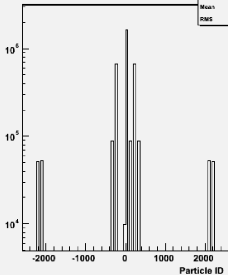
Particle ID : w100677 ddss_o
