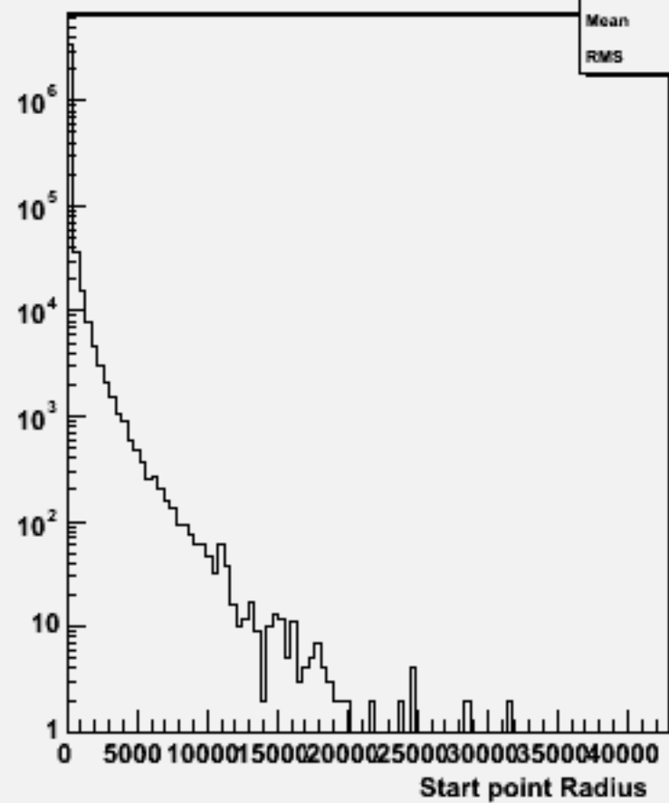
Start point R : w100677 ddss_o
