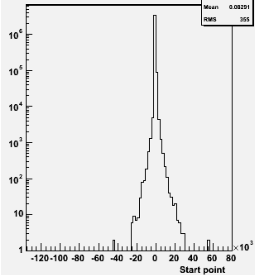
Start point Z : w100677 ddss_o
