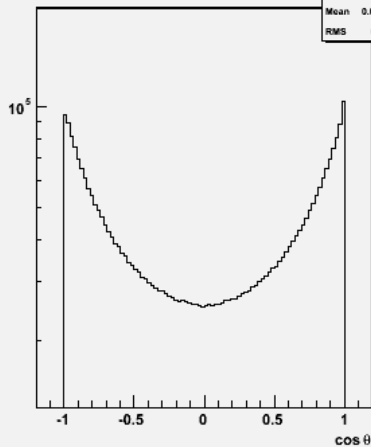
Particle cosθ : w100677 ddss_o
