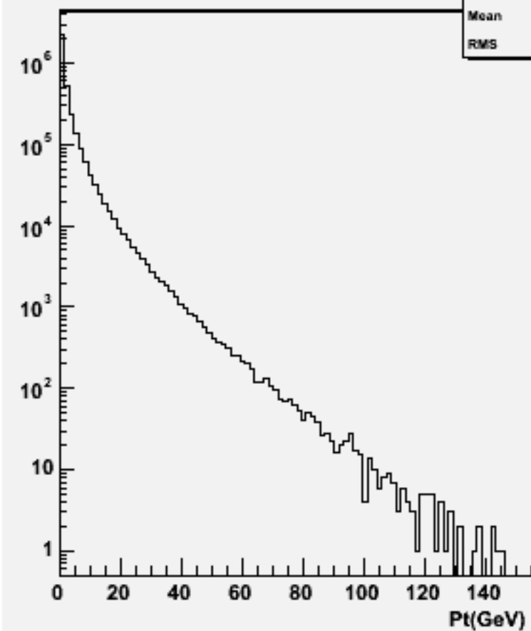
Particle Pt : w100677 ddss_o
