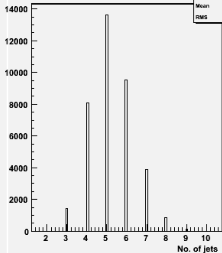
No. jets (ycut=0.001) : w100668 e3e3bb_o
