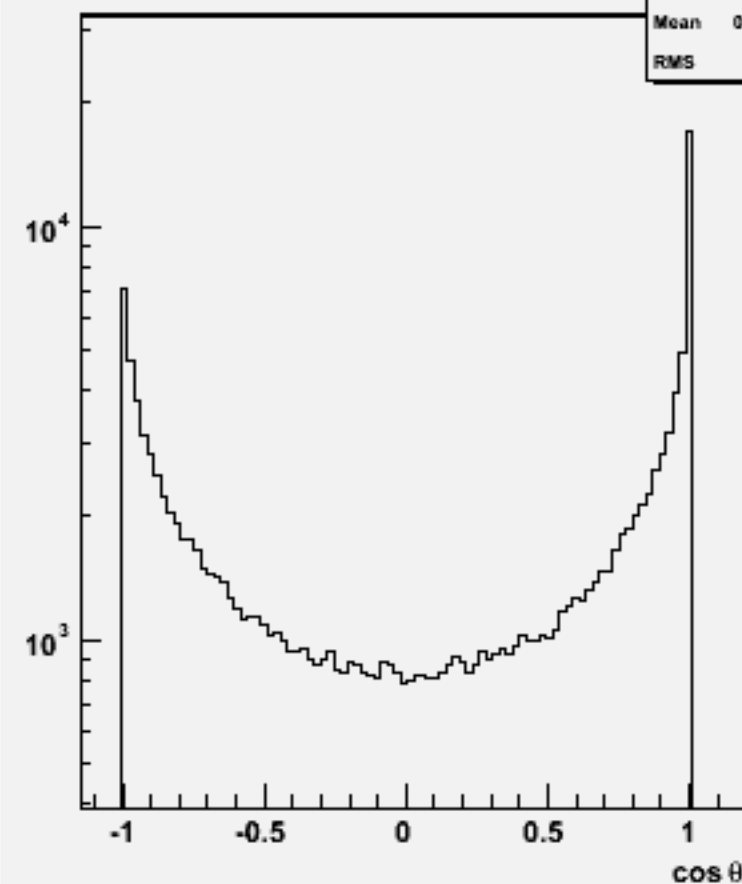
Jet cos \theta (All jets)w100668 e3e3bb_o
