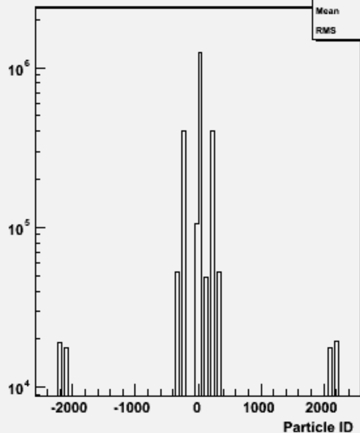
Particle ID : w100668 e3e3bb_o
