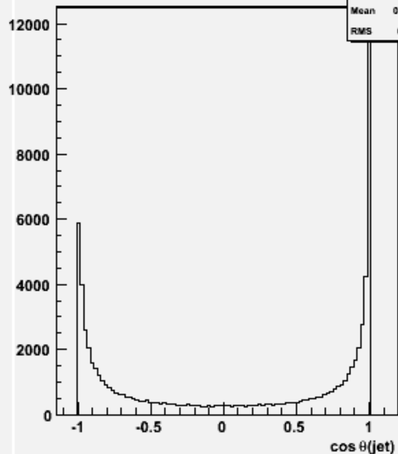
cos \theta for 2-jets :w100668 e3e3bb_o
