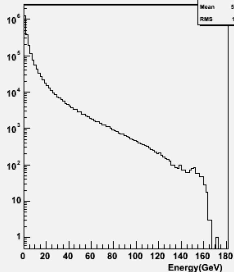
Particle Energy : w100668 e3e3bb_o
