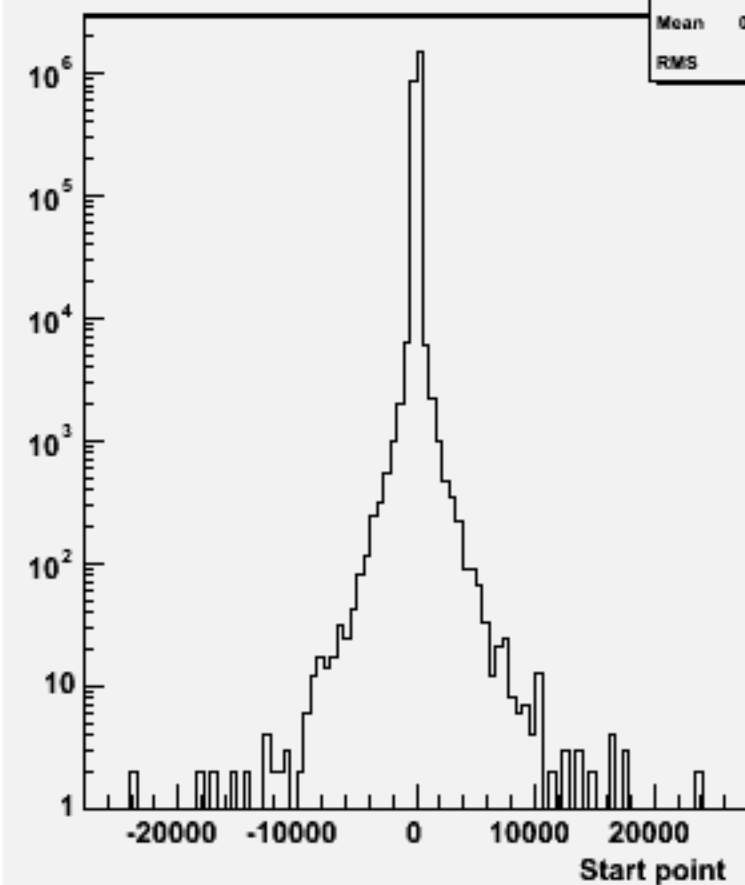
Start point Z : w100668 e3e3bb_o
