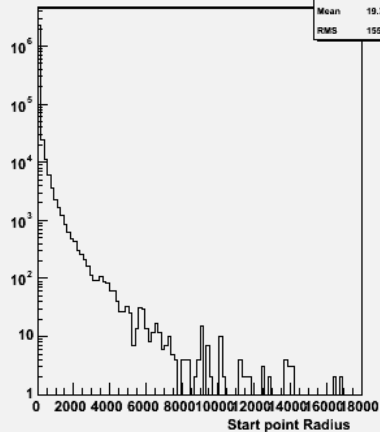
Start point R : w100668 e3e3bb_o
