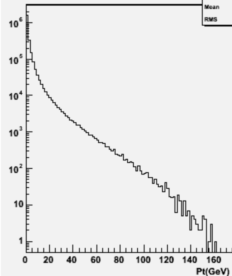
Particle Pt : w100668 e3e3bb_o
