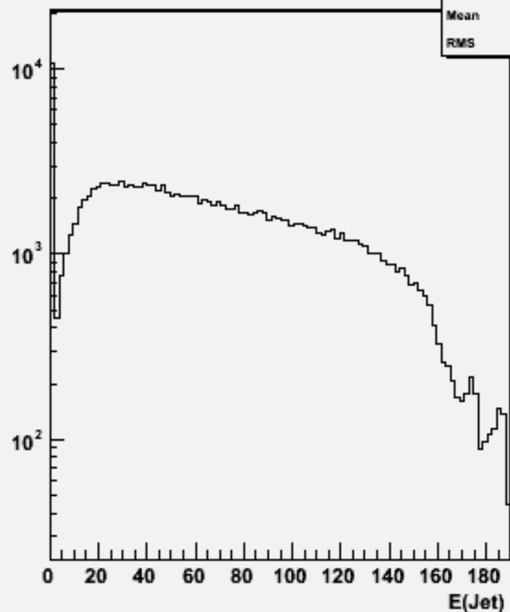
Jet energies(All jets)w100668 e3e3bb_o
