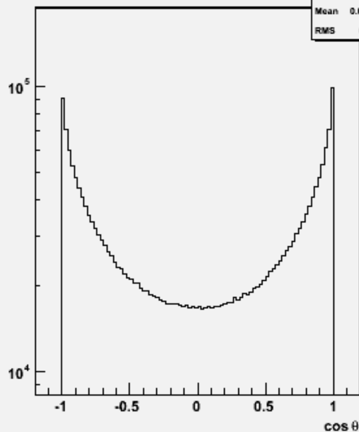
Particle cos \theta : w100668 e3e3bb_o
