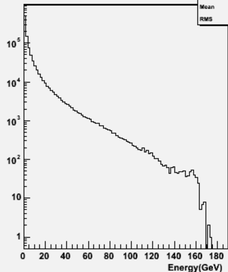
Particle Energy : w100661 e3e3dd_o
