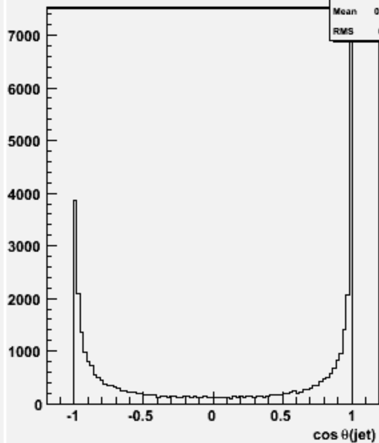
cos \theta for 2-jets :w100661 e3e3dd_o
