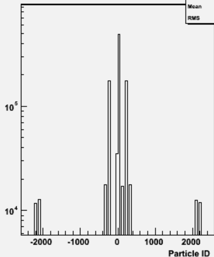
Particle ID : w100661 e3e3dd_o
