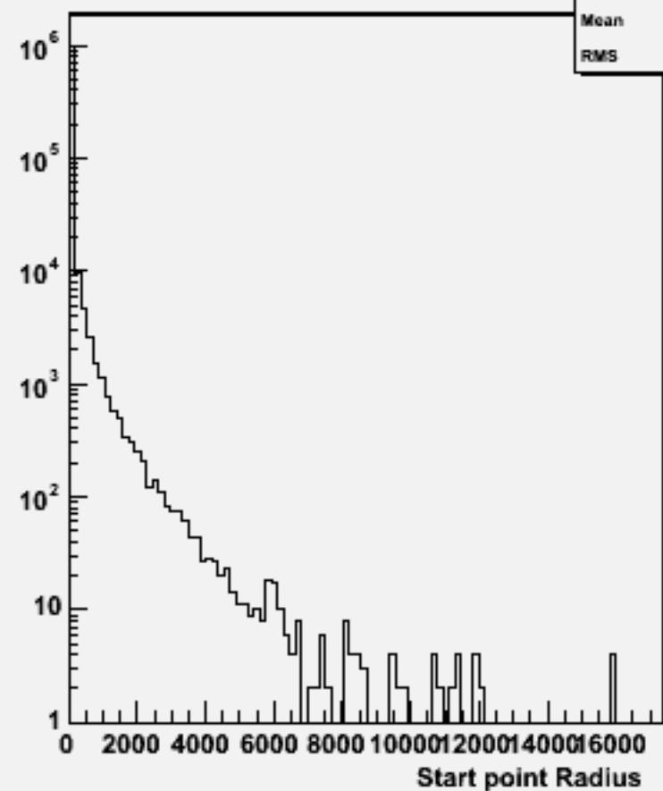
Start point R : w100661 e3e3dd_o
