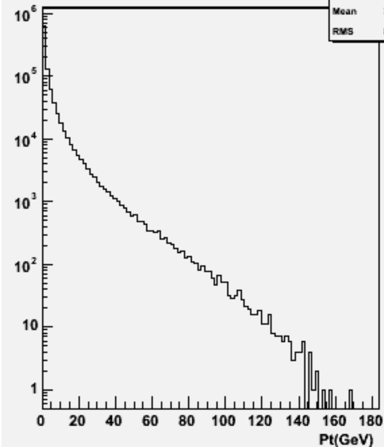
Particle Pt : w100661 e3e3dd_o
