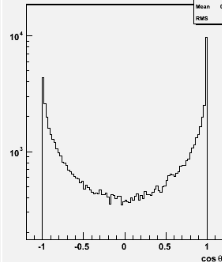
Jet cos \theta (All jets)w100661 e3e3dd_o
