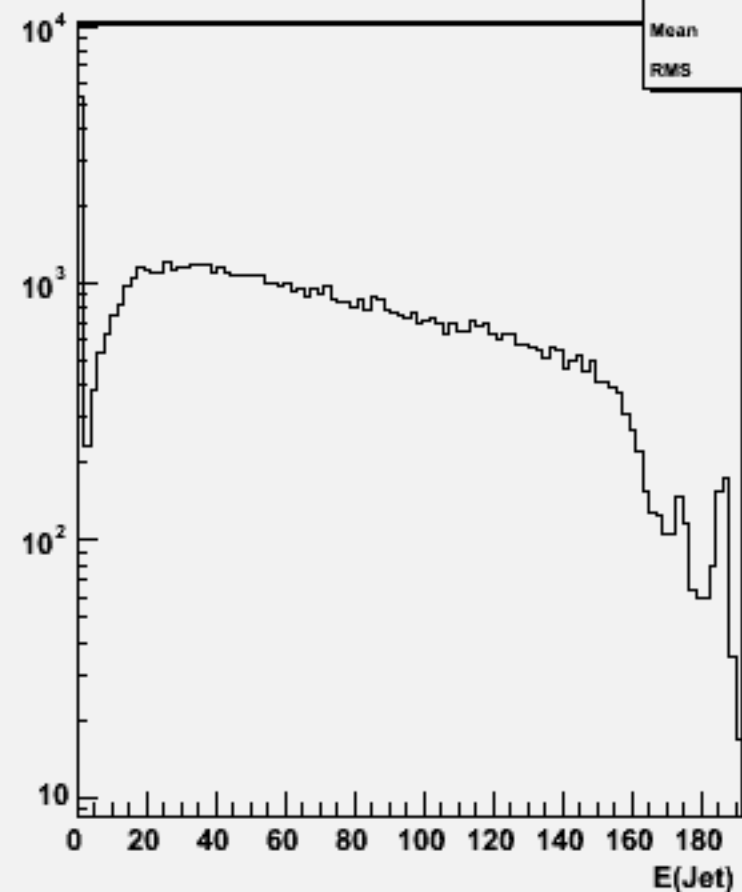
Jet energies(All jets)w100661 e3e3dd_o
