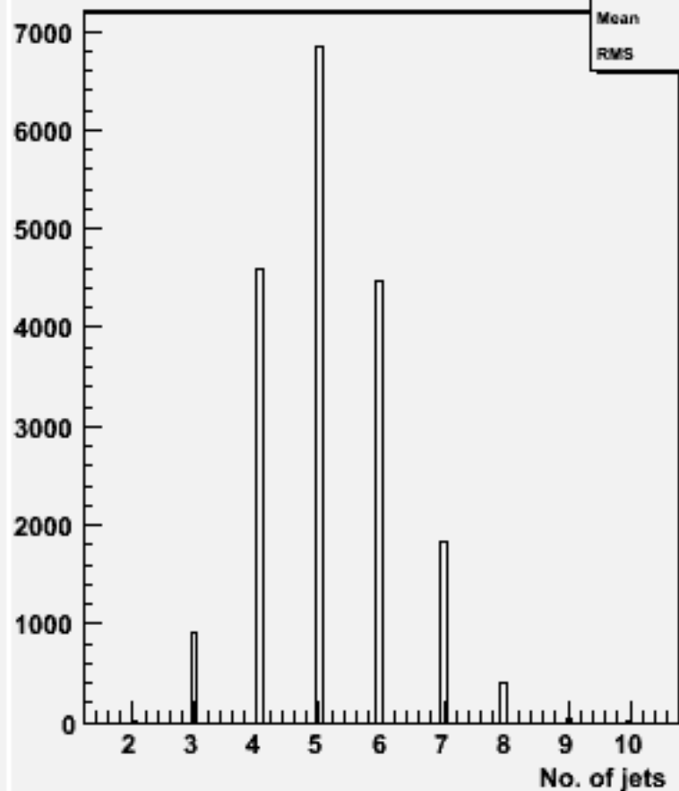
No. jets (ycut=0.001) : w100661 e3e3dd_o
