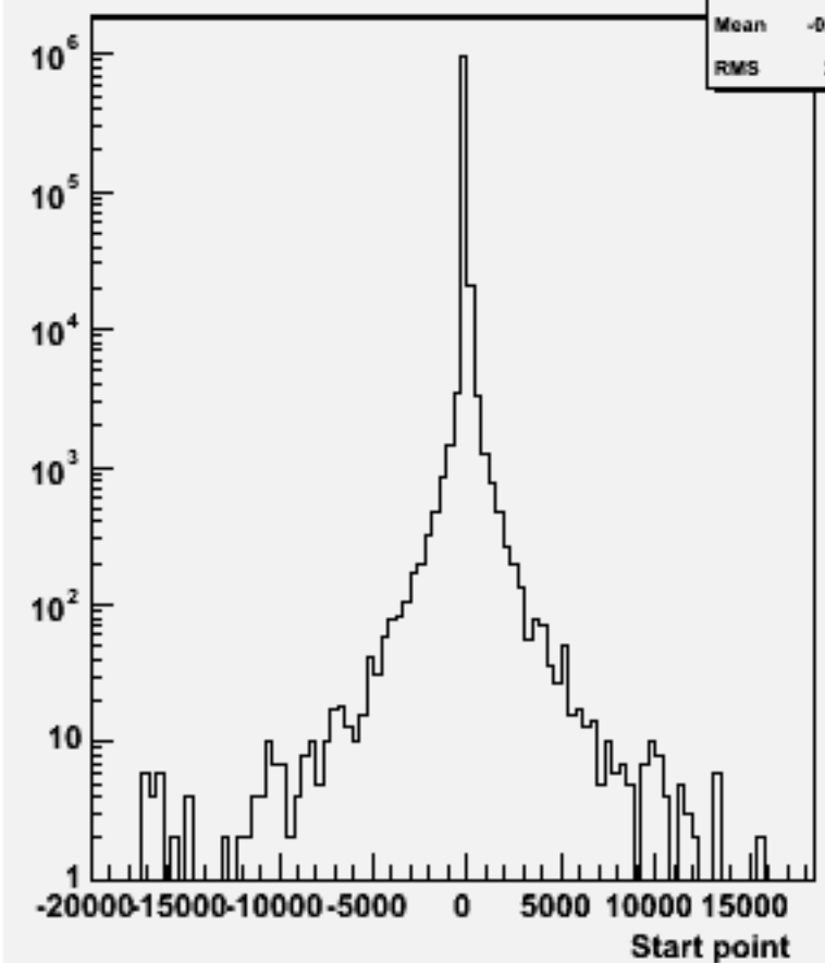
Start point Z : w100661 e3e3dd_o
