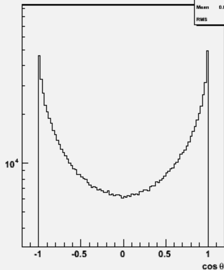
Particle cosθ : w100661 e3e3dd_o
