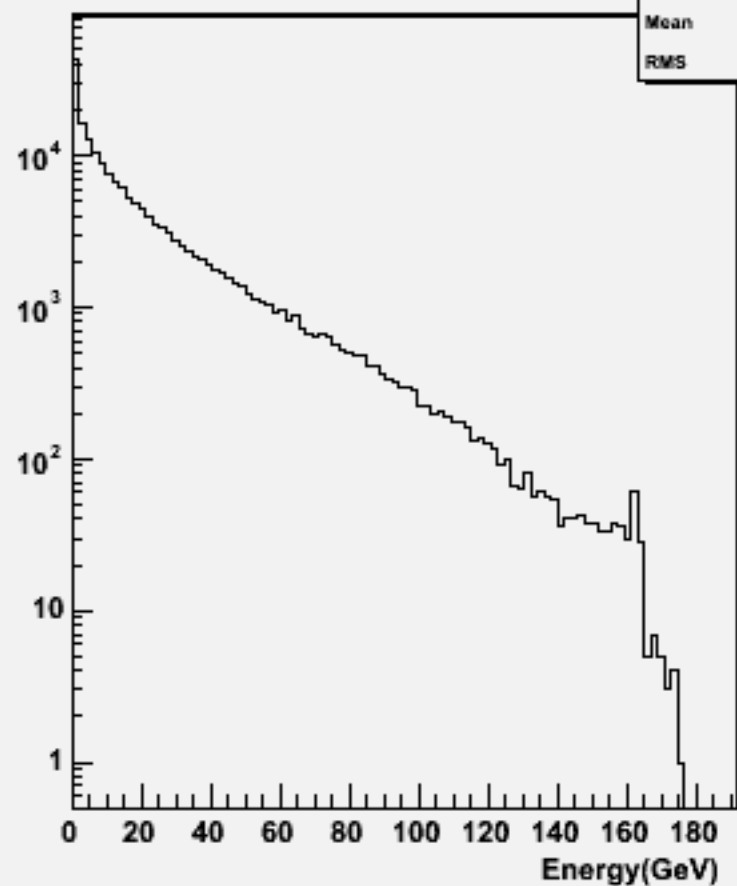
Particle Energy : w100656 e3e3e3e3_o
