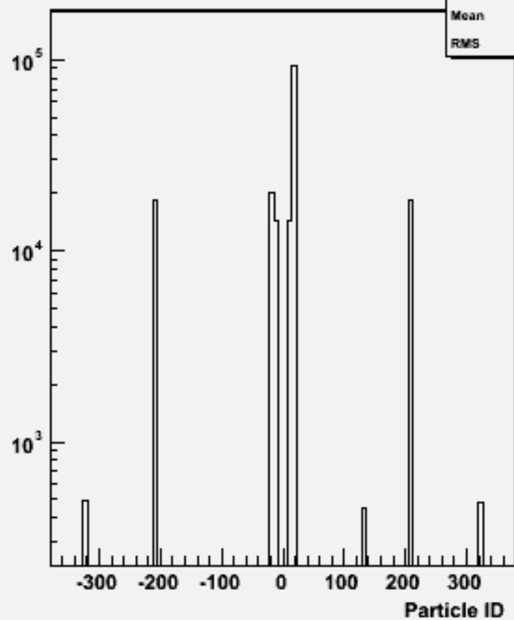
Particle ID : w100656 e3e3e3e3_o
