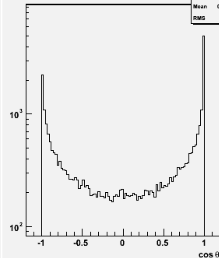
Jet cosθ (All jets)w100656 e3e3e3e3_o
