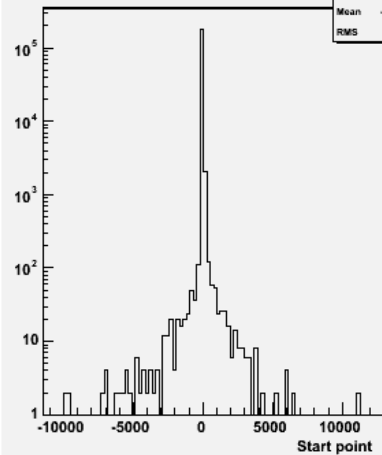
Start point Z : w100656 e3e3e3e3_o
