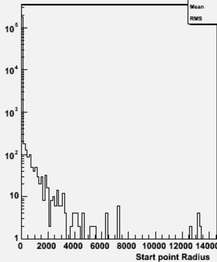
Start point R : w100656 e3e3e3e3_o
