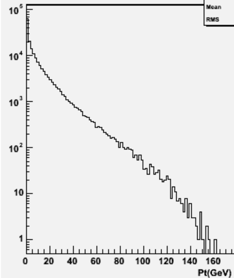
Particle Pt : w100656 e3e3e3e3_o
