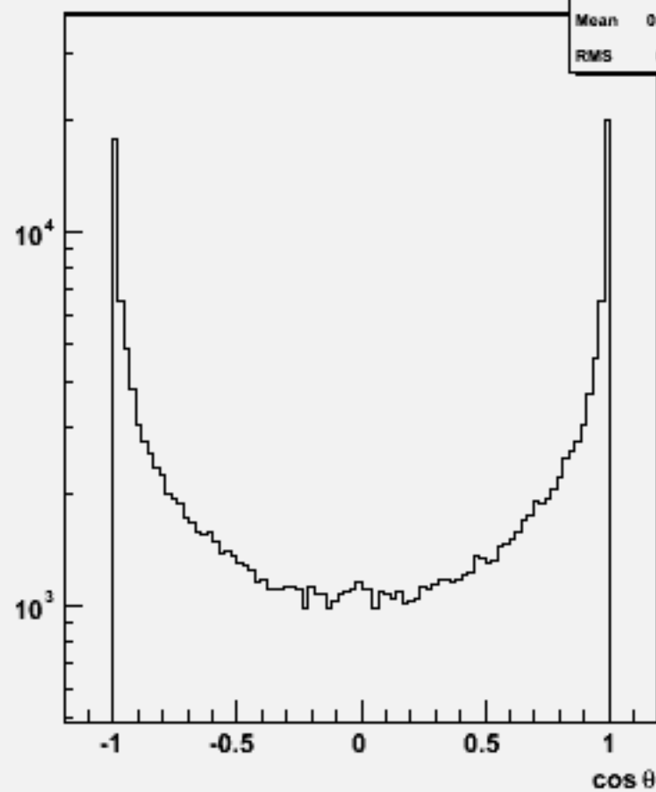
Particle cos \theta : w100656 e3e3e3e3_o
