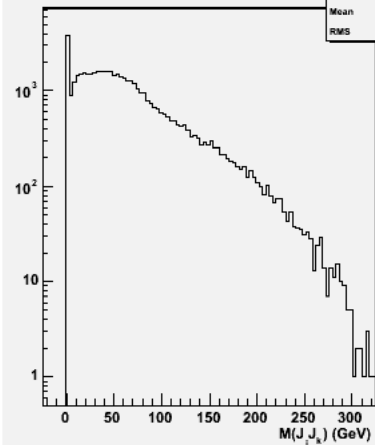
2jets mass(All comb)w100656 e3e3e3e3_o
