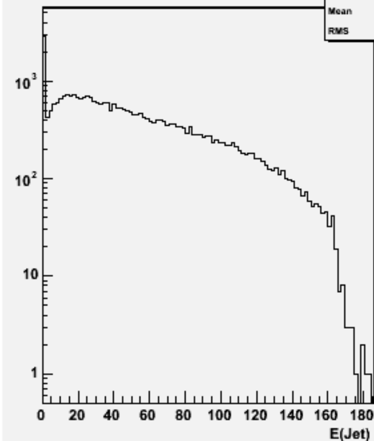
Jet energies(All jets)w100656 e3e3e3e3_o
