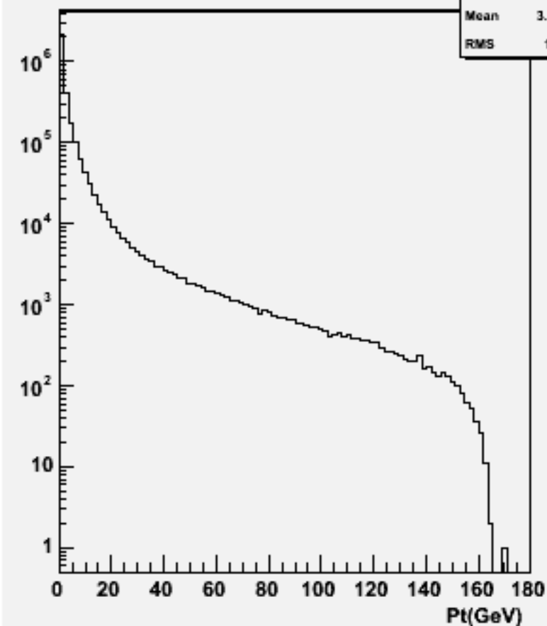
Particle Pt : w100648 e2e2ss_o
