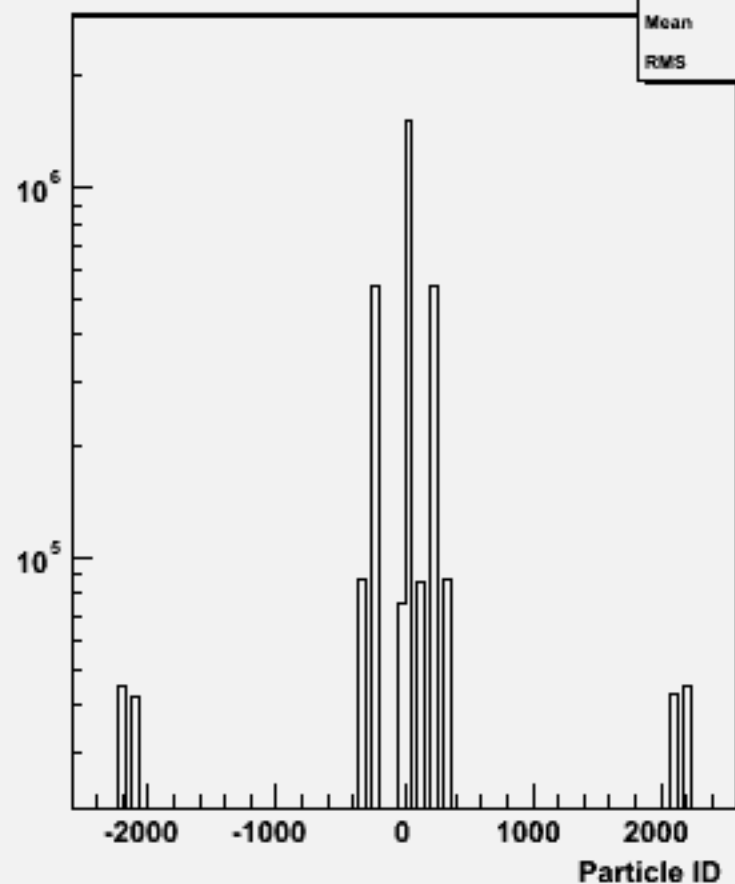
Particle ID : w100648 e2e2ss_o
