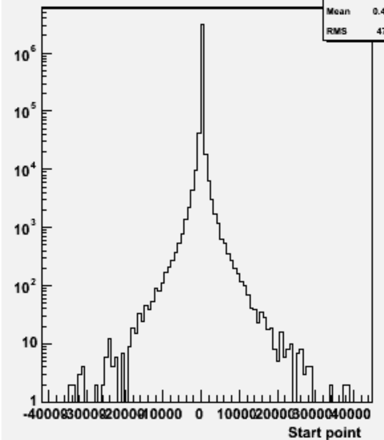
Start point Z : w100648 e2e2ss_o
