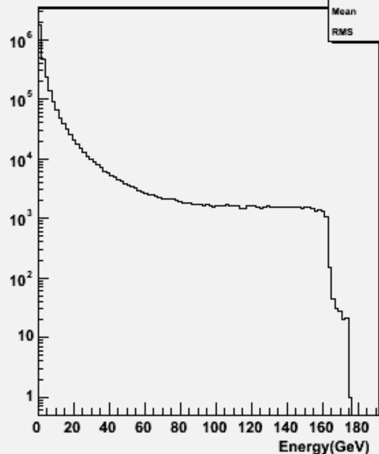
Particle Energy : w100648 e2e2ss_o
