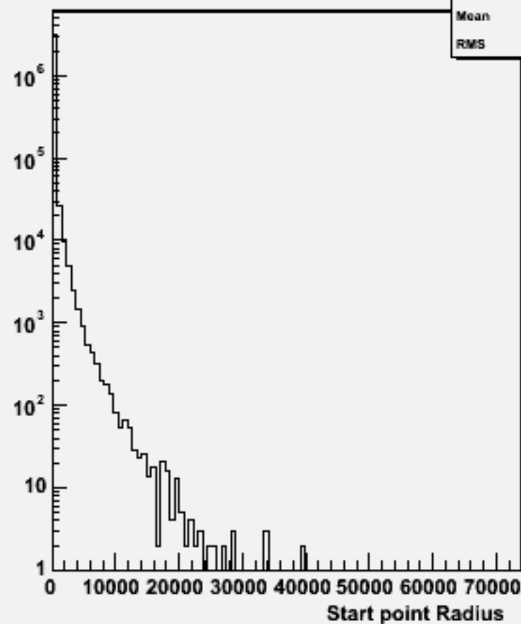
Start point R : w100648 e2e2ss_o
