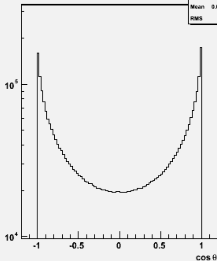
Particle cosθ : w100648 e2e2ss_o
