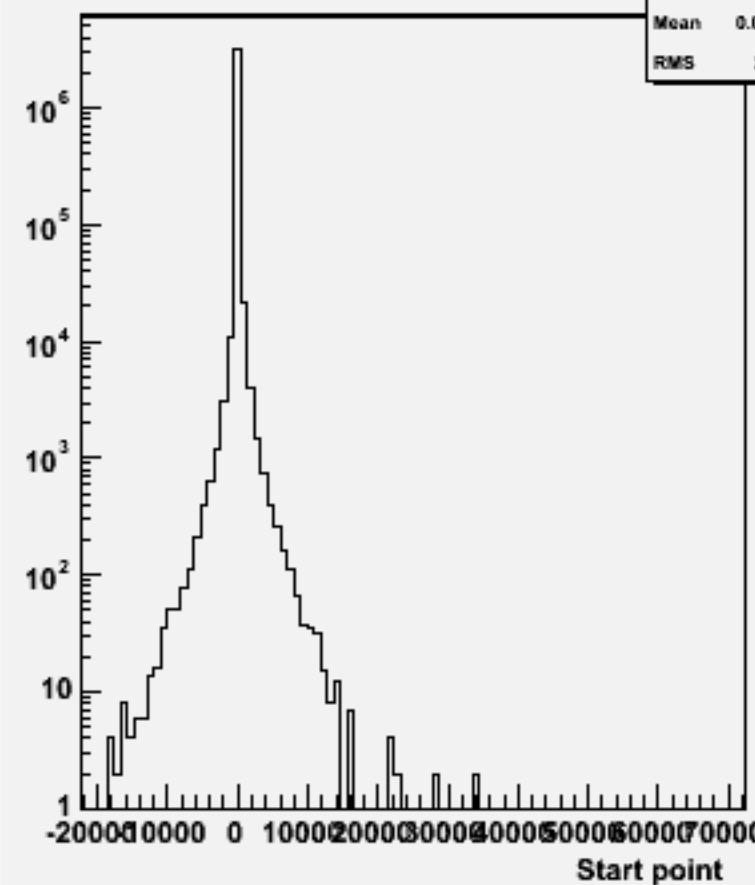
Start point Z : w100644 e2e2dd_o
