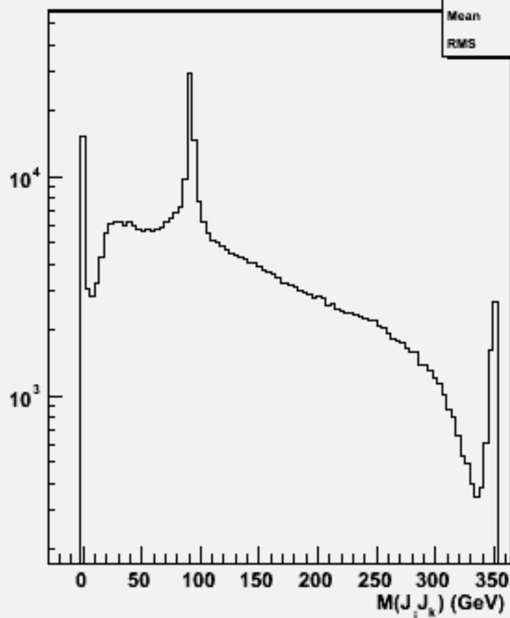
2jets mass(All comb)w100644 e2e2dd_o
