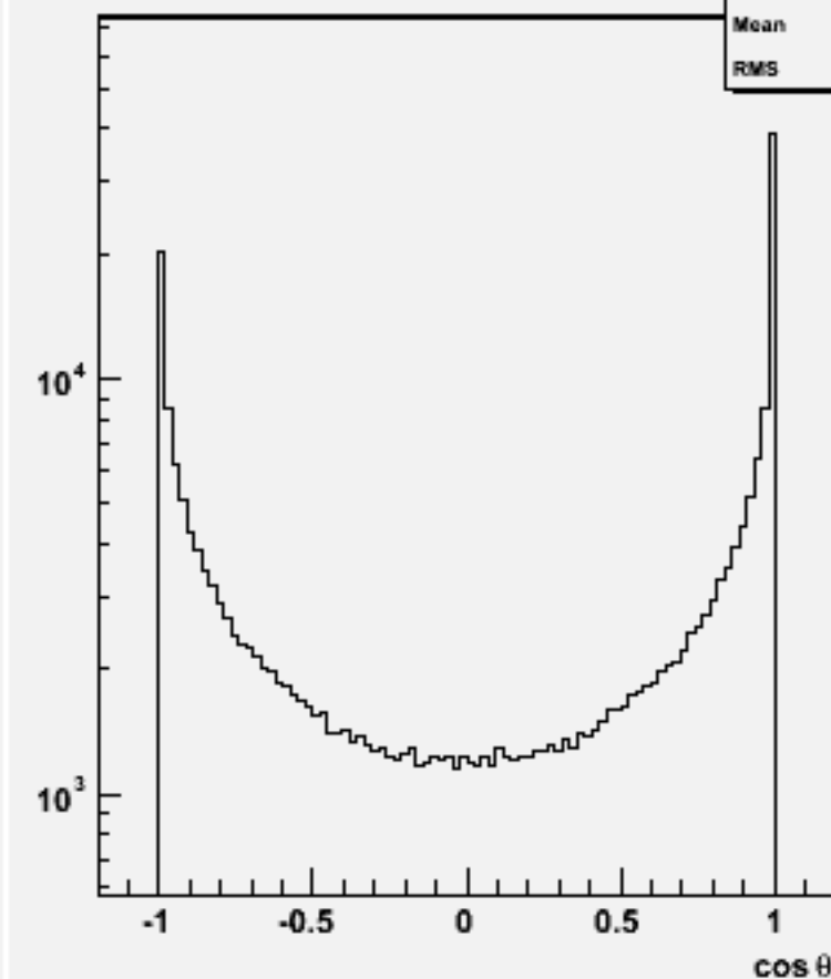
Jet cos \theta (All jets)w100644 e2e2dd_o
