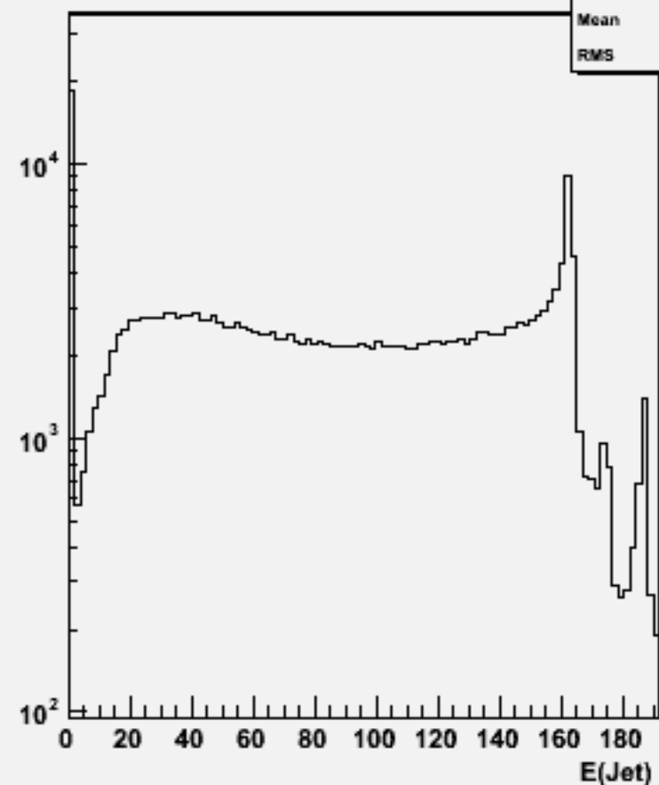
Jet energies(All jets)w100644 e2e2dd_o
