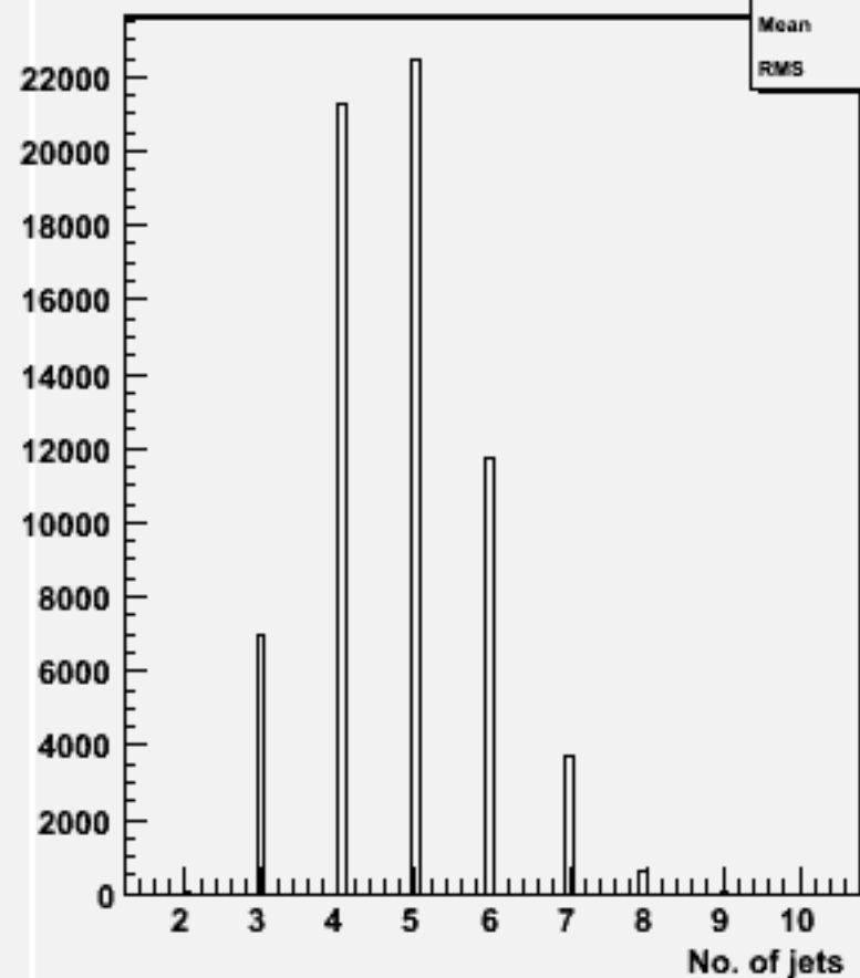
No. jets (ycut=0.001) : w100644 e2e2dd_o
