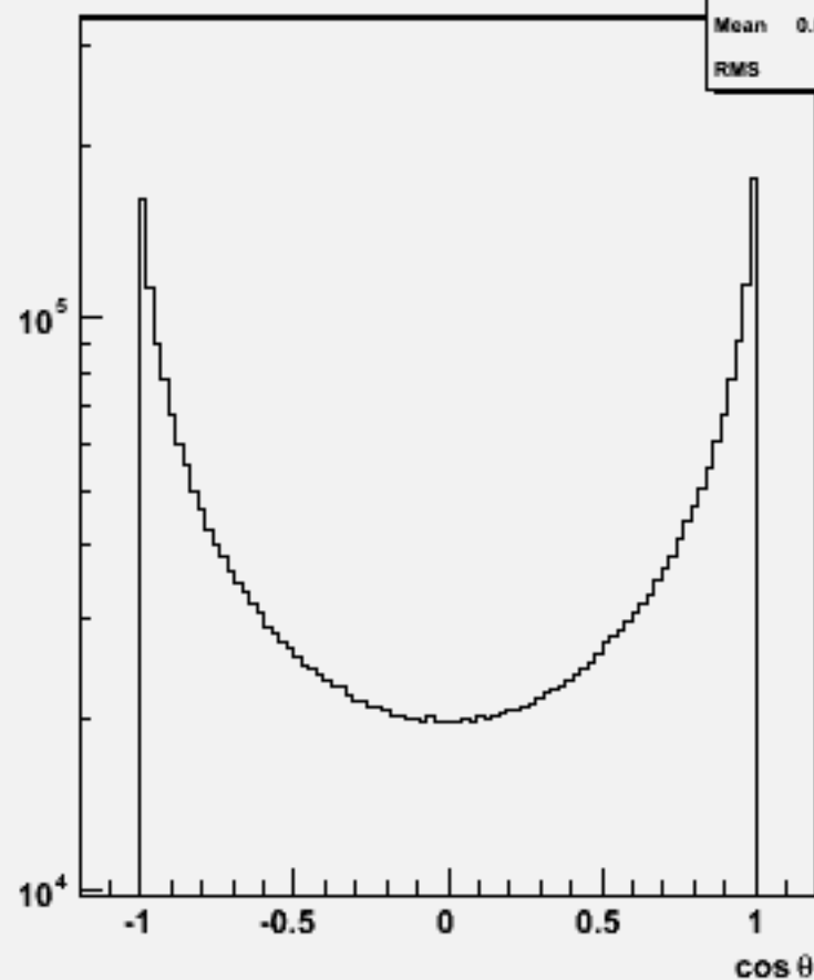
Particle cosθ : w100644 e2e2dd_o
