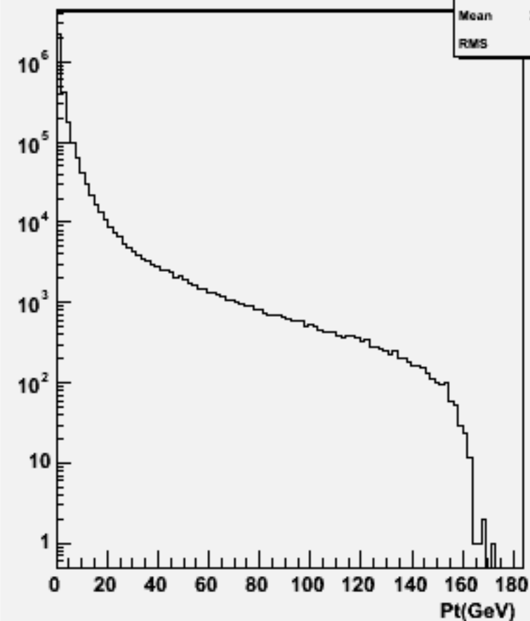
Particle Pt : w100644 e2e2dd_o
