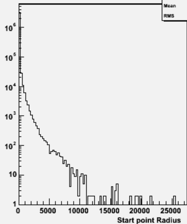
Start point R : w100644 e2e2dd_o
