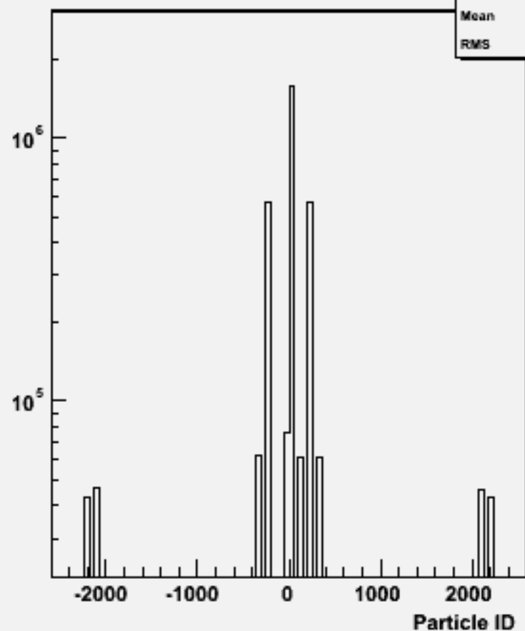
Particle ID : w100644 e2e2dd_o
