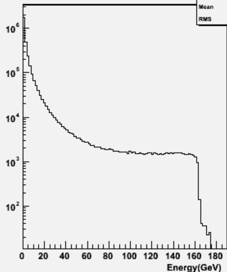
Particle Energy : w100644 e2e2dd_o
