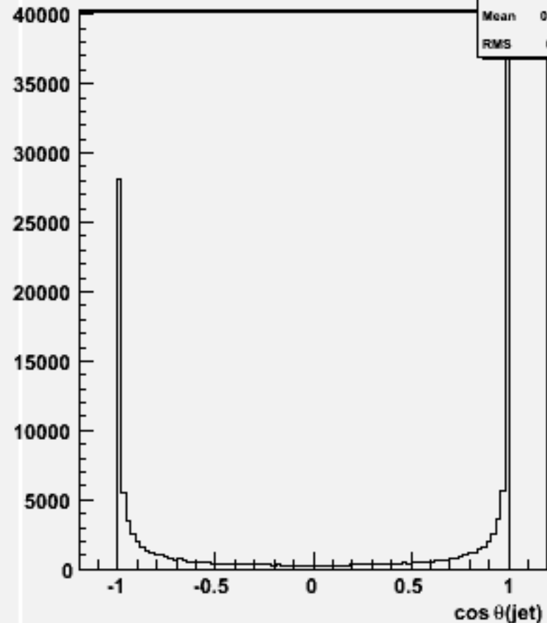
cos \theta for 2-jets :w100644 e2e2dd_o
