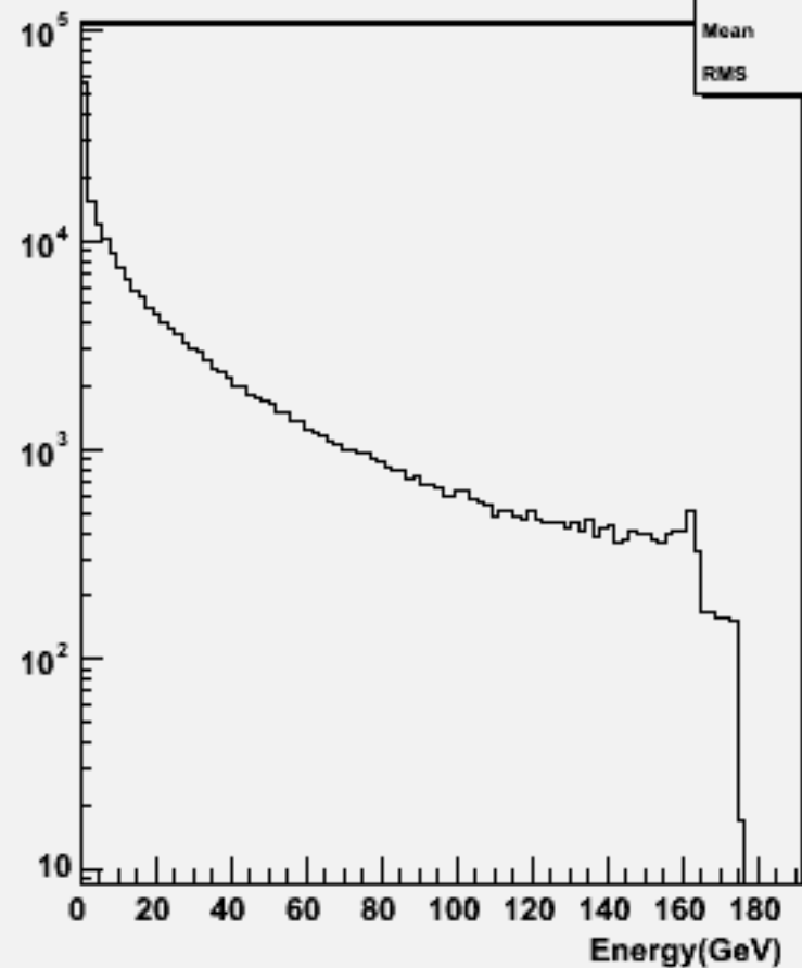
Particle Energy : w100641 e2e2e3e3_o
