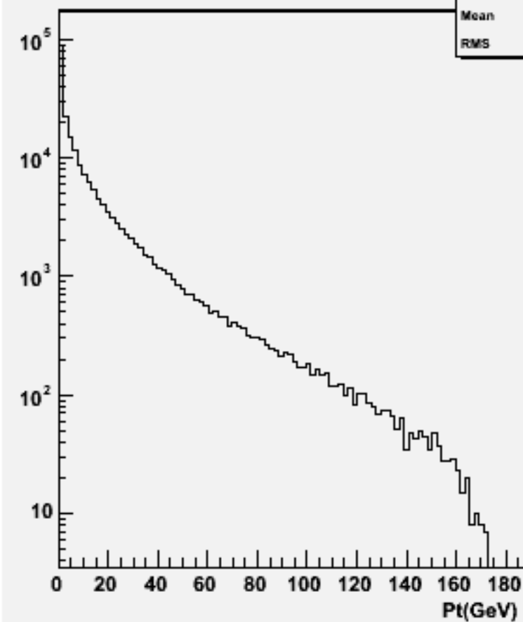
Particle Pt : w100641 e2e2e3e3_o
