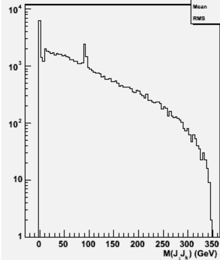
2jets mass(All comb)w100641 e2e2e3e3_o
