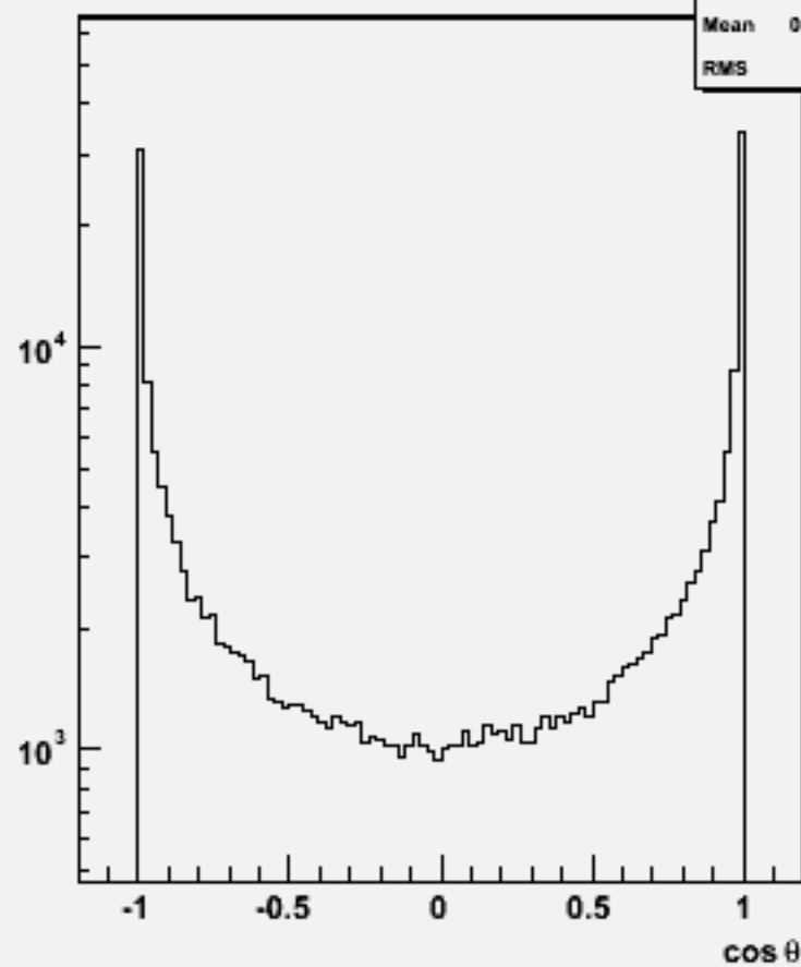
Particle cos \theta : w100641 e2e2e3e3_o
