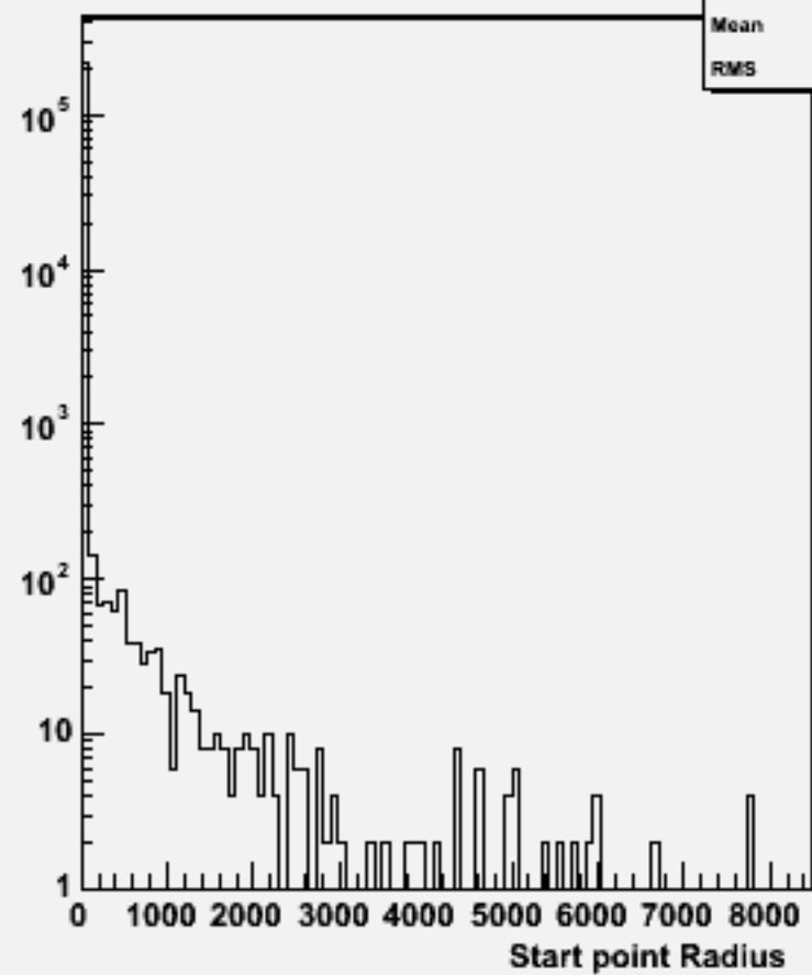
Start point R : w100641 e2e2e3e3_o
