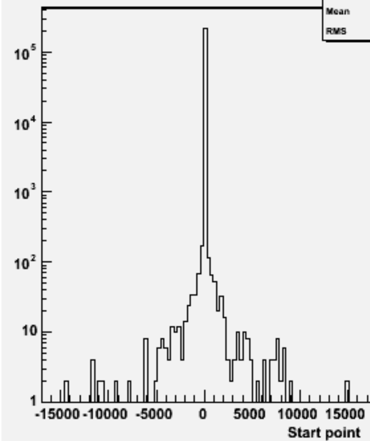
Start point Z : w100641 e2e2e3e3_o
