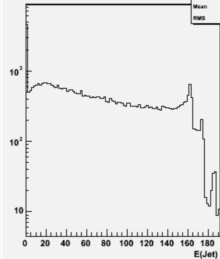
Jet energies(All jets)w100641 e2e2e3e3_o
