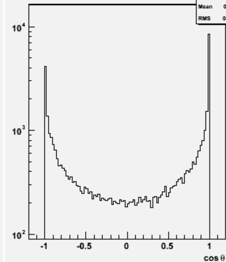
Jet cosθ (All jets)w100641 e2e2e3e3_o
