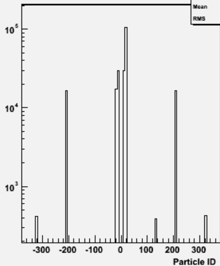
Particle ID : w100641 e2e2e3e3_o
