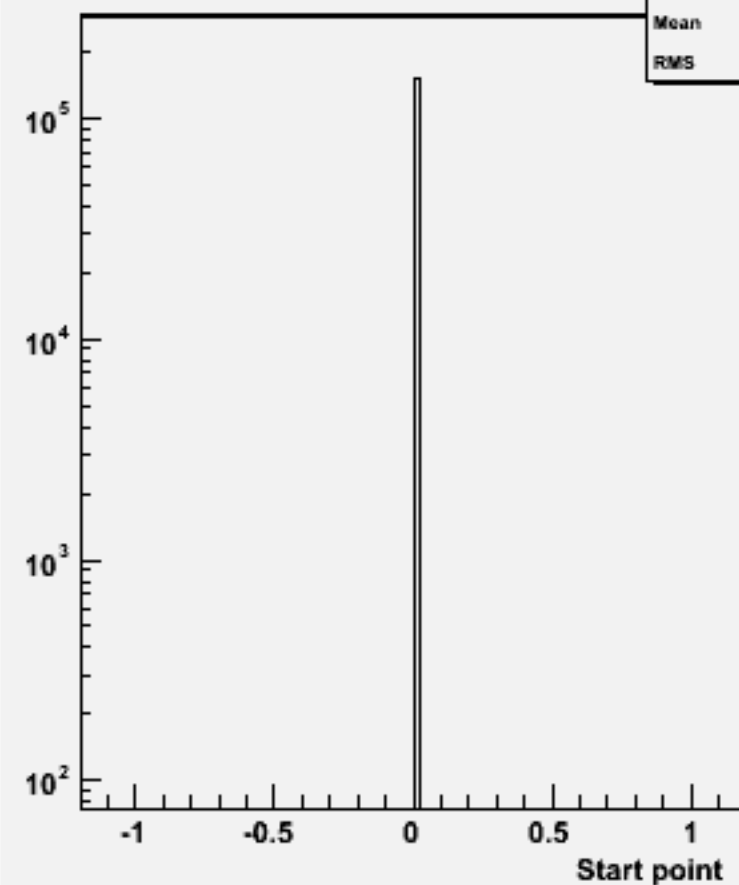
Start point Z : w100636 e2e2e2e2_o
