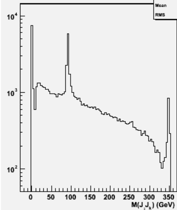
2jets mass(All comb)w100636 e2e2e2e2_o
