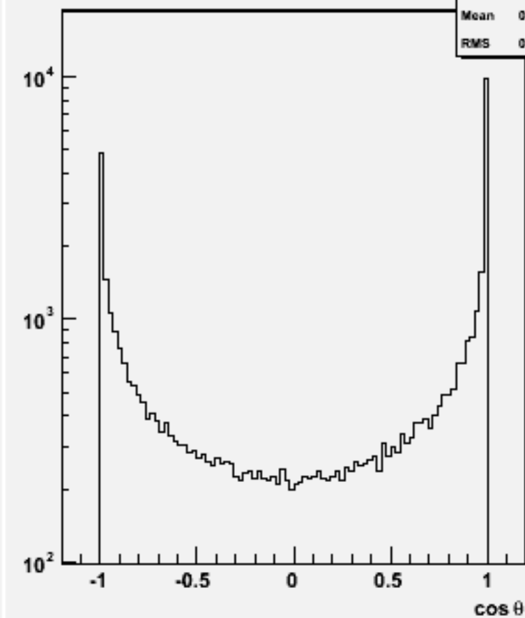
Jet cos \theta (All jets)w100636 e2e2e2e2_o
