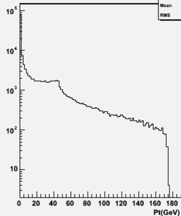
Particle Pt : w100636 e2e2e2e2_o
