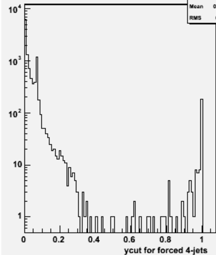
Ycut for 4-jets :w100636 e2e2e2e2_o
