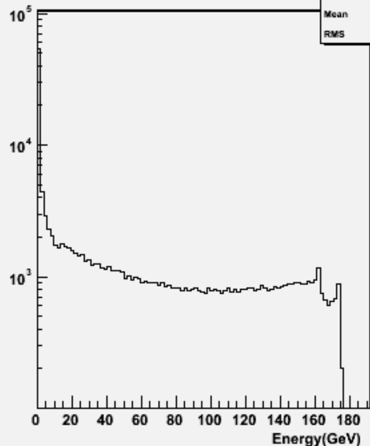
Particle Energy : w100636 e2e2e2e2_o
