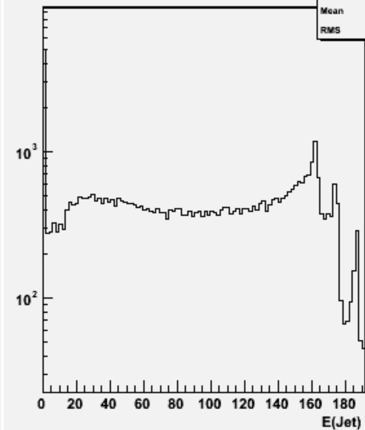
Jet energies(All jets)w100636 e2e2e2e2_o
