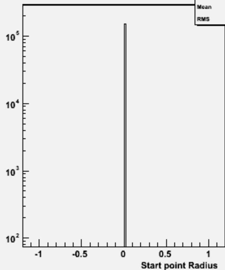
Start point R : w100636 e2e2e2e2_o
