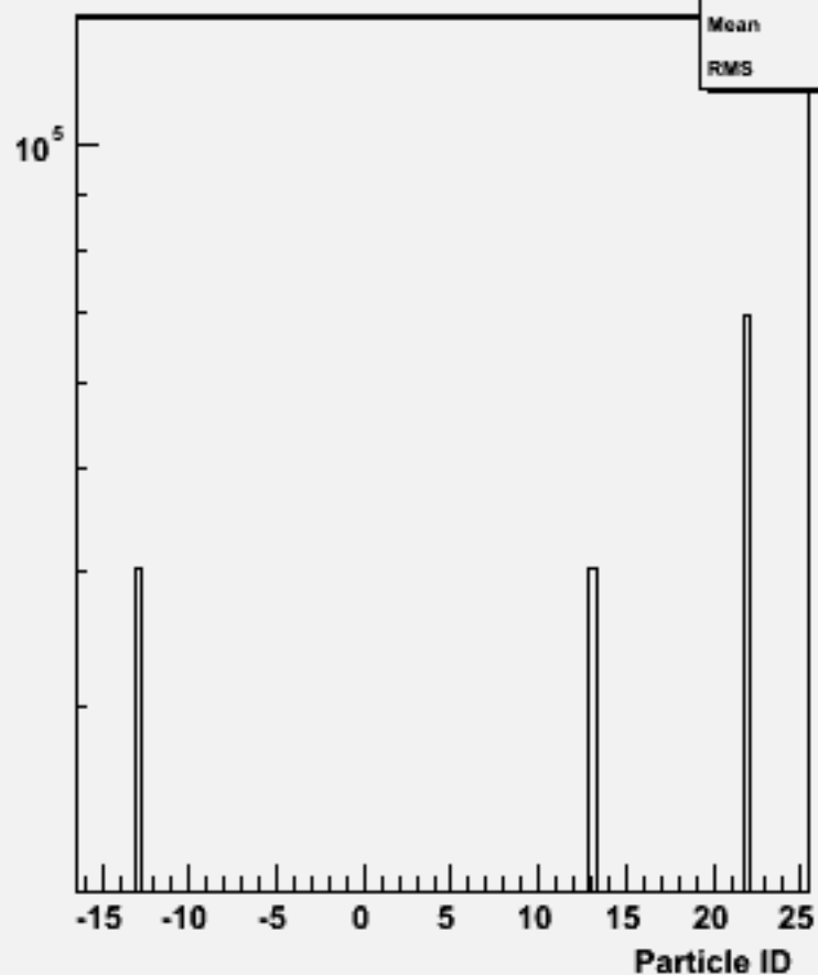
Particle ID : w100636 e2e2e2e2_o
