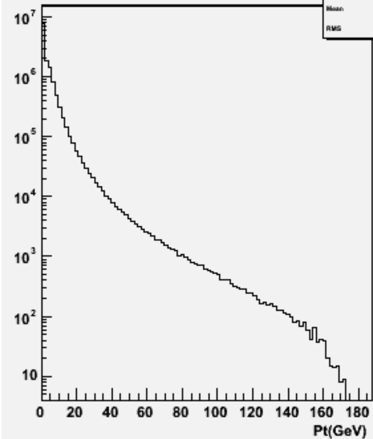
Start point Z : w100621 e1e1e3e3_o
