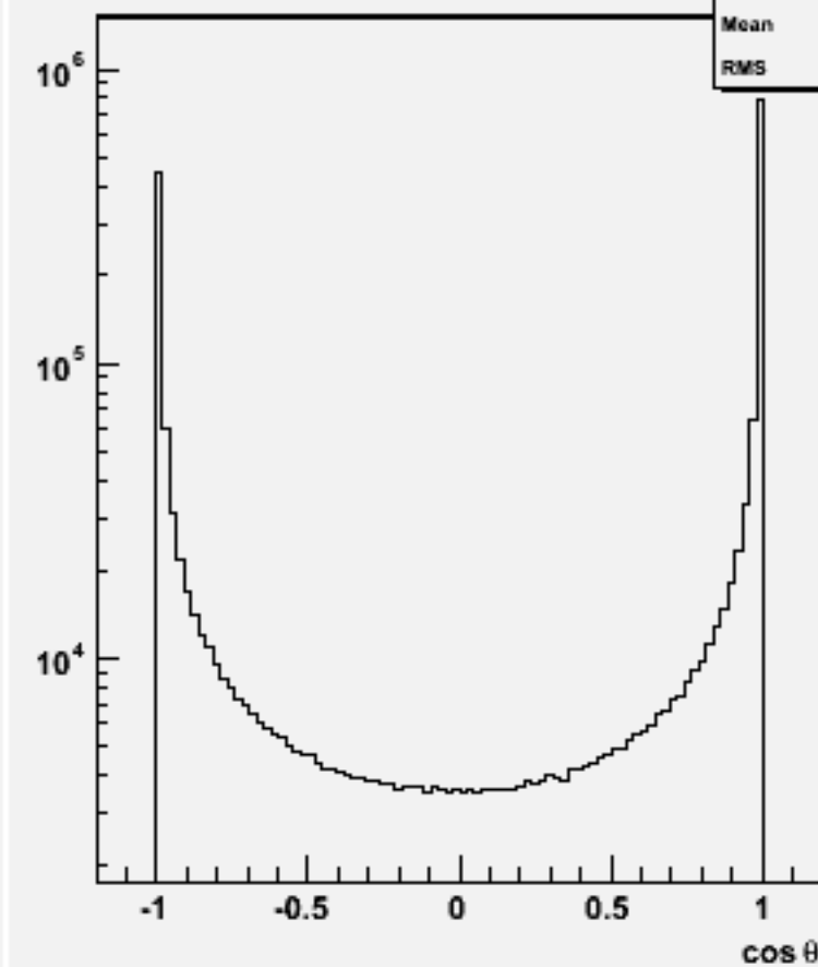
Jet cosθ (All jets)w100621 e1e1e3e3_o
