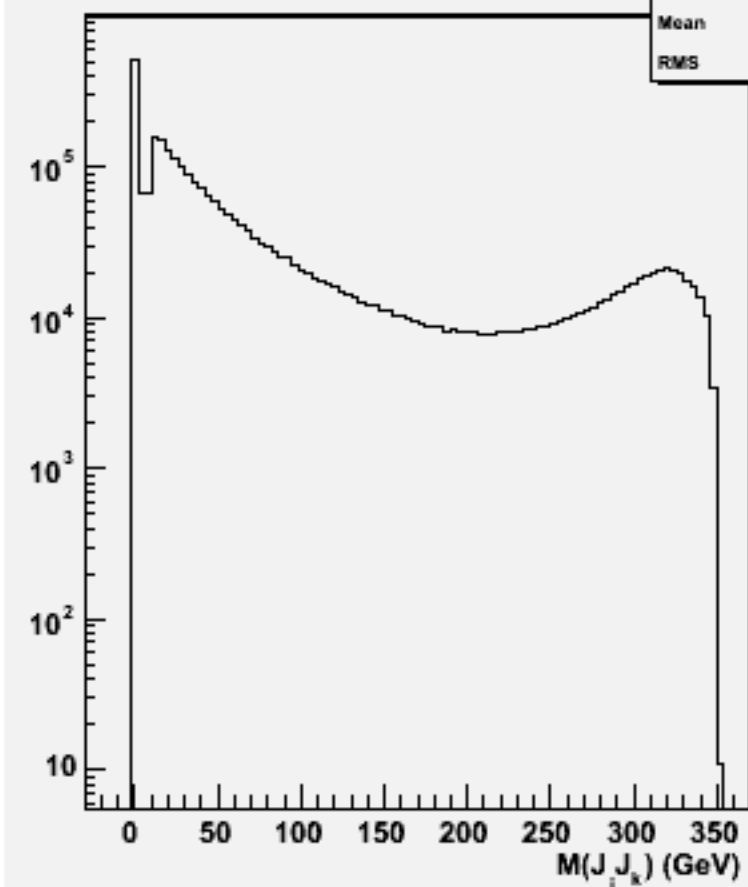
2jets mass(All comb)w100621 e1e1e3e3_o
