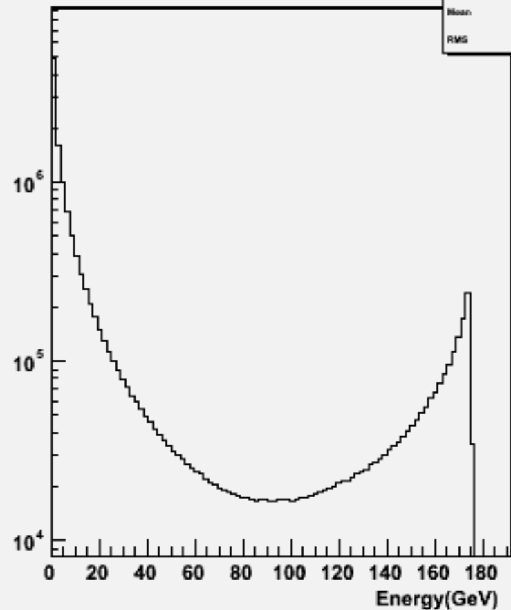
Start point R : w100621 e1e1e3e3_o
