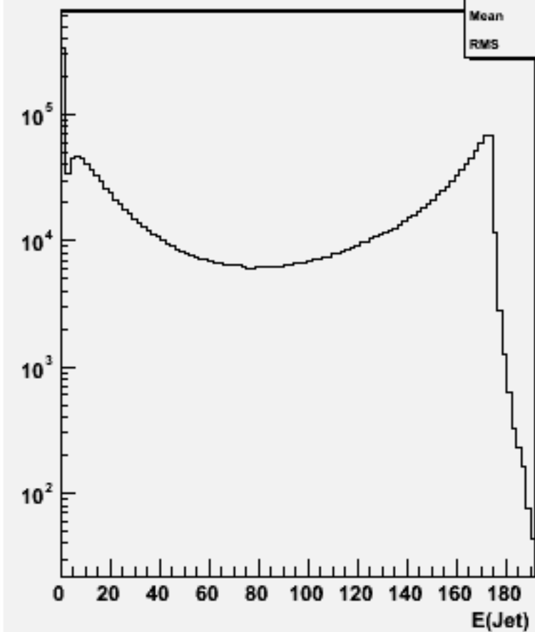
Jet energies(All jets)w100621 e1e1e3e3_o
