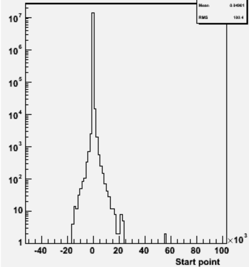
Start point Z : w100621 e1e1e3e3_o
