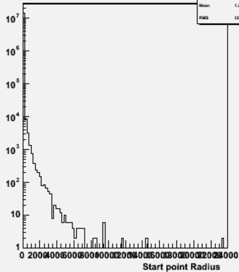
Start point R : w100621 e1e1e3e3_o
