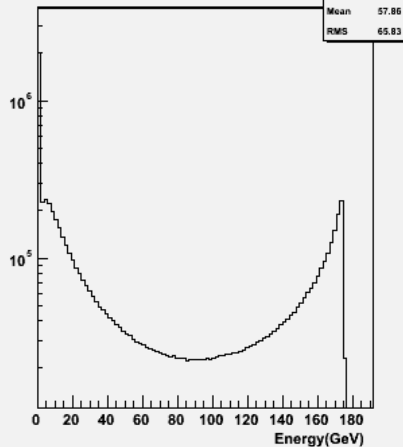
Particle Energy : w100613 e1e1e1e1_o
