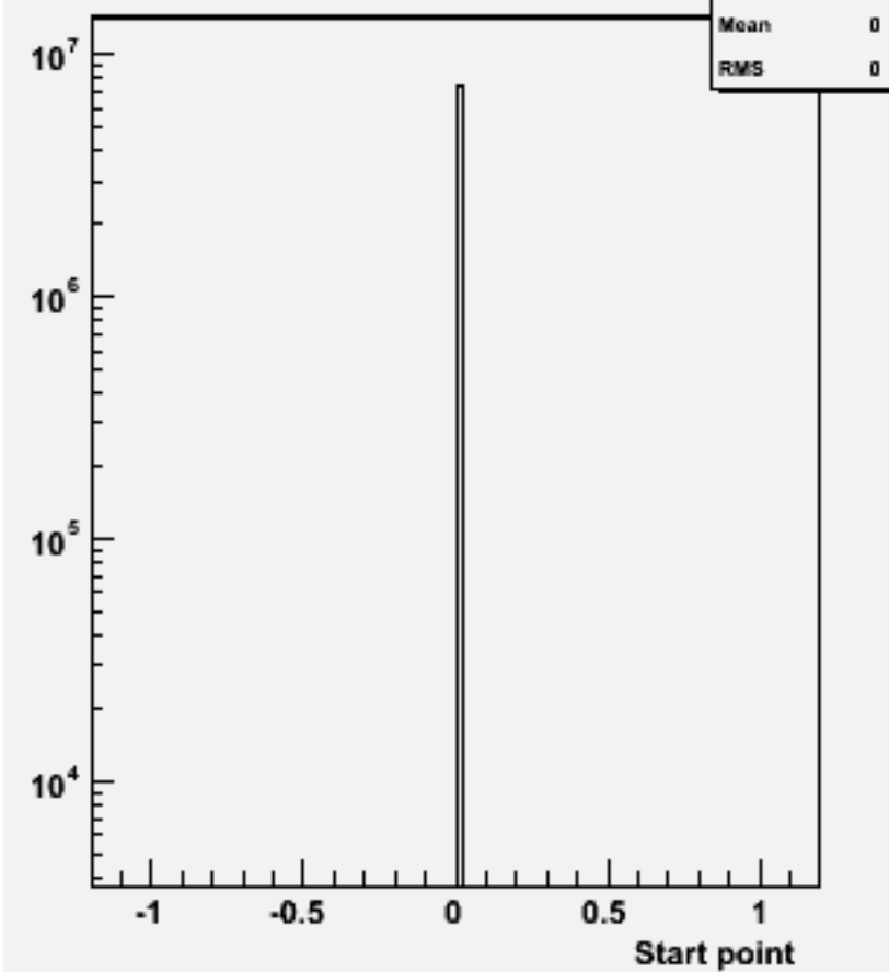
Start point Z : w100613 e1e1e1e1_o
