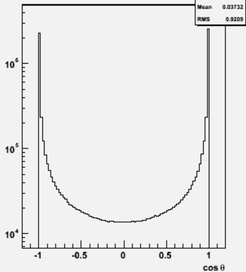
Particle cos \theta : w100613 e1e1e1e1_o
