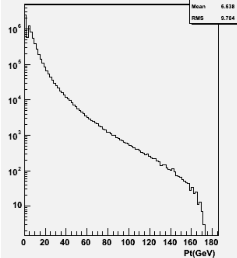
Particle Pt : w100613 e1e1e1e1_o
