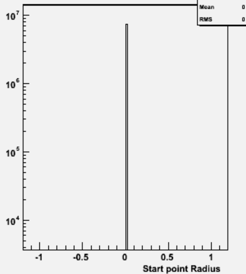
Start point R : w100613 e1e1e1e1_o
