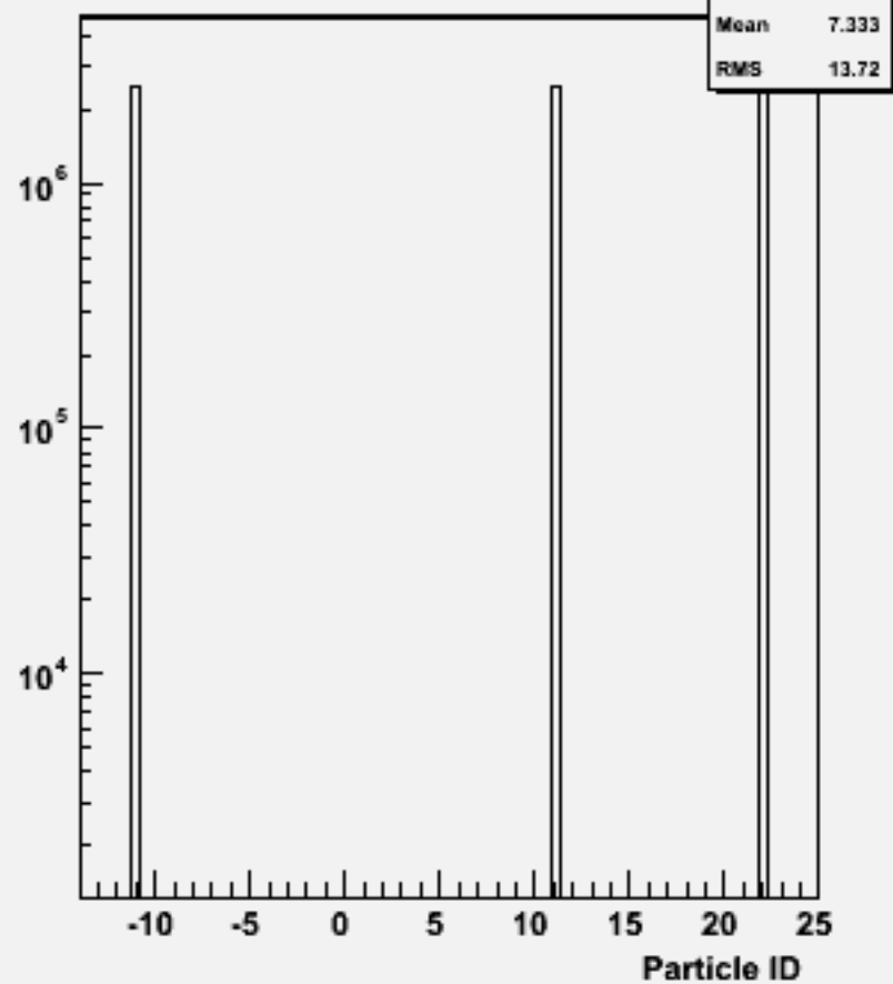
Particle ID : w100613 e1e1e1e1_o
