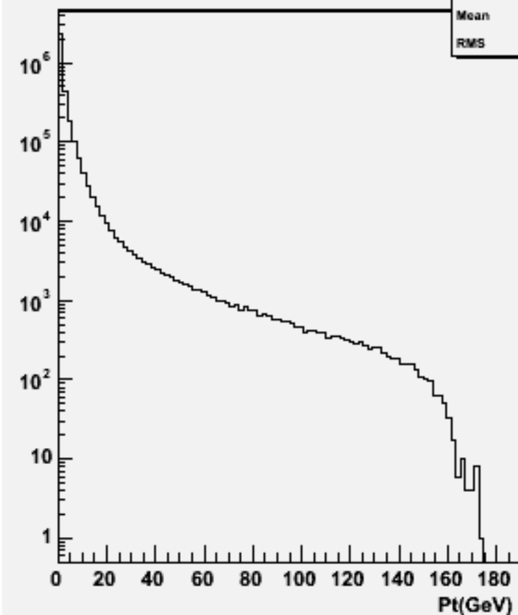
Particle Pt : w100596 cce2e2_o
