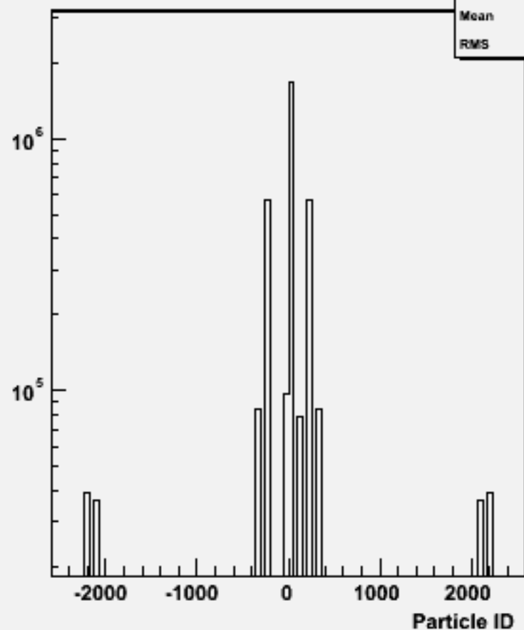
Particle ID : w100596 cce2e2_o
