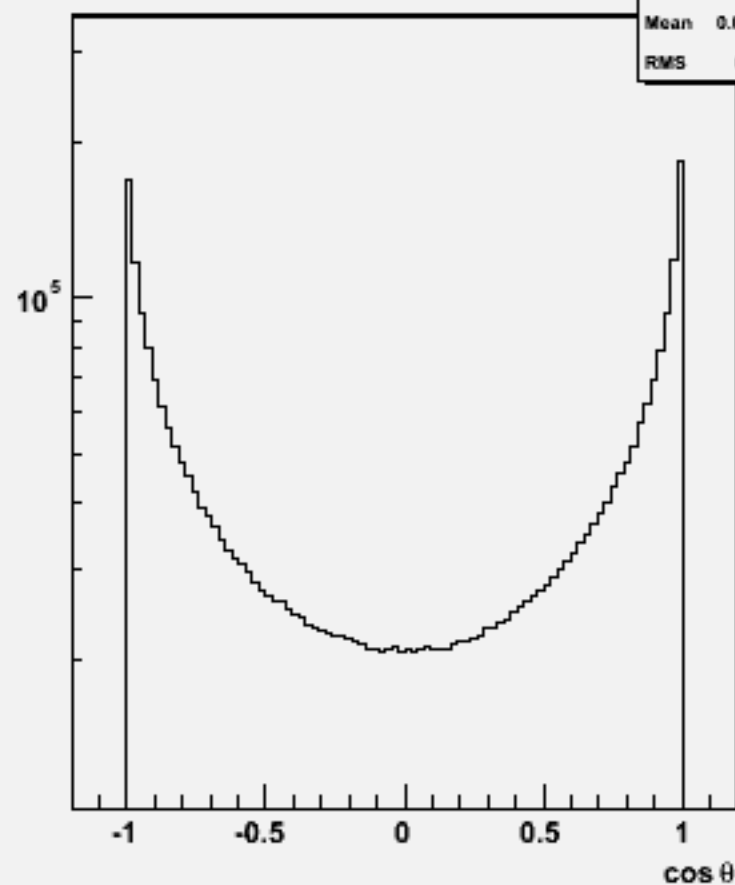
Particle cos \theta : w100596 cce2e2_o
