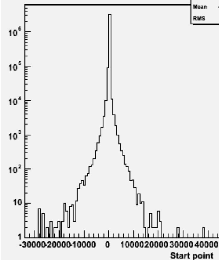
Start point Z : w100596 cce2e2_o
