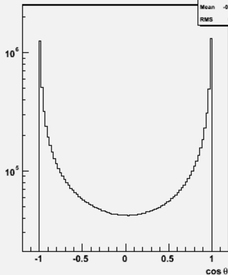
Particle cos \theta : w100594 cce1e1_o
