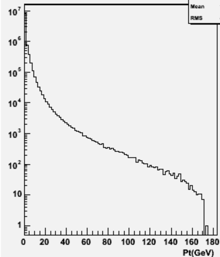
Particle Pt : w100594 cce1e1_o
