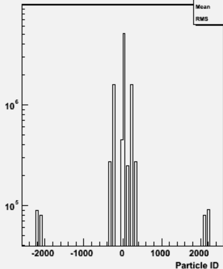
Particle ID : w100594 cce1e1_o
