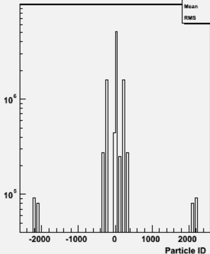
Particle ID : w100593 cce1e1_o
