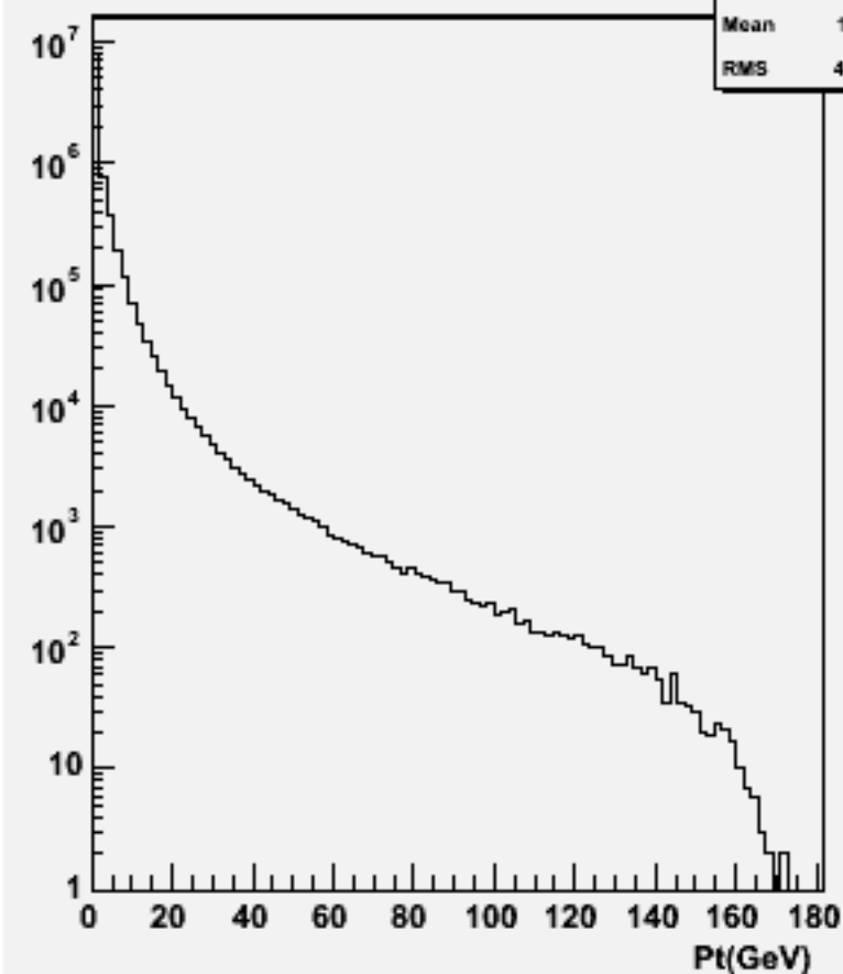
Particle Pt : w100593 cce1e1_o
