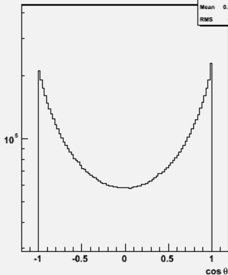
Particle cosθ : w100584 uuss_o
