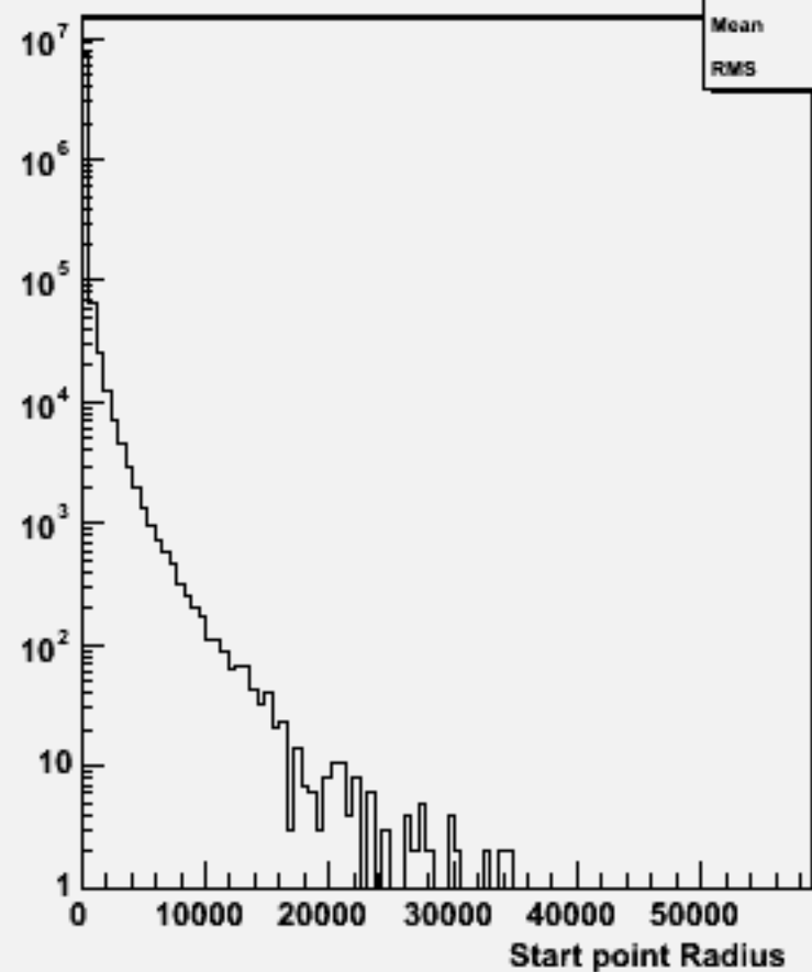
Start point R : w100584 uuss_o
