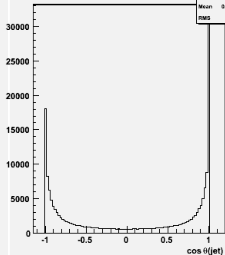
cos \theta for 2-jets :w100584 uuss_o
