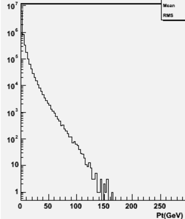
Particle Pt : w100584 uuss_o
