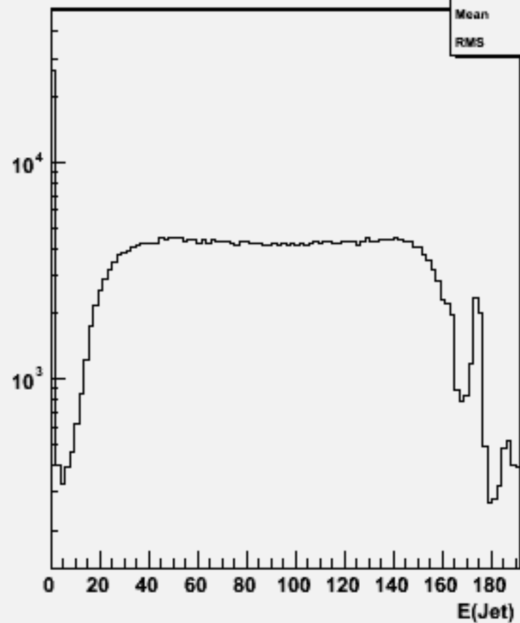
Jet energies(All jets)w100584 uuss_o
