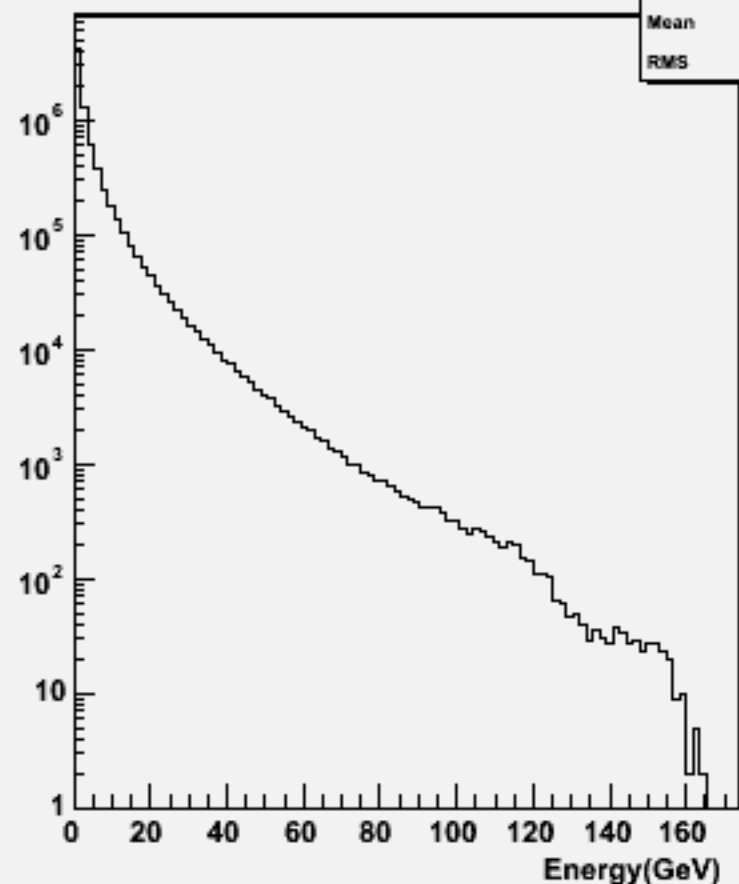
Particle Energy : w100584 uuss_o
