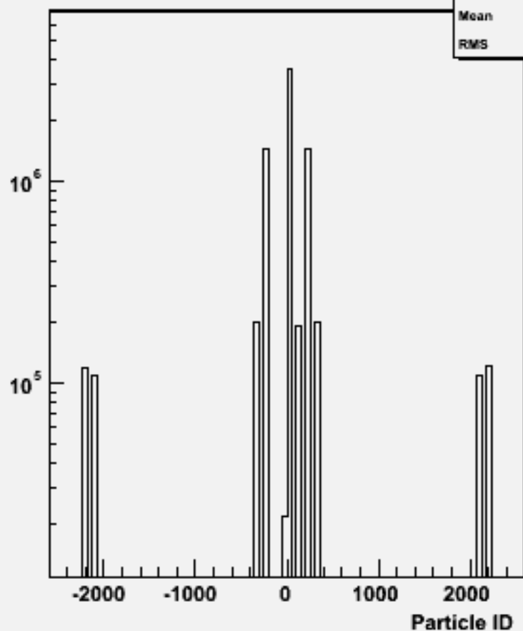
Particle ID : w100584 uuss_o
