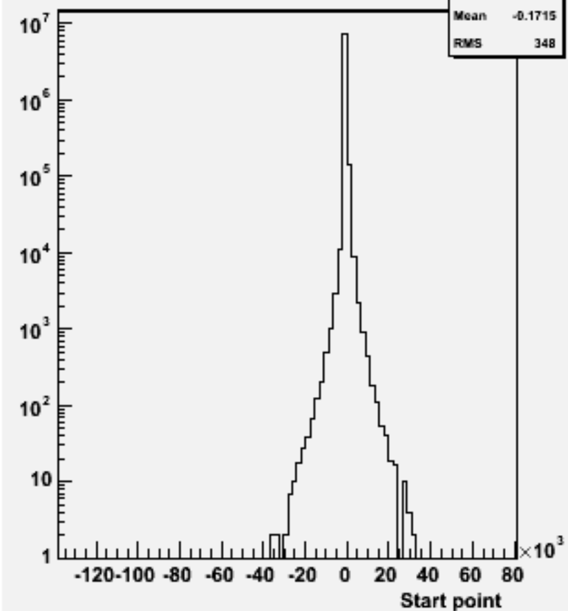
Start point Z : w100584 uuss_o
