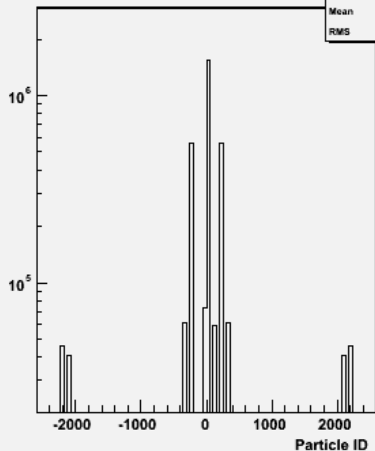
Particle ID : w100576 uue2e2_o
