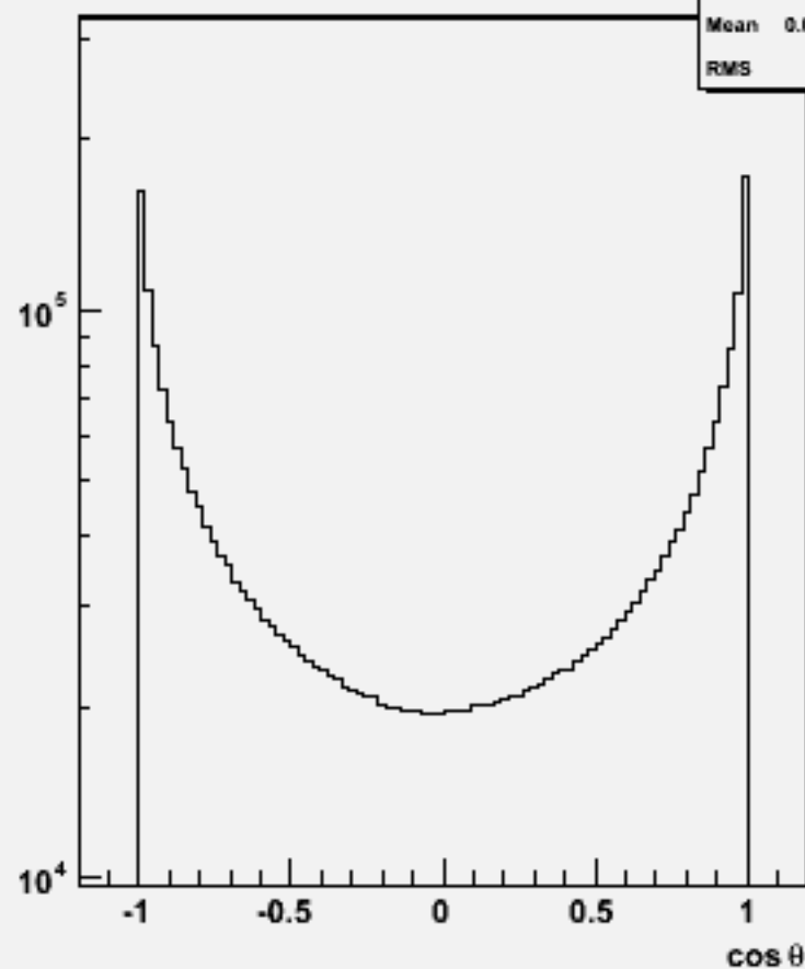
Particle cosθ : w100576 uue2e2_o
