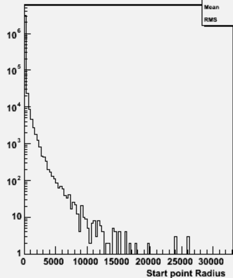
Start point R : w100576 uue2e2_o
