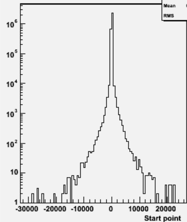
Start point Z : w100576 uue2e2_o
