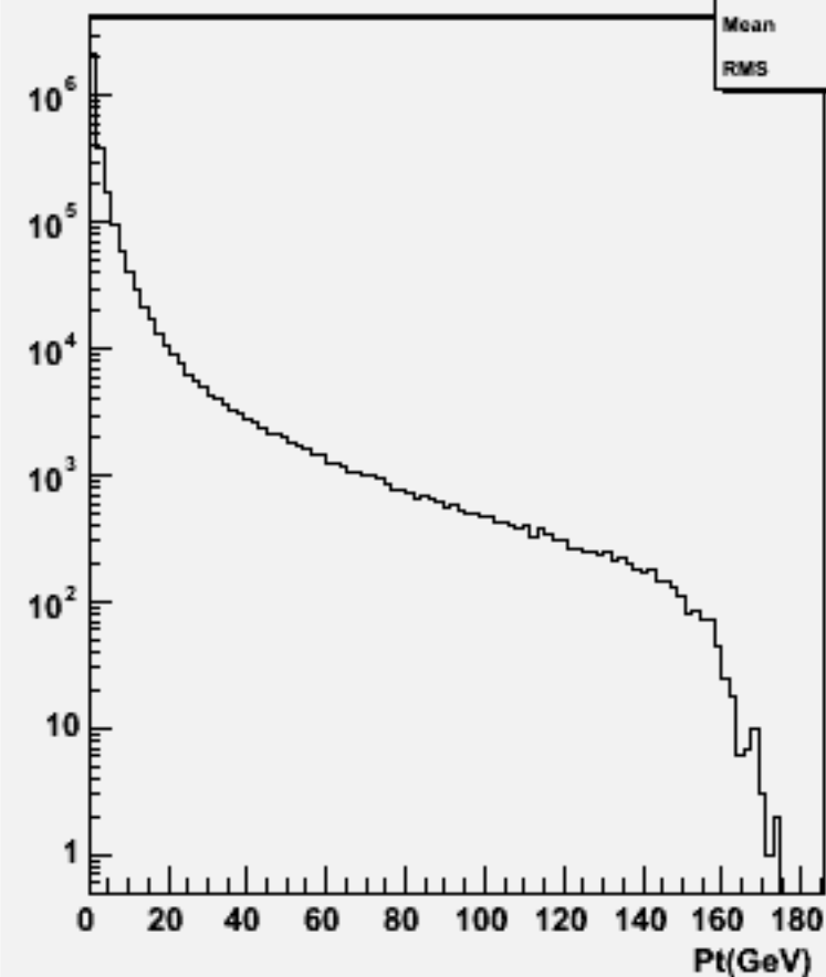
Particle Pt : w100576 uue2e2_o
