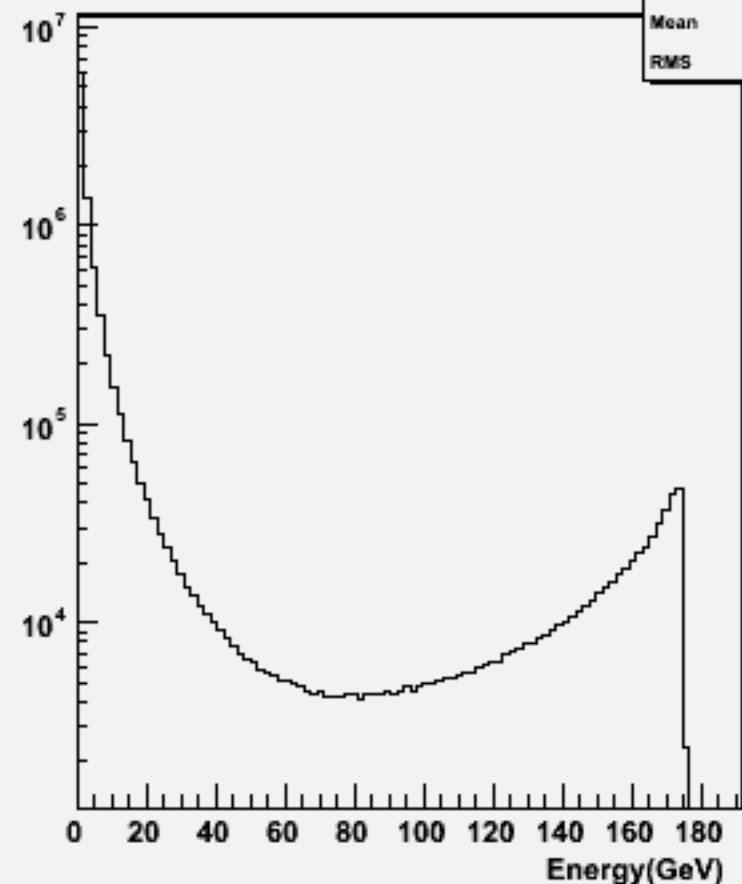
Particle Energy : w100574 uue1e1_o
