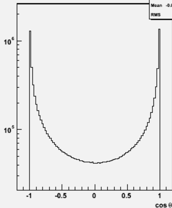
Particle cosθ : w100574 uue1e1_o
