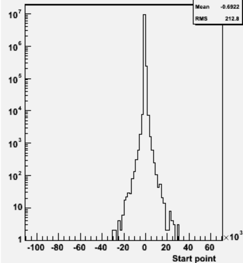
Start point Z : w100574 uue1e1_o
