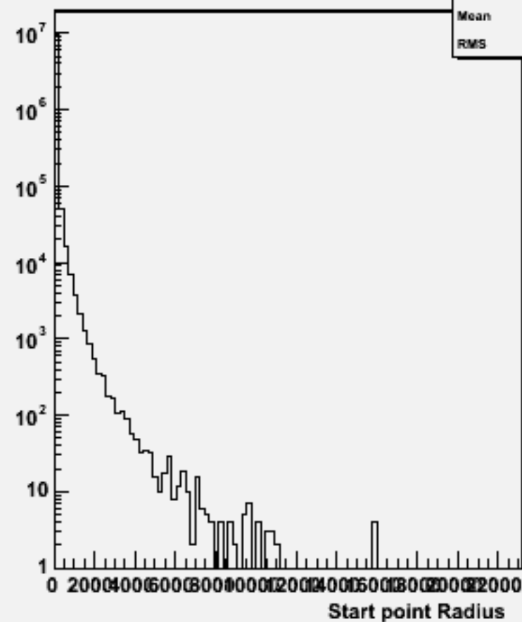
Start point R : w100574 uue1e1_o
