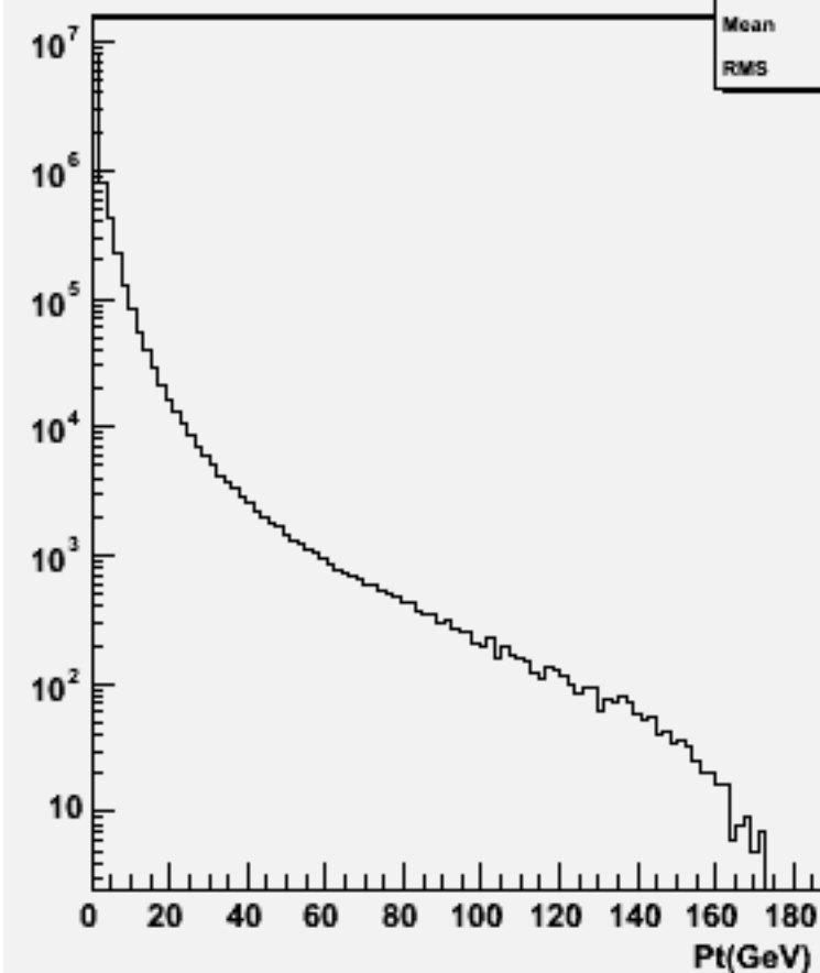
Particle Pt : w100574 uue1e1_o
