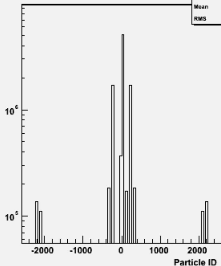
Particle ID : w100574 uue1e1_o
