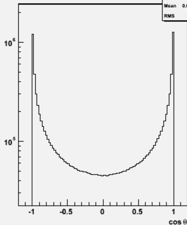
Particle cos \theta : w100572 uue1e1_o
