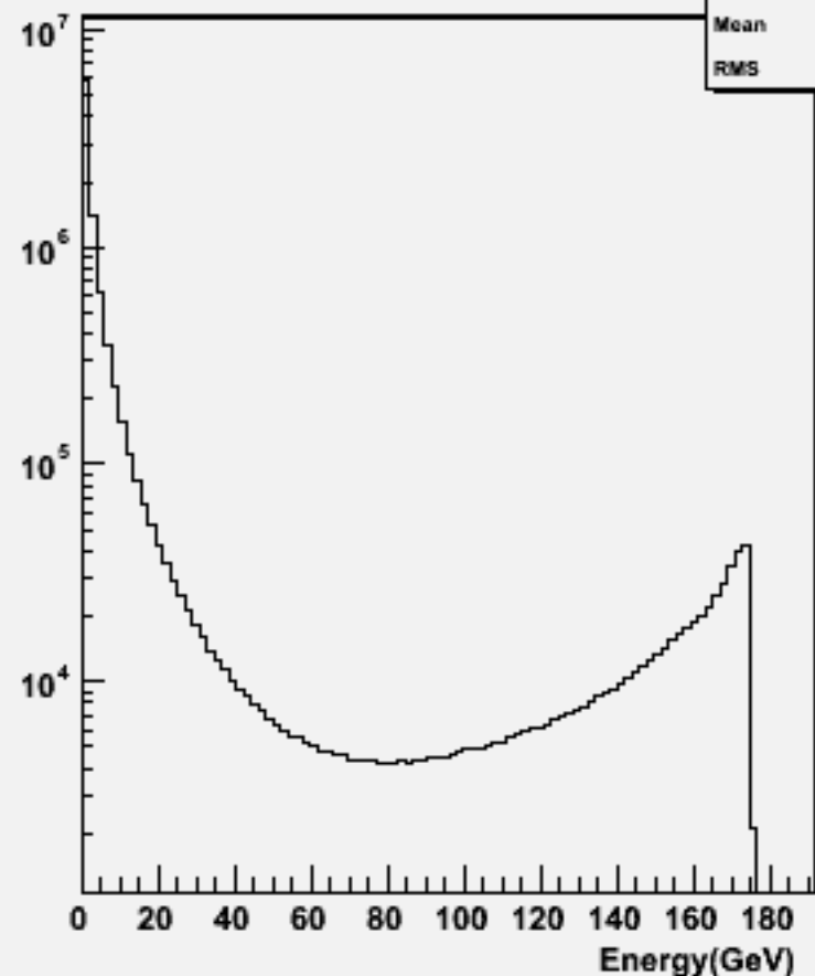
Particle Energy : w100572 uue1e1_o
