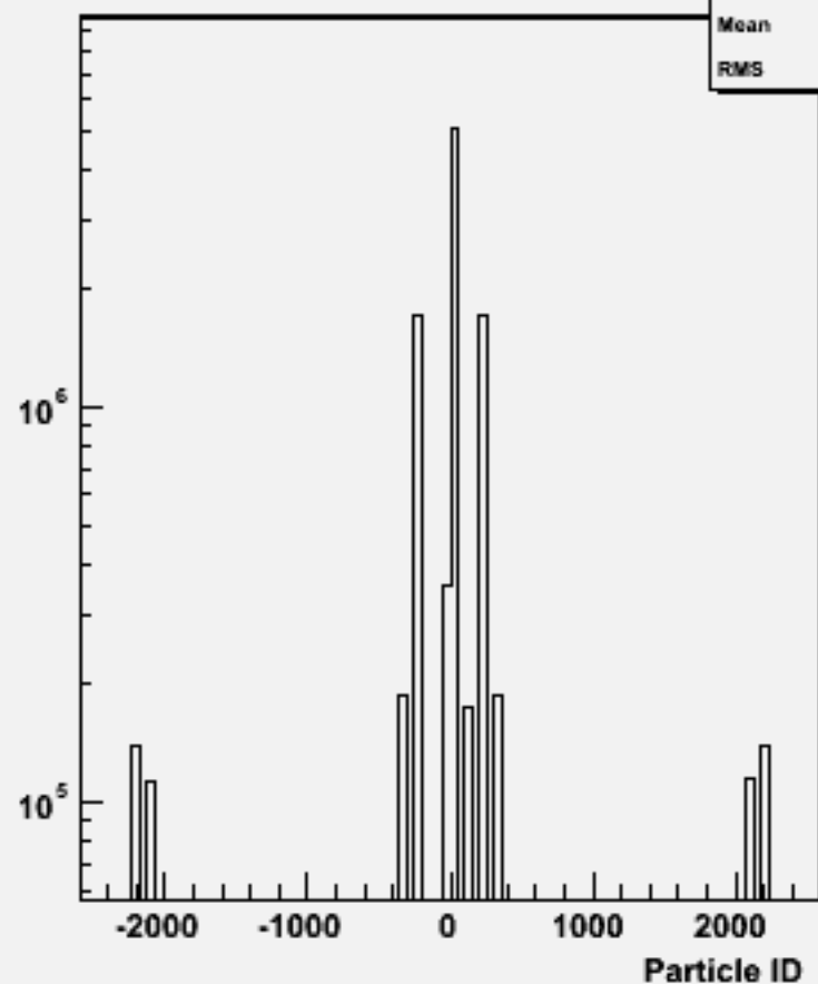
Particle ID : w100572 uue1e1_o
