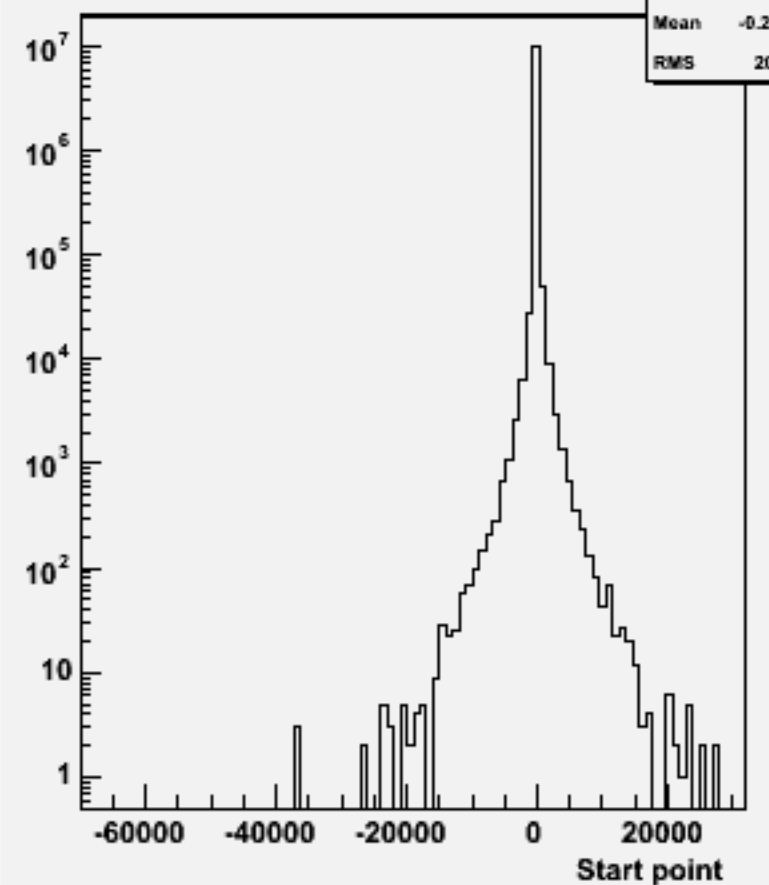
Start point Z : w100572 uue1e1_o
