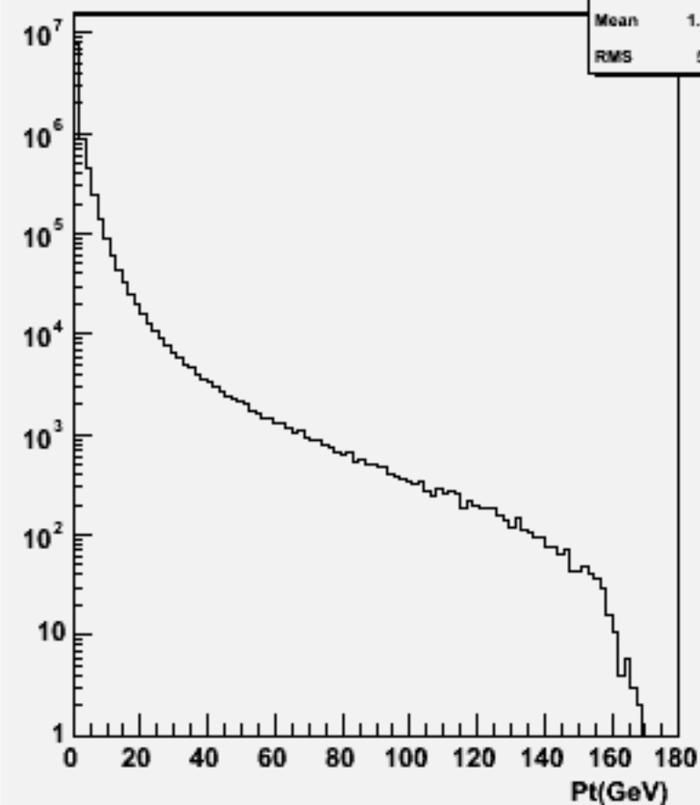
Particle Pt : w100572 uue1e1_o
