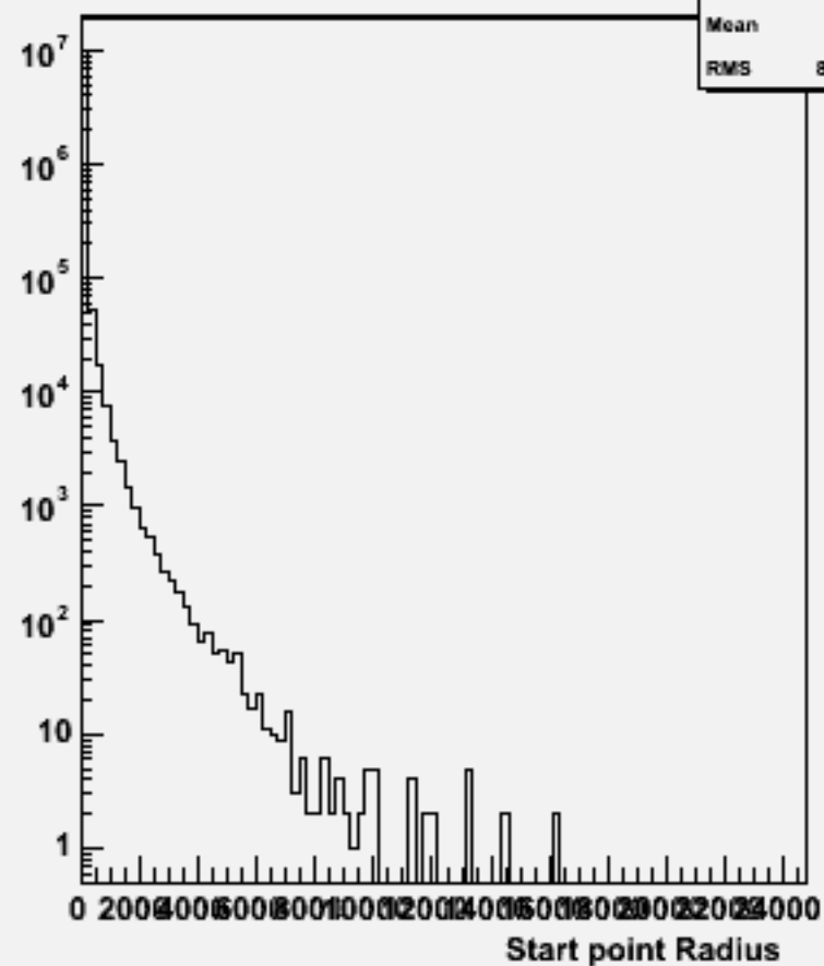
Start point R : w100572 uue1e1_o
