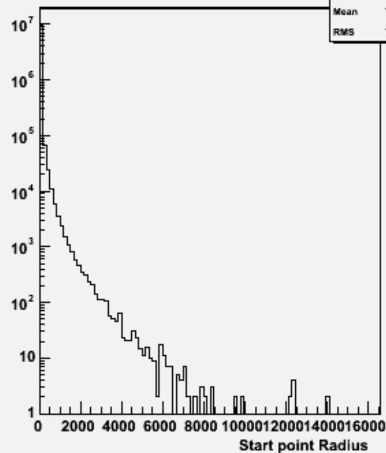
Start point R : w100571 uue1e1_o
