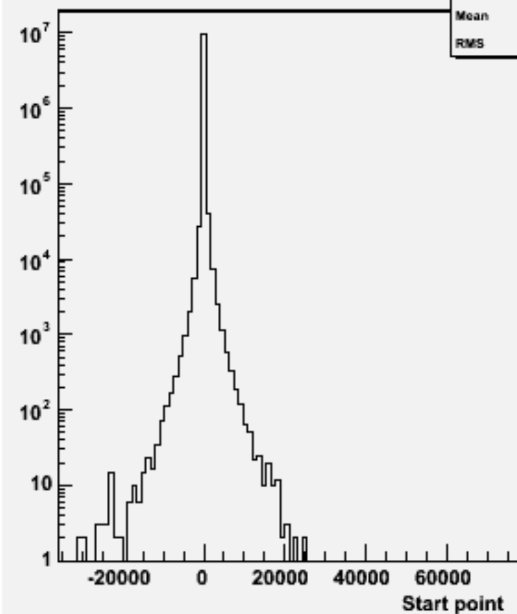
Start point Z : w100571 uue1e1_o
