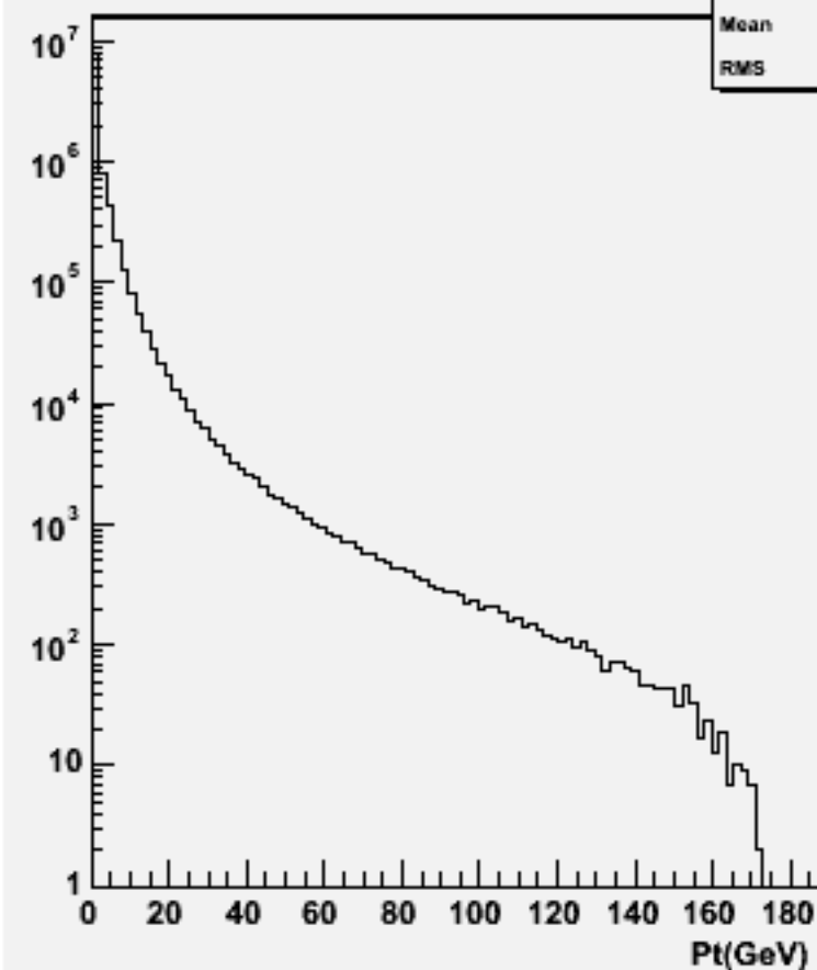
Particle Pt : w100571 uue1e1_o
