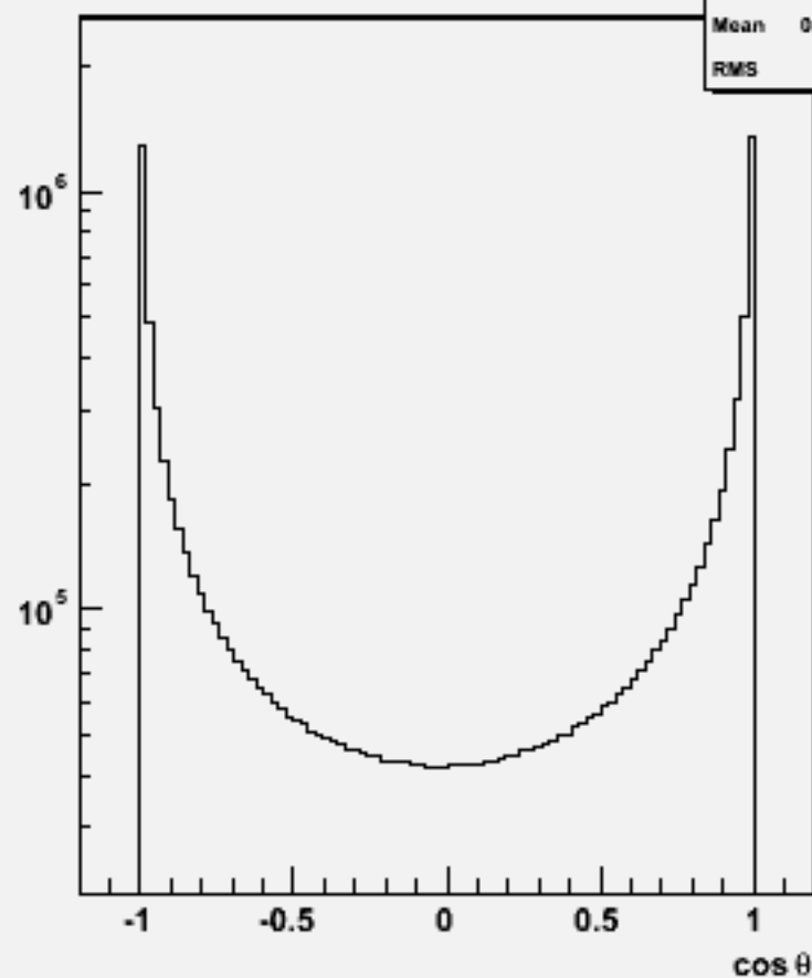
Particle cosθ : w100571 uue1e1_o
