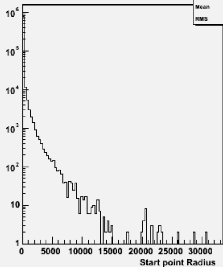
Start point R : w100565 n3n3ss_o
