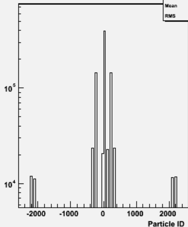
Particle ID : w100565 n3n3ss_o
