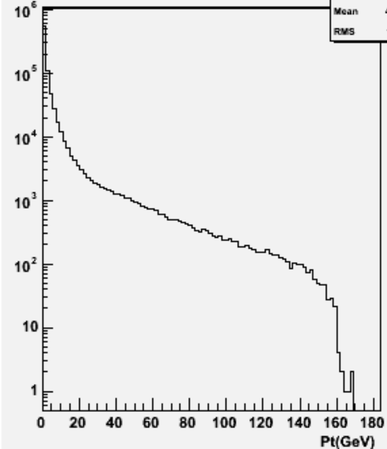
Particle Pt : w100565 n3n3ss_o
