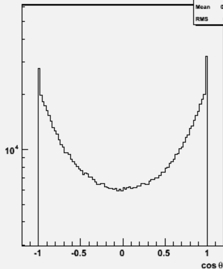
Particle cosθ : w100565 n3n3ss_o
