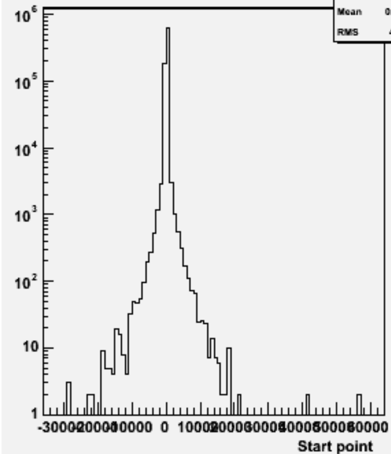
Start point Z : w100565 n3n3ss_o
