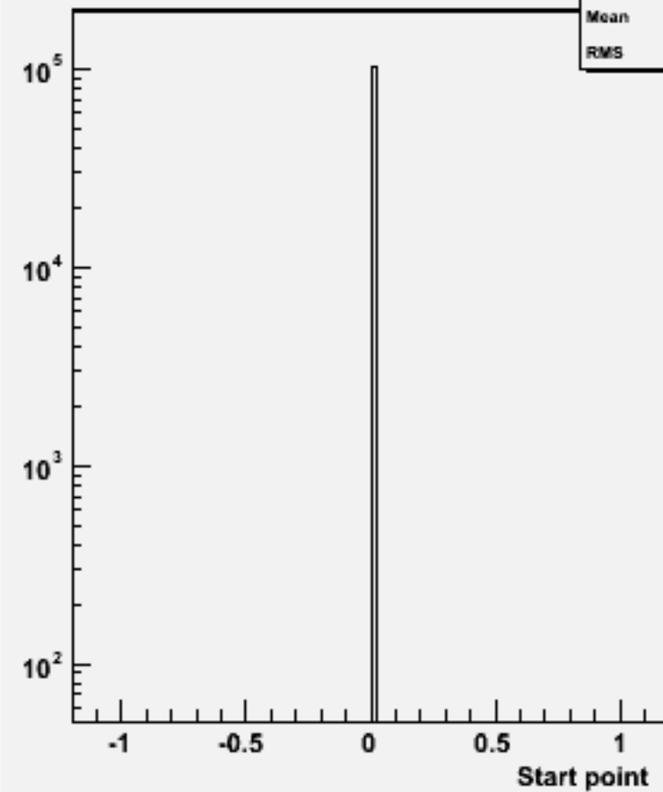
Start point Z : w100557 n3n3e2e2_o
