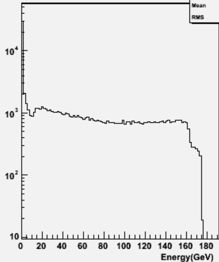
Start point R : w100557 n3n3e2e2_o
