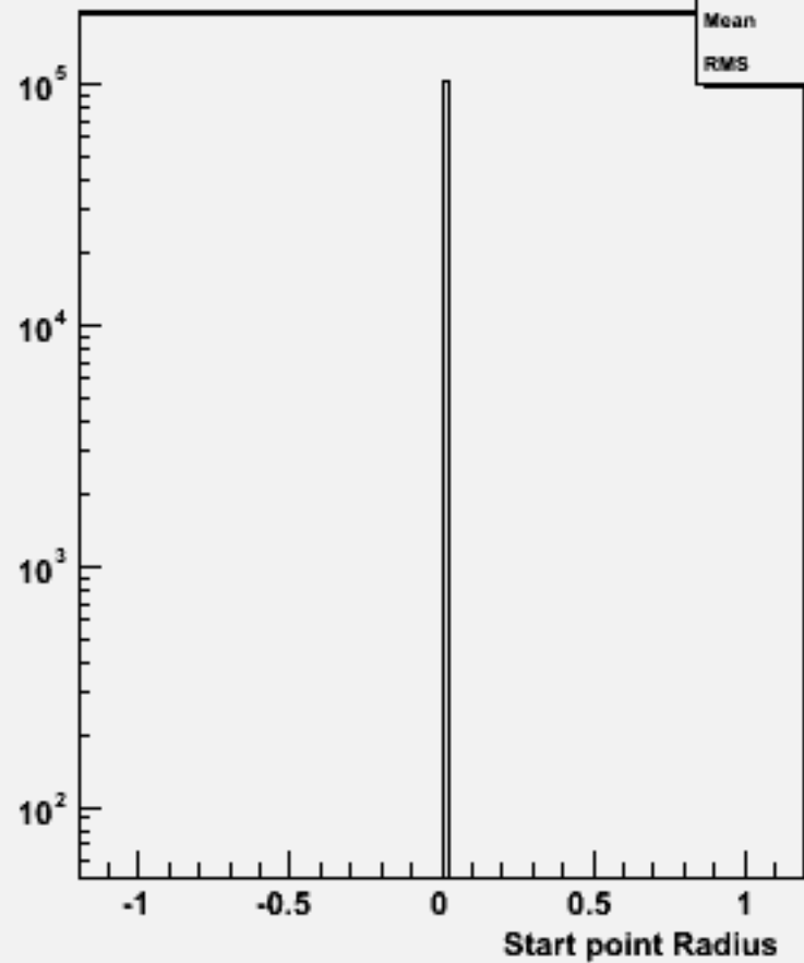
Start point R : w100557 n3n3e2e2_o
