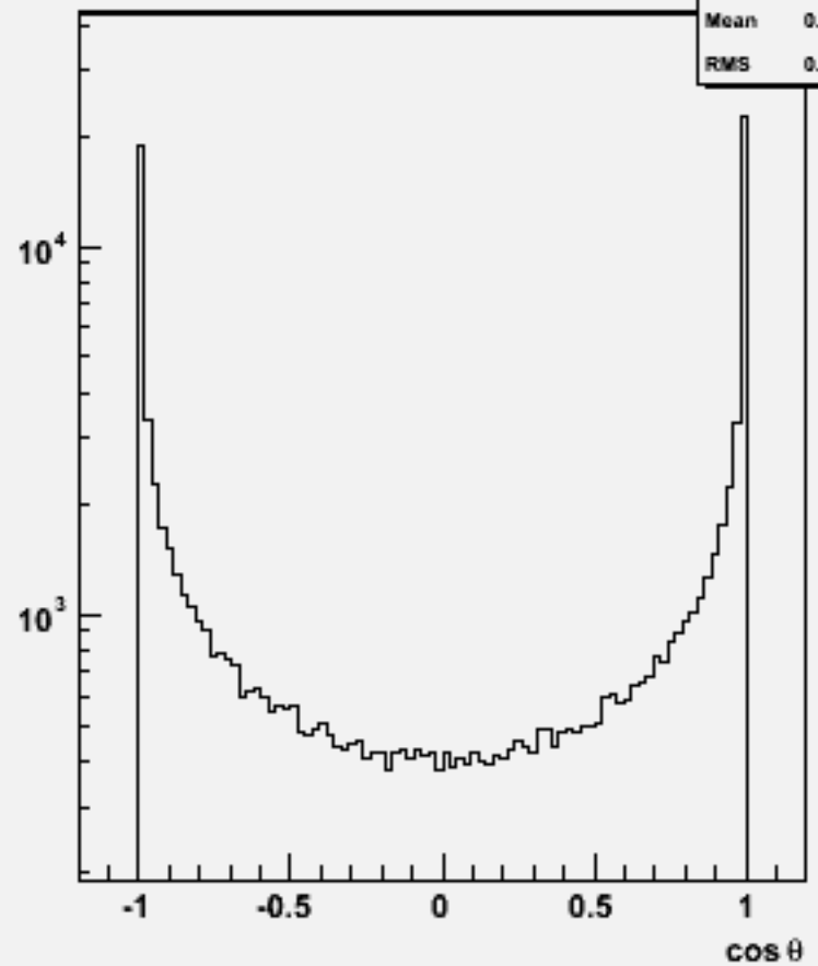
Particle cos \theta : w100557 n3n3e2e2_o
