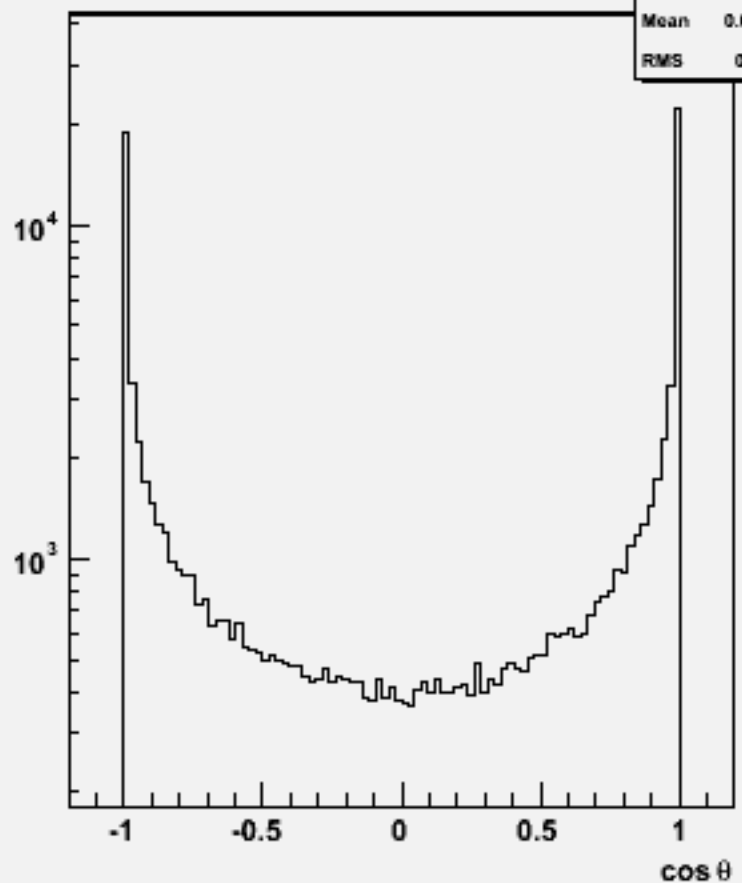
Particle cos \theta : w100513 n1n1e2e2_o
