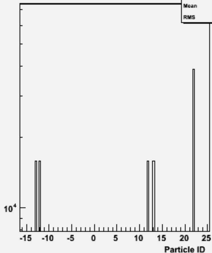
Particle ID : w100513 n1n1e2e2_o
