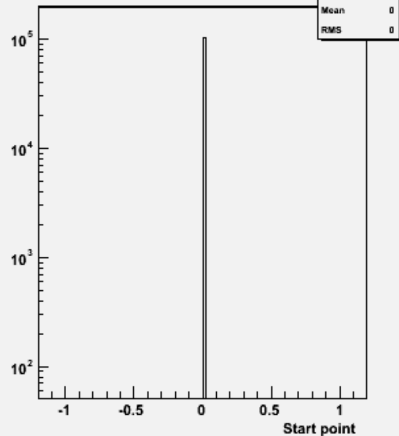
Start point Z : w100513 n1n1e2e2_o
