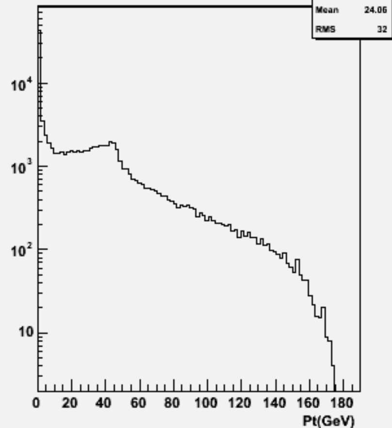
Particle Pt : w100513 n1n1e2e2_o
