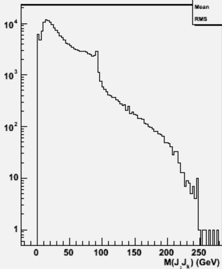
2jets mass(All comb)w100496 n3n3cc_o
