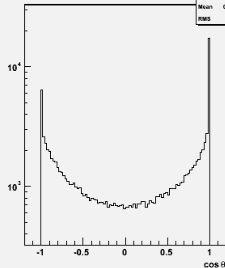
Jet cos \theta (All jets)w100496 n3n3cc_o
