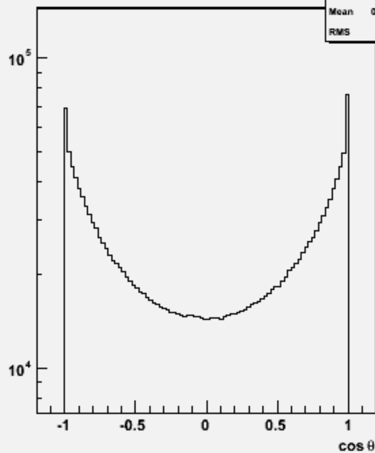
Particle cos \theta : w100496 n3n3cc_o
