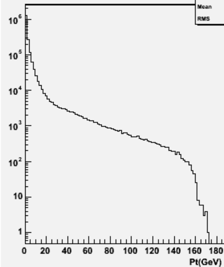
Particle Pt : w100496 n3n3cc_o
