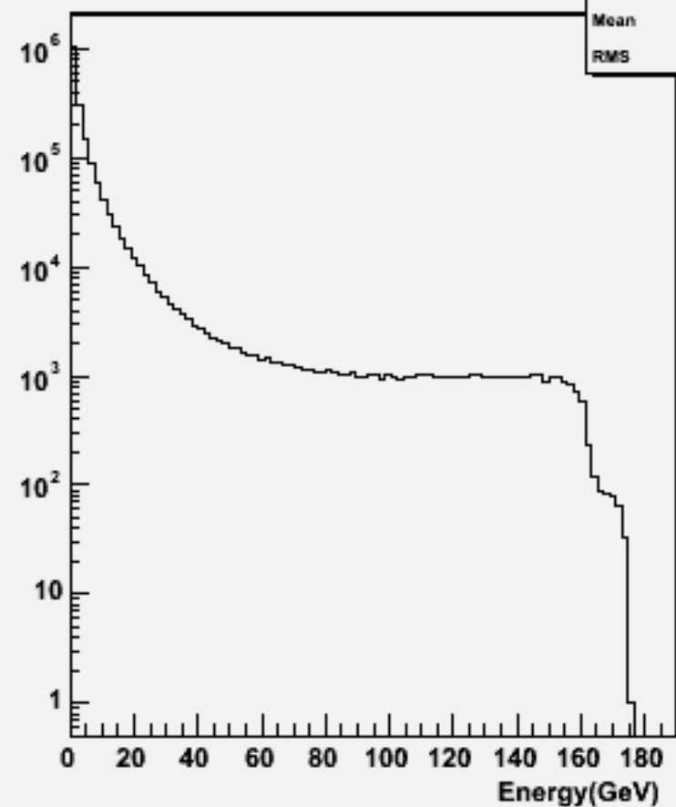
Particle Energy : w100496 n3n3cc_o
