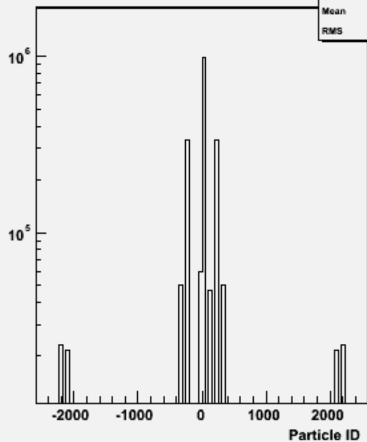
Particle ID : w100496 n3n3cc_o
