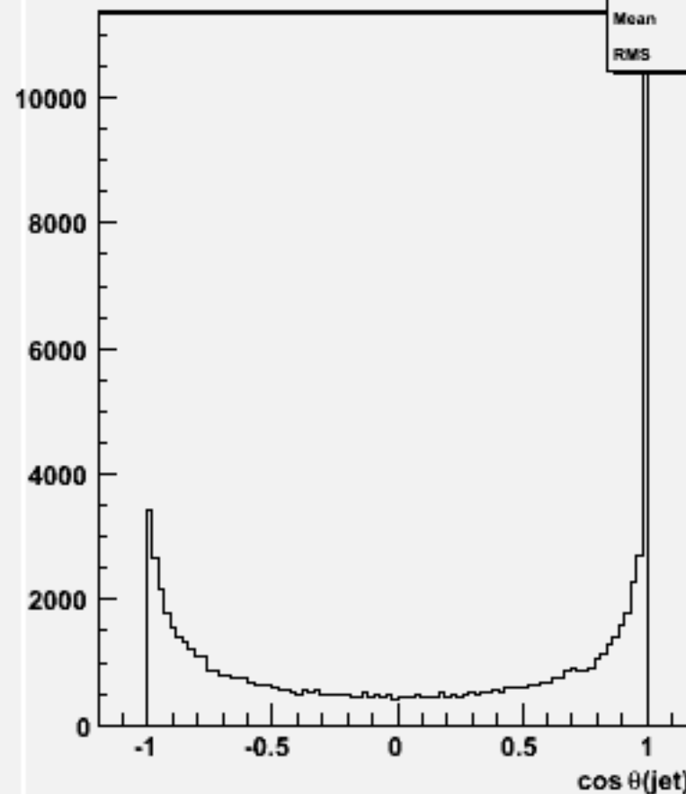
cos \theta for 2-jets :w100496 n3n3cc_o
