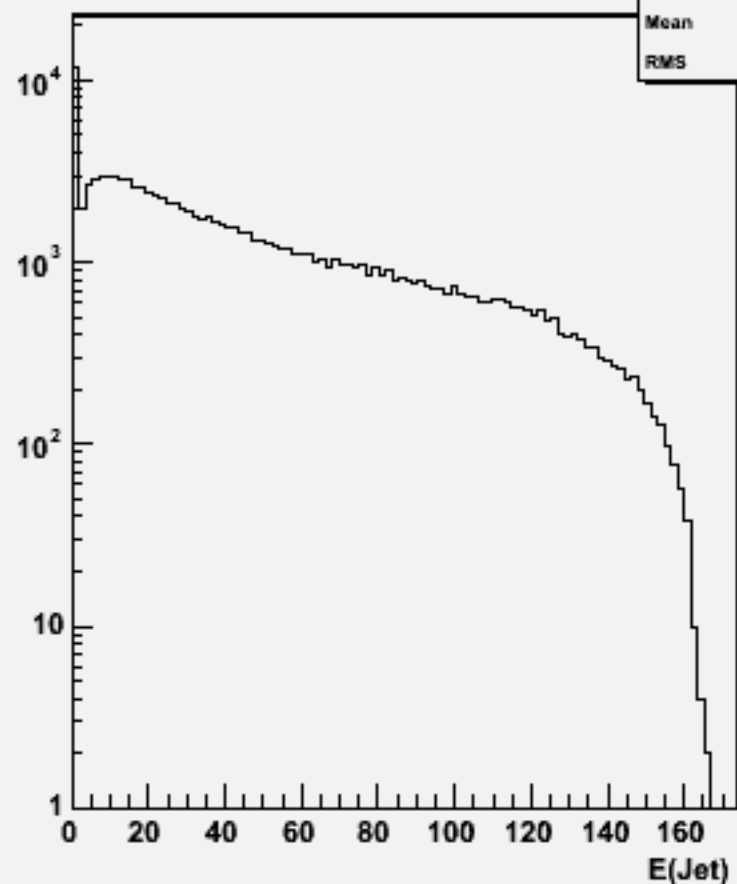
Jet energies(All jets)w100496 n3n3cc_o
