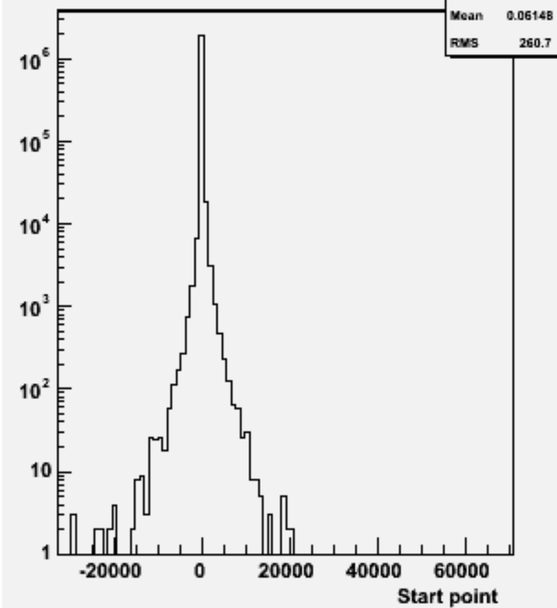
Start point Z : w100496 n3n3cc_o
