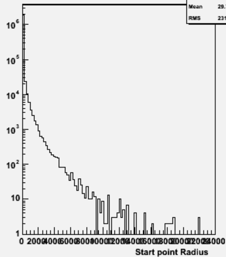
Start point R : w100496 n3n3cc_o
