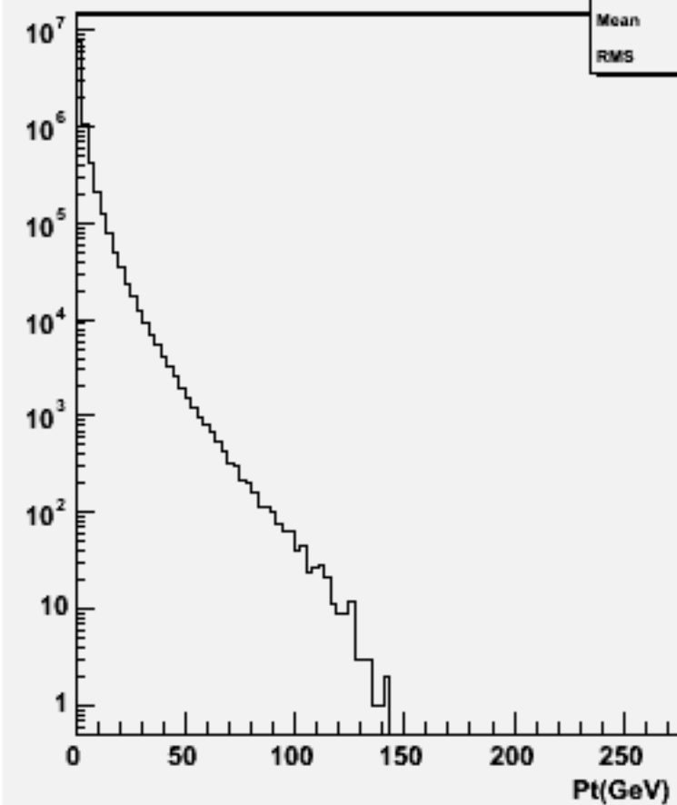
Particle Pt : w100468 csdu_o
