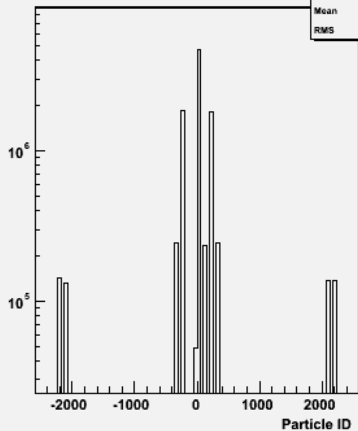
Particle ID : w100468 csdu_o
