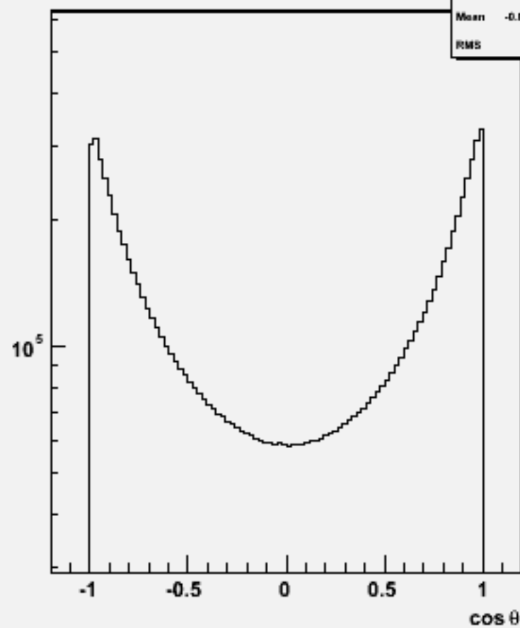
Particle cosθ : w100468 csdu_o
