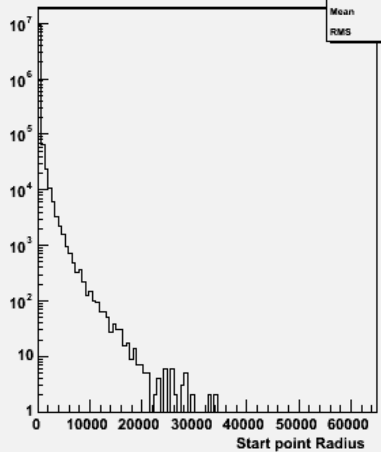
Start point R : w100468 csdu_o
