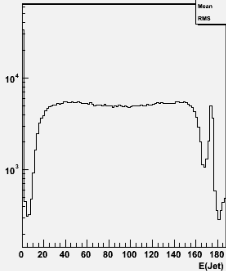
Jet energies(All jets)w100468 csdu_o
