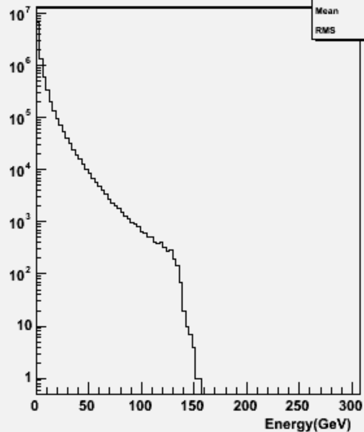
Particle Energy : w100468 csdu_o
