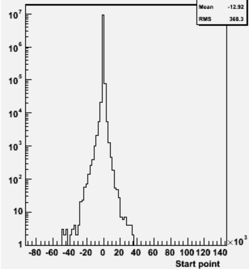
Start point Z : w100468 csdu_o
