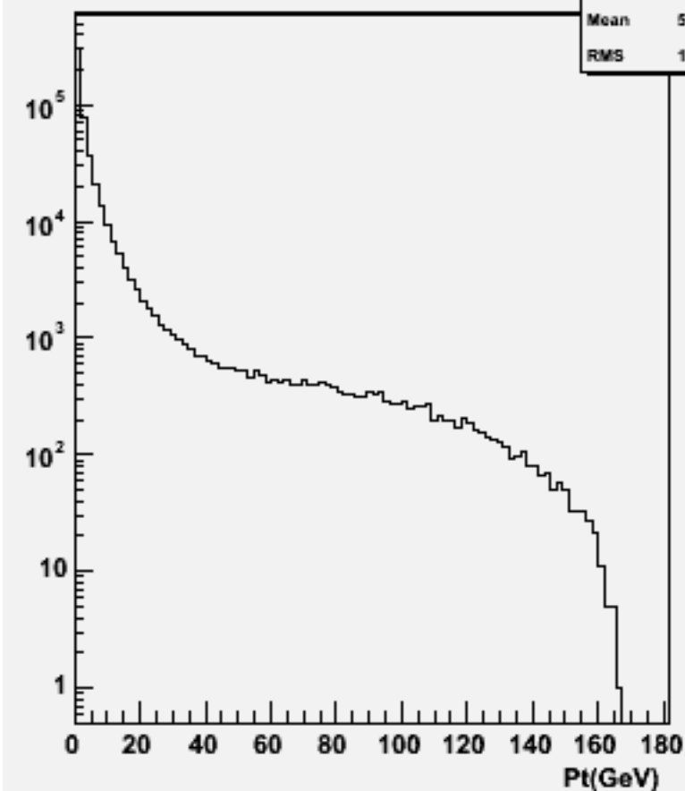
Particle Pt : w100457 cse1n1_o
