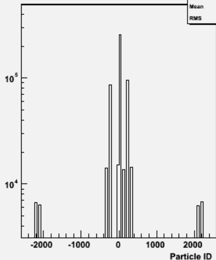
Particle ID : w100457 cse1n1_o
