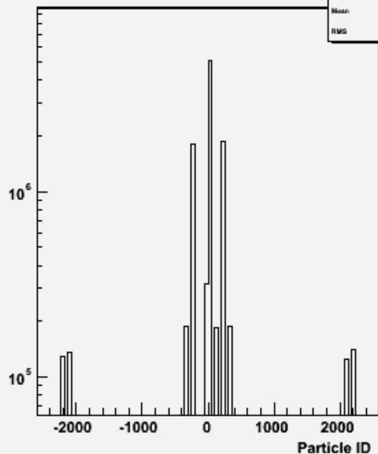
Particle ID : w100444 ude3n3_o
