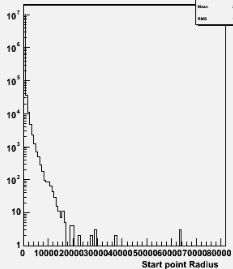
Start point R : w100444 ude3n3_o
