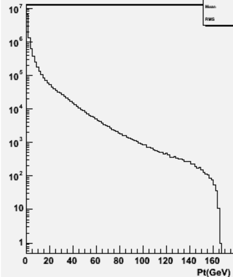
Particle Pt : w100444 ude3n3_o
