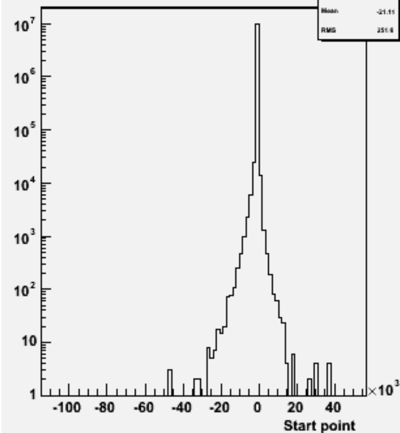
Start point Z : w100444 ude3n3_o
