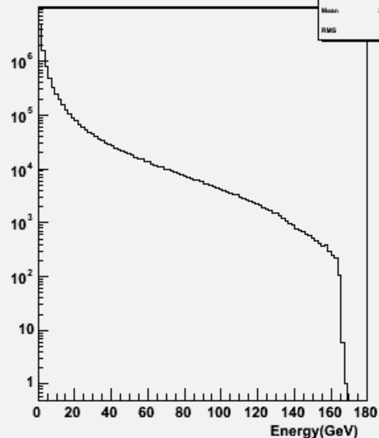
Particle Energy : w100444 ude3n3_o
