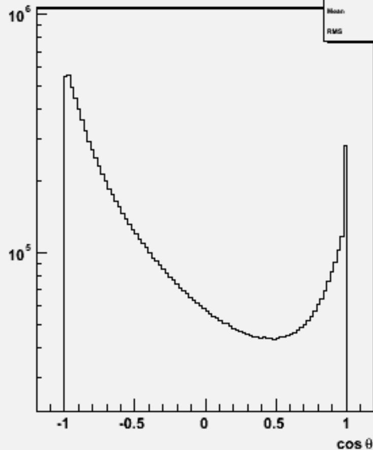
Particle cosθ : w100444 ude3n3_o
