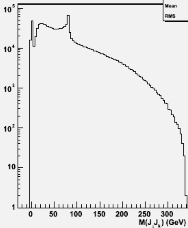
2jets mass(All comb)w100444 ude3n3_o
