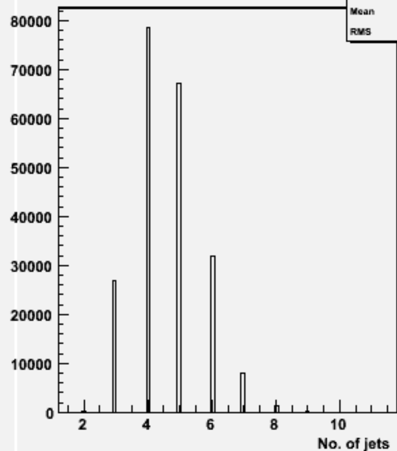
No. jets (ycut=0.001) : w100444 ude3n3_o
