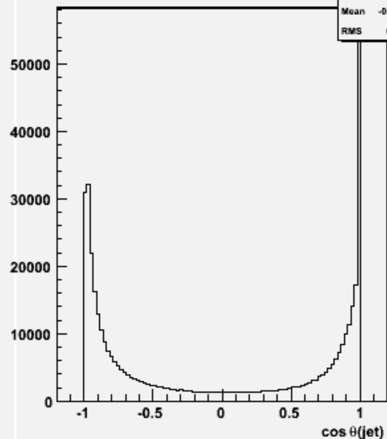
cos \theta for 2-jets :w100444 ude3n3_o
