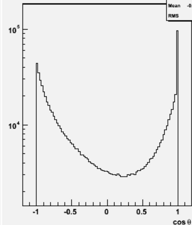
Jet cos \theta (All jets)w100444 ude3n3_o
