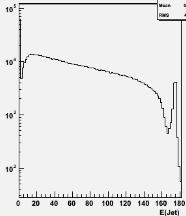
Jet energies(All jets)w100444 ude3n3_o
