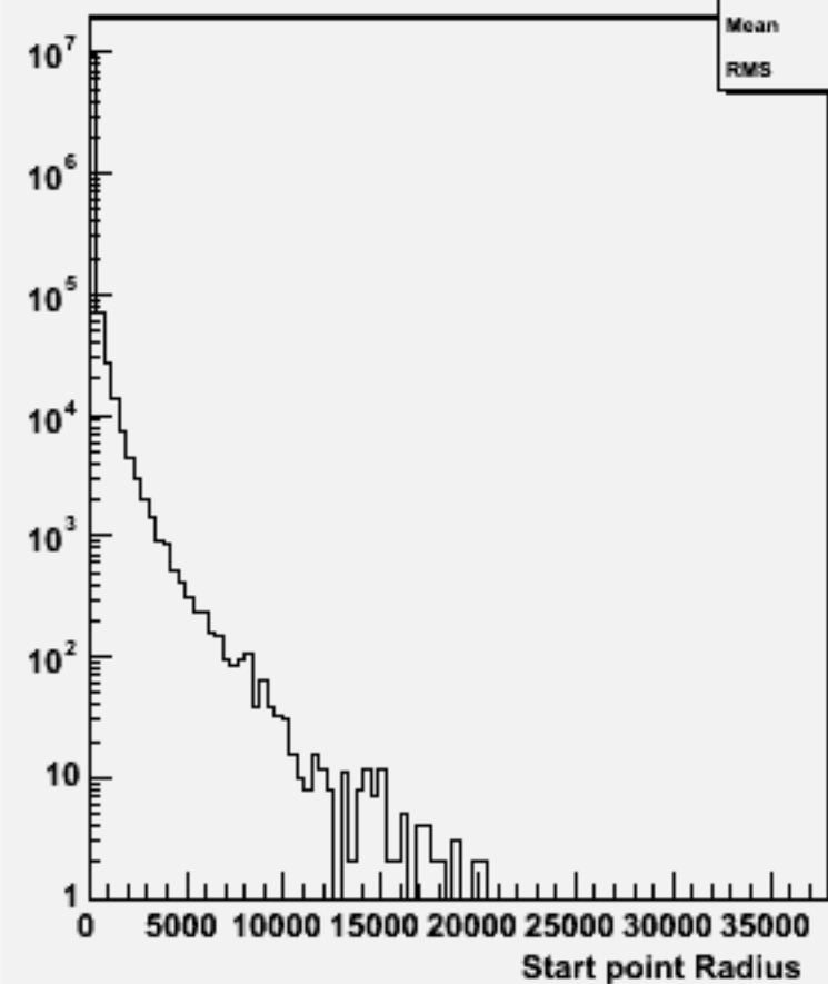
Start point R : w100436 ude1n1_o
