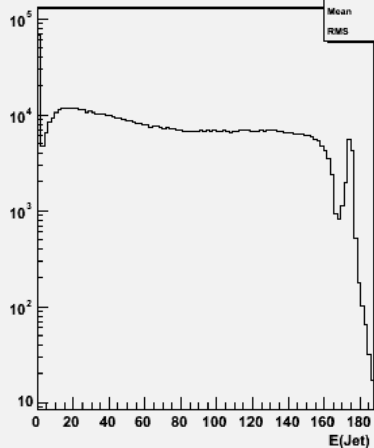
Jet energies(All jets)w100436 ude1n1_o
