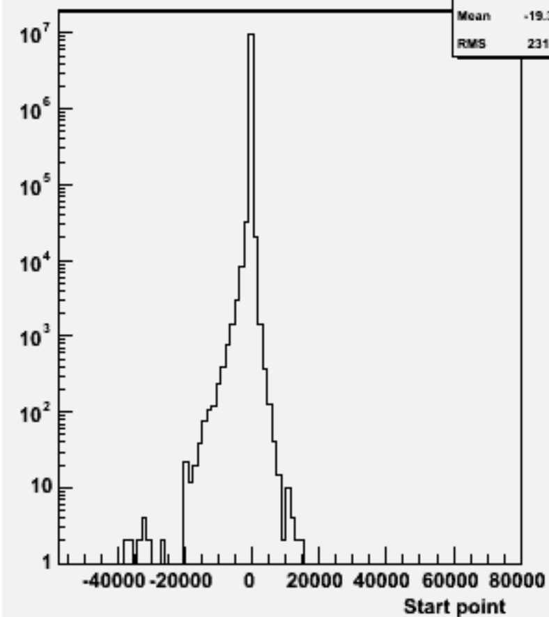
Start point Z : w100436 ude1n1_o
