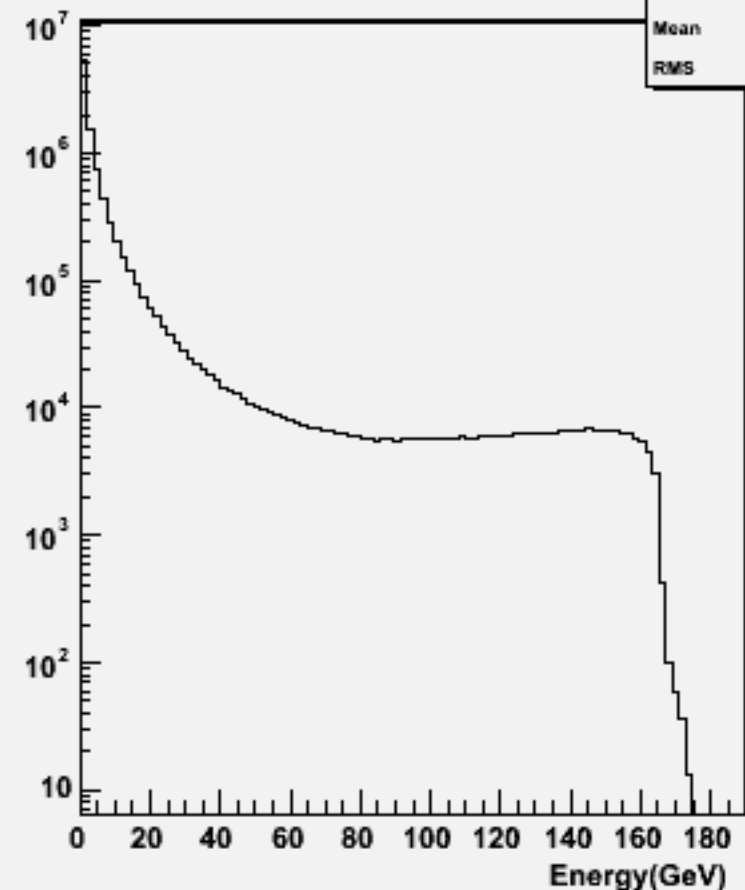
Particle Energy : w100436 ude1n1_o
