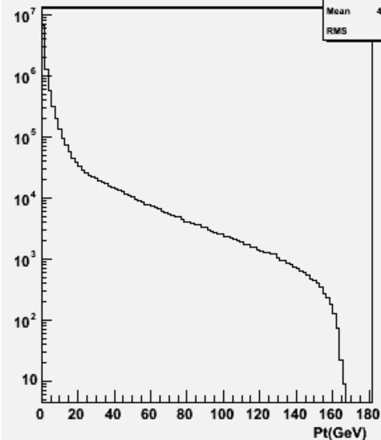
Start point Z : w100436 ude1n1_o
