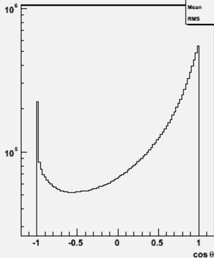
Particle cos \theta : w100392 n1e1sc_o
