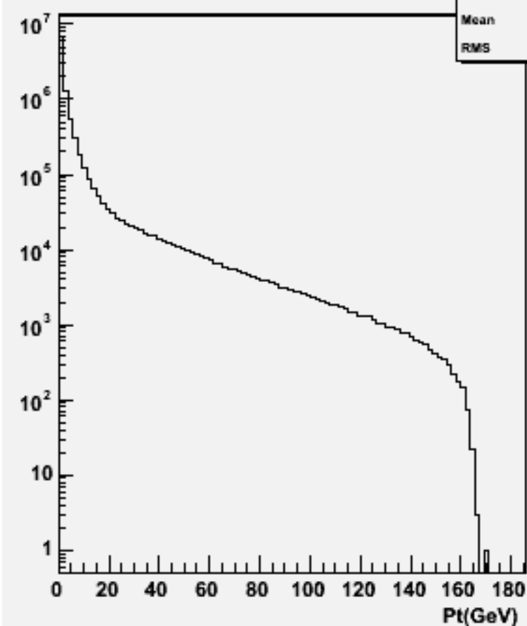
Particle Pt : w100392 n1e1sc_o
