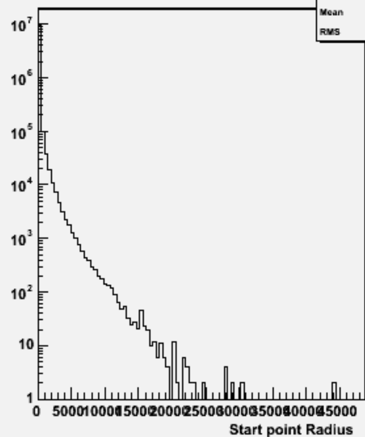
Start point R : w100392 n1e1sc_o
