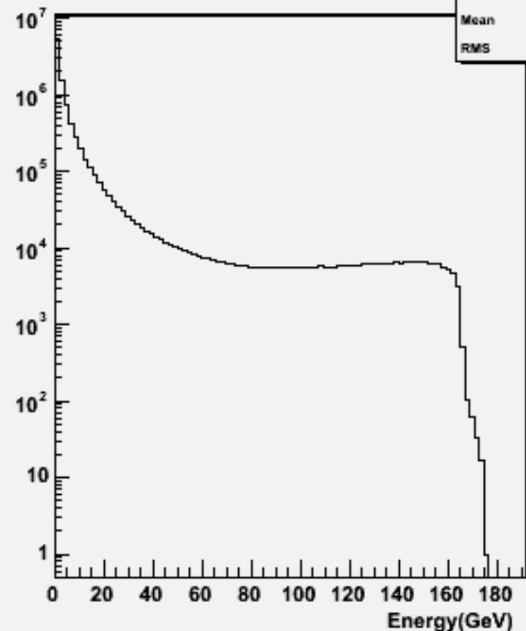
Particle Energy : w100392 n1e1sc_o
