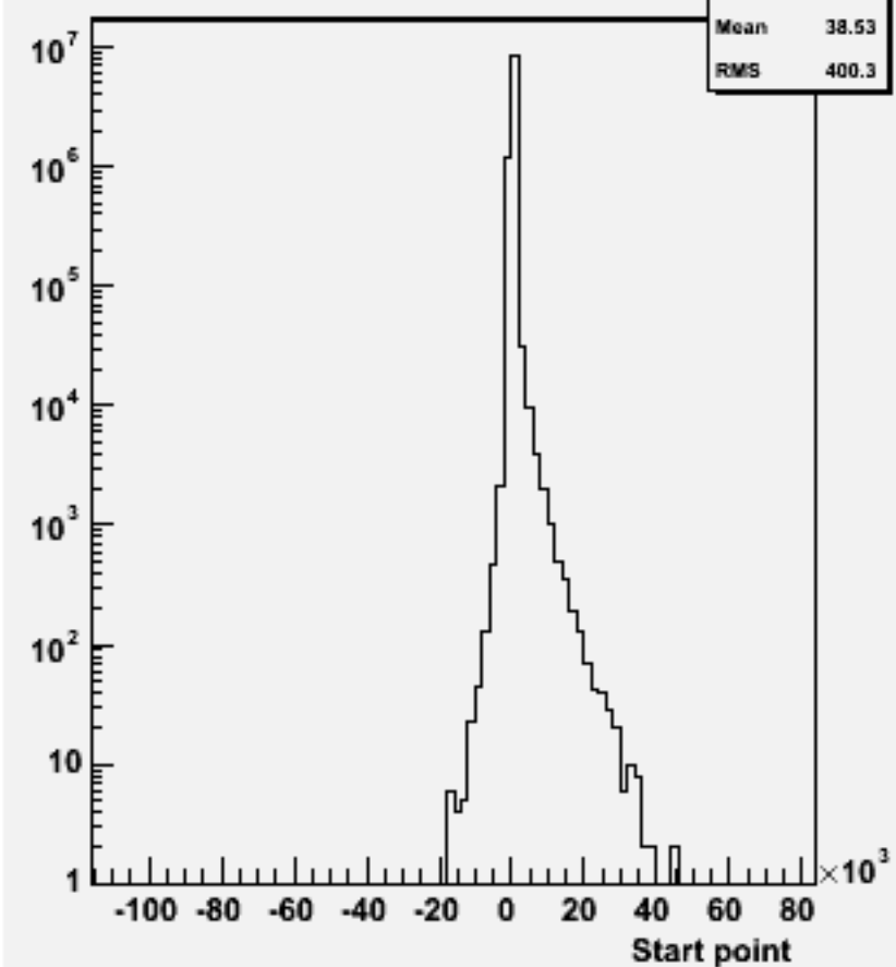
Start point Z : w100392 n1e1sc_o
