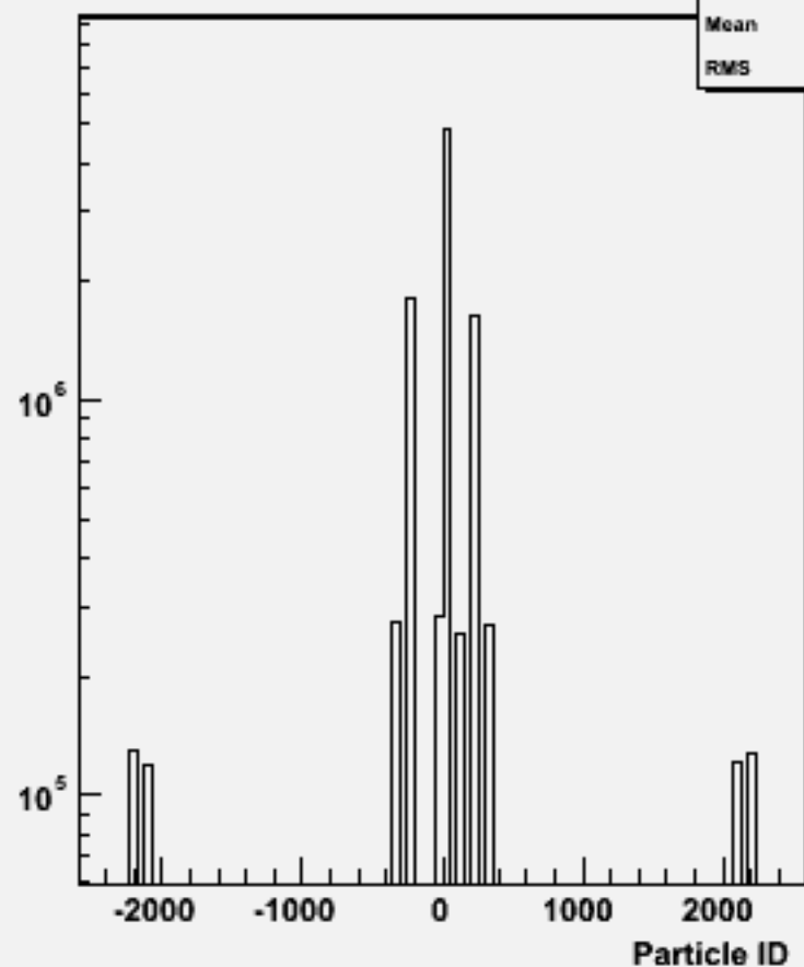
Particle ID : w100392 n1e1sc_o
